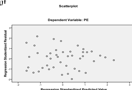
Gambar 2 Uji Heteroskedastisitas
