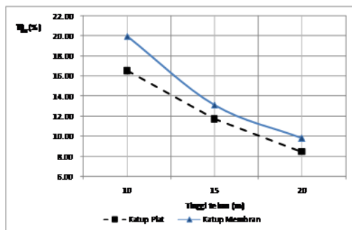
Gambar 11. Grafik efisiensi volumetris pompa hidram
