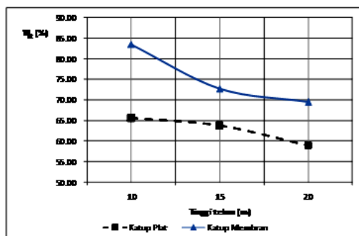
Gambar 12. Grafik efisiensi total pompa hidram
