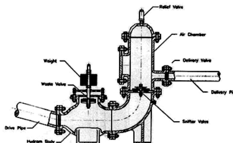
Gambar 3. Komponen – komponen utama pompa hydram. (sumber : Tessema, 2000, hal 3)
