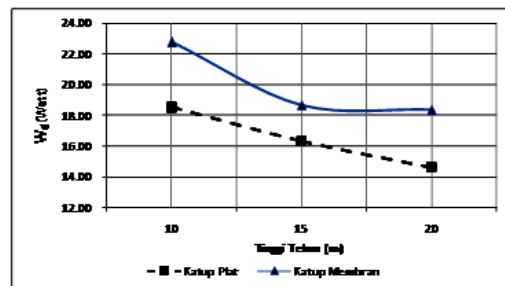
Gambar 10. Grafik Daya output pompa hidram
