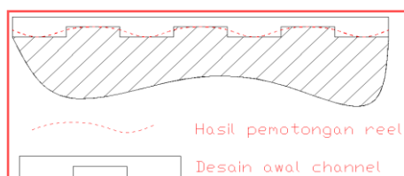
Gambar 8. Hasil Perbandingan antara desain channel dengan hasil akhir permukaan setelah proses pemotongan
