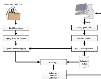
Gambar 3. Alur proses dari metode Latent Semantic Indexing
