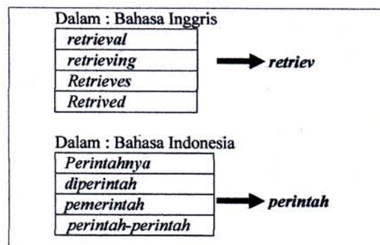
Gambar 3. Stemming dalam Bahasa Inggris dan Indonesia
