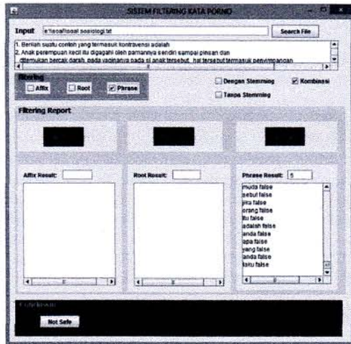
Gambar 12. Pengujian pada kata frase ( Phrase Filtering )
