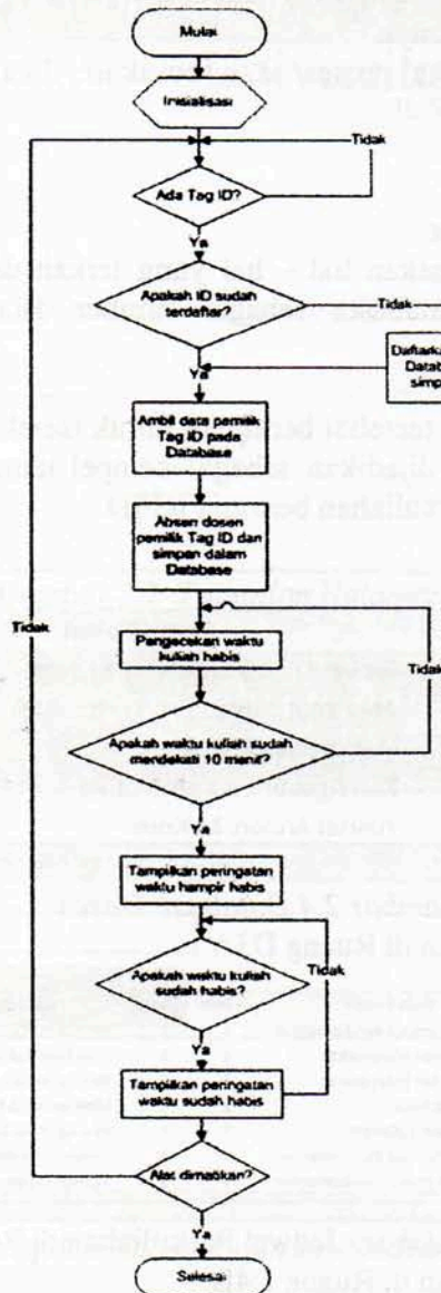
Gambar 2.3 Flowchart sistem validasi dan pencatatan kehadiran Dosen
