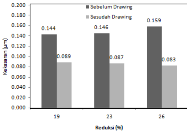
Gambar 5. Grafik hasil pengujian kekasaran
