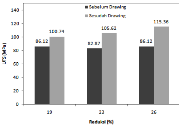
Gambar 2. Grafik kekuatan tarik hasil pengujian tarik
