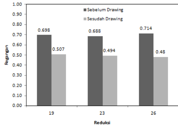
Gambar 3. Grafik regangan hasil pengujian tarik
