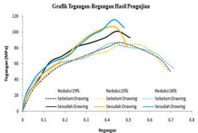
Gambar 4 Grafik tegangan regangan hasil pengujian
