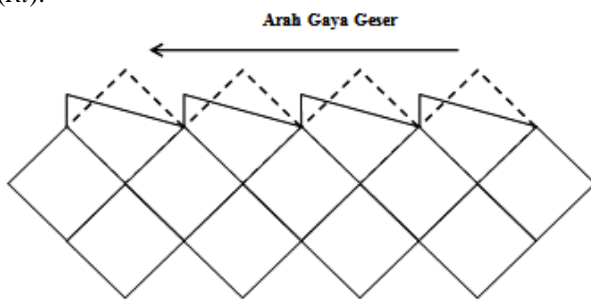
Gambar 7. Deformasi permukaan akibat proses drawing
