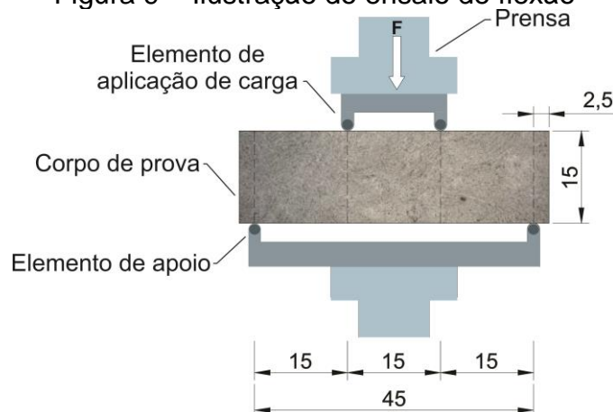
Figura 9 – Ilustração do ensaio de flexão
