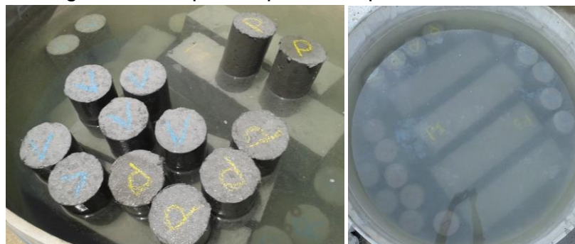
Figura 5 – Corpos de prova em processo de cura
