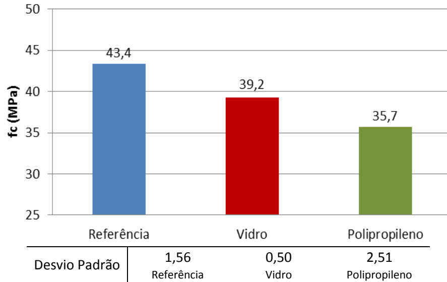
Figura 13 – Resultados de resistência à compressão axial
