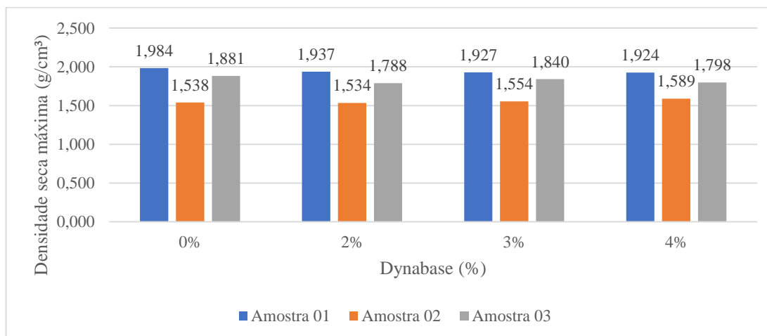
Figura 6. Densidade seca máxima
