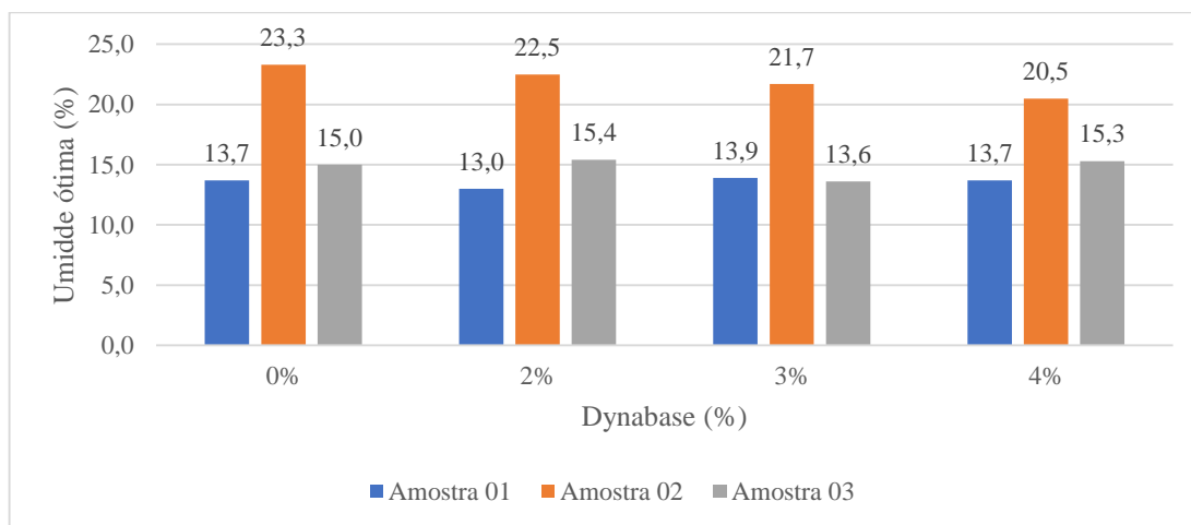
Figura 5. Umidade ótima de compactação
