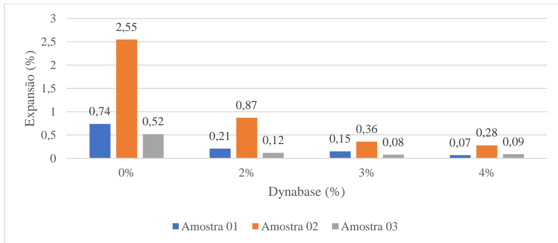
Figura 7. Expansão volumétrica
