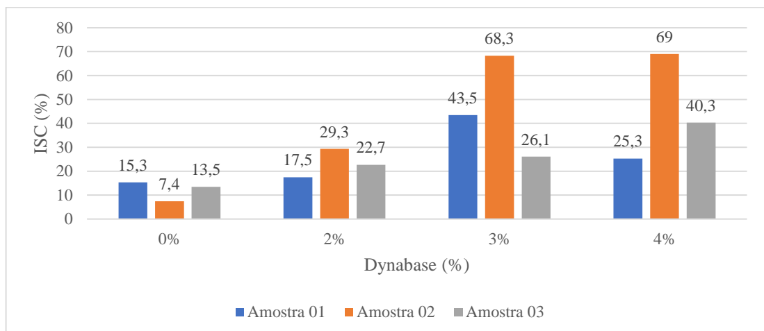
Figura 8. Índice de Suporte Califórnia
