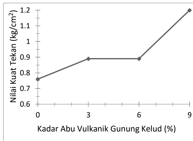
Gambar 1 Grafik peningkatan nilai kuat tekan bebas
