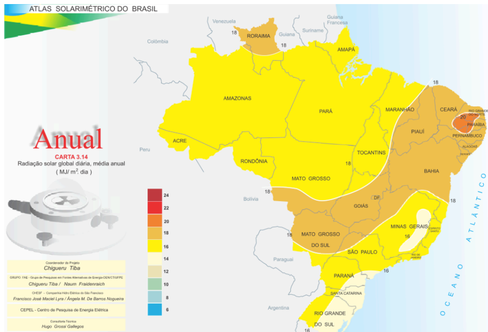
Figura 7. Radiação Solar Global Diária média anual diária (MJ/m 2 /dia) no Brasil. Fonte: Grupo FAE, 2000.
