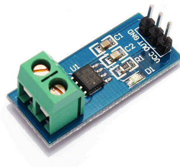
Figura 101. Sensor de corrente ACS712. Fonte: FilipeFlop.com
