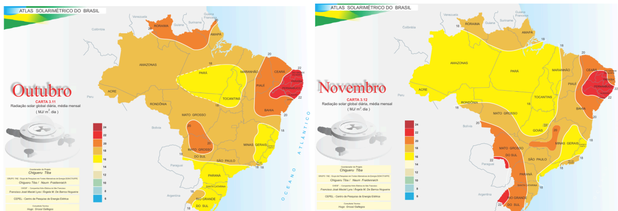
Figura 8. Radiação solar global diária média mensal (MJ/m 2 /dia) no Brasil. Fonte: Grupo FAE, 2000
