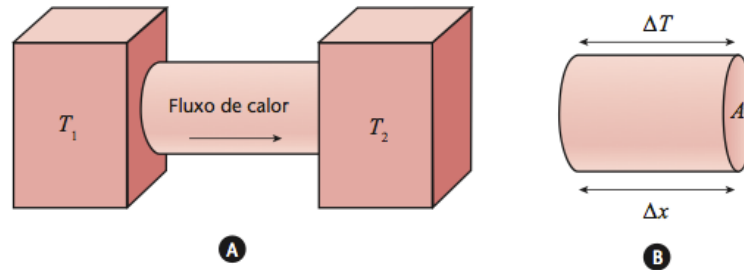
Figura 17. a) Esquema de uma barra condutora ligada com dois reservatórios térmicos com temperaturas diferentes ( T_1 > T_2 ). b) Detalhe do segmento de barra condutora. Fonte: (CRUZ, 2014)
