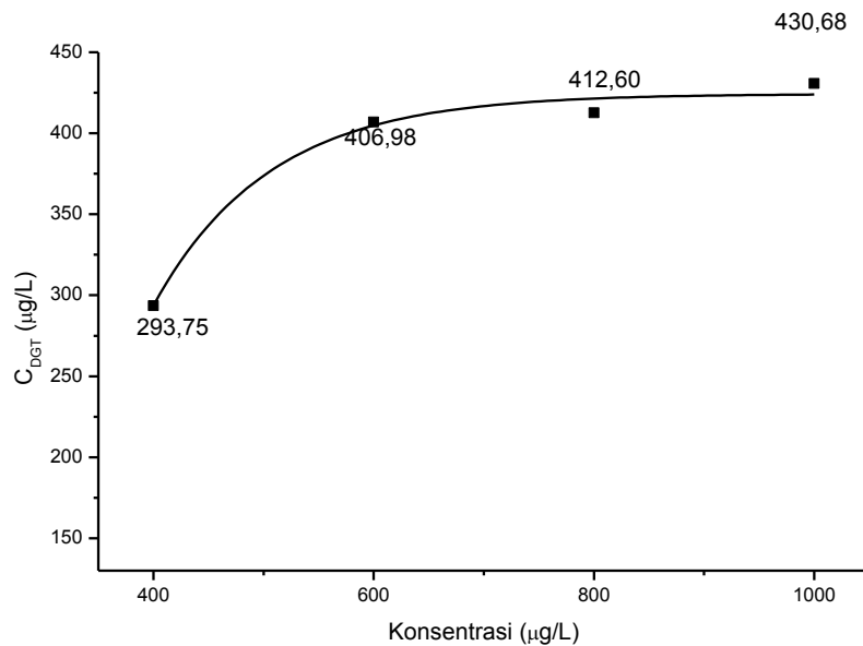
Gambar 5. Pengaruh Konsentrasi Awal Larutan Terhadap Konsentrasi Cu(II) pada Gel Selulosa–dietilentriamina dengan Gel Difusi Poliakrilamida.
