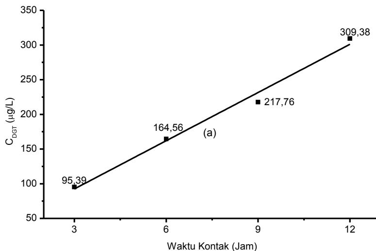
Gambar 4. Pengaruh Waktu Kontak Terhadap Konsentrasi Cu(II) yang Terikat pada Gel Selulosa– dietilentraina dengan Lapisan Difusi Gel Poliakrilamida.
