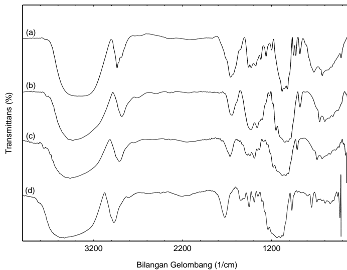
Gambar 3. Spektrum FTIR dari (a) selulosa, (b) natrium selulosa (c) epoksi selulosa (d) dietilentraina – selulosa.
