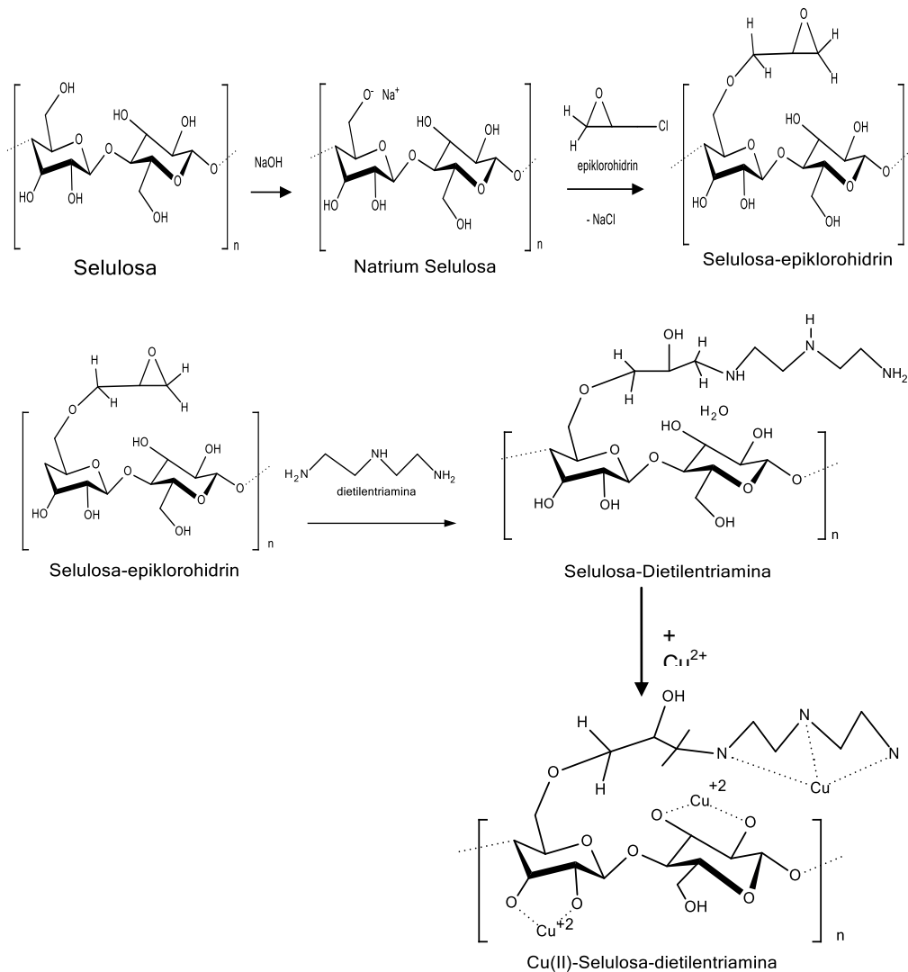
Gambar 2. Skema reaksi sintesis selulosa – dietilentriamina.
