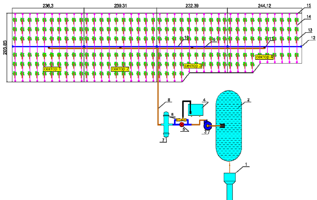
Рис. 1. План-схема ділянки крапельного поливу малини:
