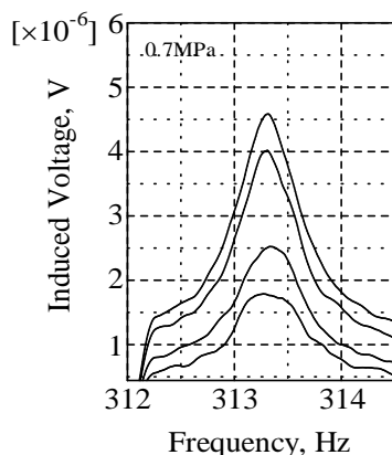
Gambar 3 Perubahan variasi tegangan input mengakibatkan naiknya puncak dari sinyal dari sekitar 1,5 sampai 4,5 μV, namun nilai frekuensi natural bernilai relatif hampir sama
