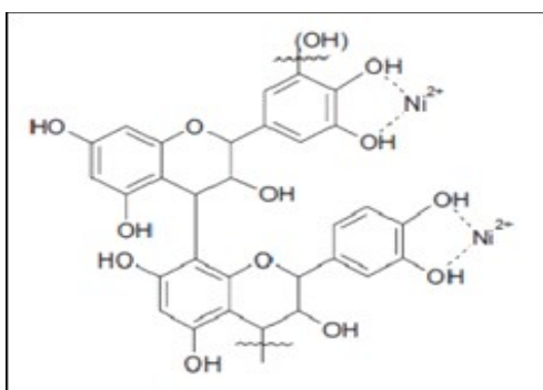
Gambar 2. Reaksi tanin dan ion nikel membentuk lapisan pasif
