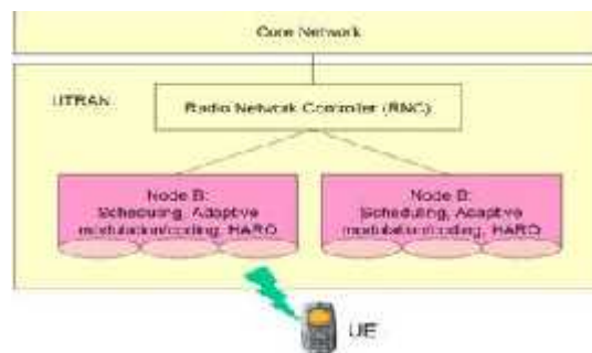
Gambar 1. Arsitektur HSDPA
