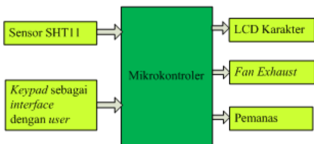
Gambar 2. Blok diagram sistem keseluruhan
