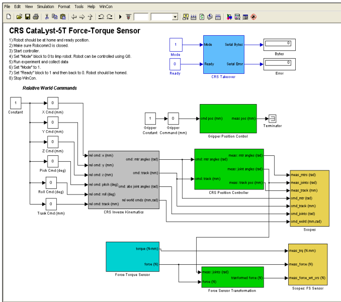
Fig. 3 Simulink model
