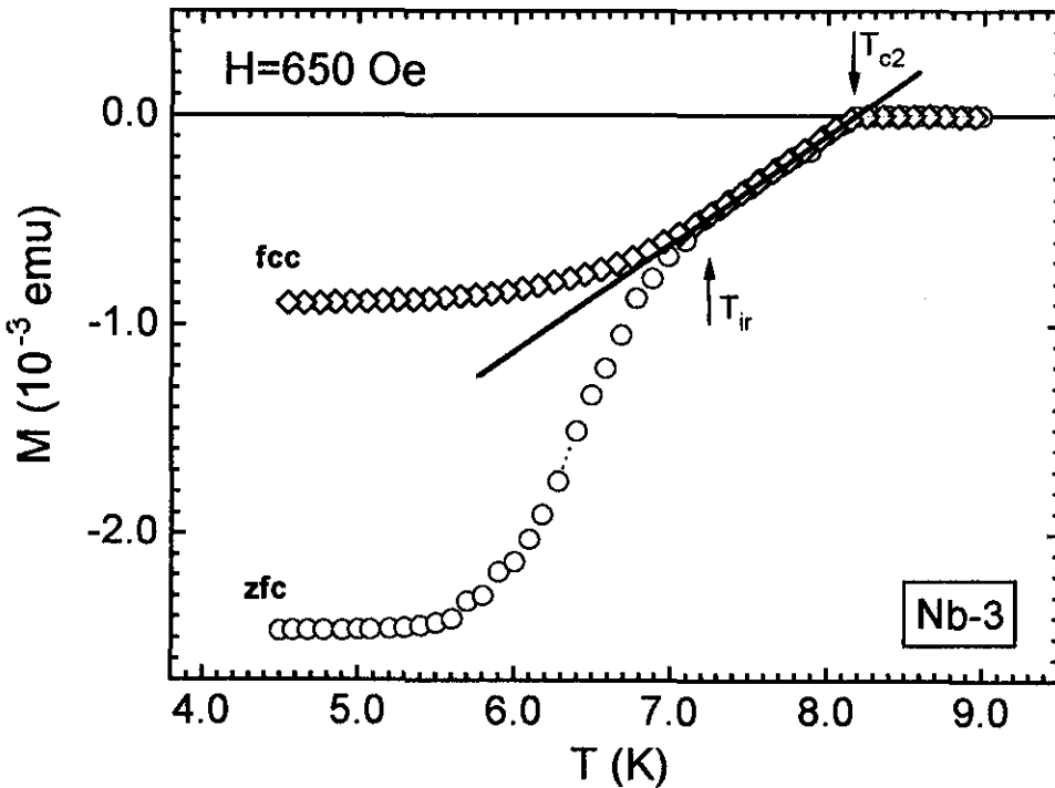
Figura (4.2) Curvas de M vs. T (zfc e fcc) para amostra Nb-3 com um campo magnético aplicado de 650 Oe, mostrando o procedimento adotado na obtenção de T_{c2} e T_{ir} .
