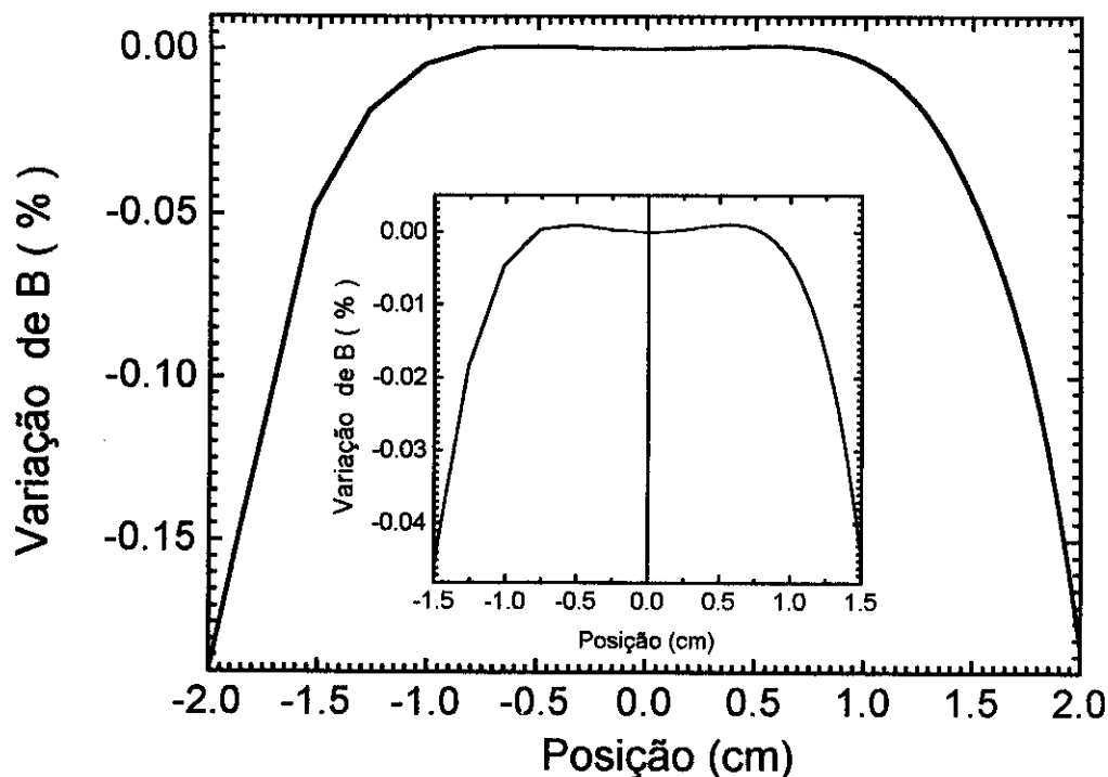
Figura (3.5) Variação do campo magnético em função da posição no magneto de 55 kOe do magnetômetro-SQUID. Na inserção temos uma ampliação mostrando a variação do campo magnético durante uma varredura de 3.0 cm. (dados extraídos da ref. [48])
