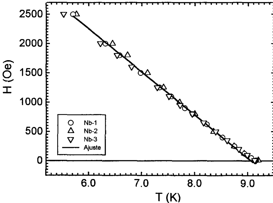
Figura (4.6) Linha de H_{c2} para as amostras Nb-1 (círculo), Nb-2 (triângulo para cima) e Nb-3 (triângulo para baixo). A linha contínua mostra o ajuste da aproximação linear para H_{c2}(T) (eq. 4.1) para a amostra Nb-3, com H_{c2}^* = 6174 Oe e T_c = 9.13 K.
