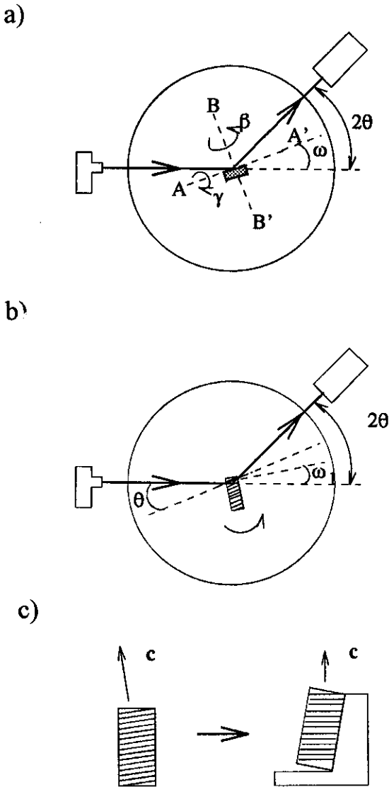
Figura (3.16) a) Esquema do método para orientação de monocristais, o detector é posicionado em um ângulo 2\theta e a amostra é girada em relação aos eixos AA' , BB' e o eixo difratômetro até obter-se um máximo na intensidade do feixe difratado. b) Esquema do procedimento utilizado na localização do eixo c da amostra YMT. c) Montagem da amostra YMT, mostrando a posição do eixo c em relação às faces da amostra, as ranhuras representam a posição dos planos ab.
