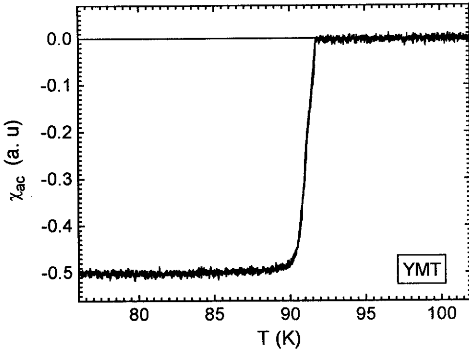
Figura (3.15) Curva de \chi' vs. T da amostra YMT, tomada em uma frequência de 10 Hz e h_{ac}=0.1 Oe, na qual é indicada sua T_c = 91.0 K ( \Delta T_c = 1.18 K).
