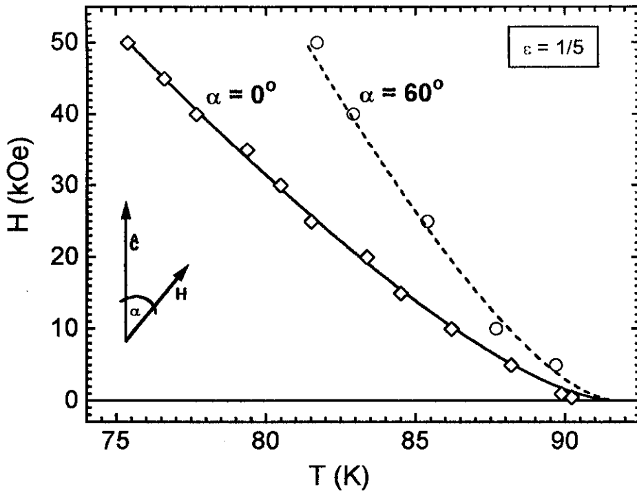
Figura (5.5) Diagrama H vs. T para amostra YMT, mostrando os dados da linha de irreversibilidade para \alpha=0^\circ ( H//c ) e \alpha=60^\circ . A linha cheia ( \alpha = 0^\circ ) e a tracejada ( \alpha = 60^\circ ) representam os ajustes da equação de fusão com correções quânticas, de acordo com a equação (5.3).
