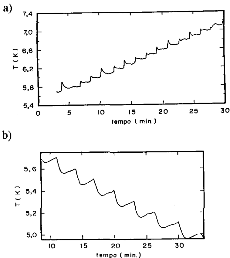
Figura (3.7) Comportamento típico da temperatura em função do tempo no magnetômetro-SQUID em baixas temperaturas (intervalo de 5-10 K), quando a temperatura é variada em passos de 0.1 K: a)aquecimento e b)resfriamento.
