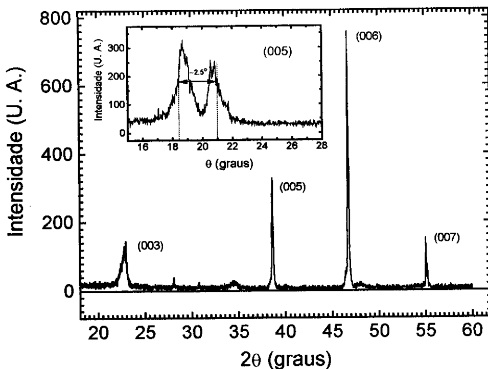
Figura (3.17) Difratoograma \theta - 2\theta da amostra YMT já orientada. Este difratoograma apresenta apenas picos na direção (00\ell) , o que demonstra o bom alinhamento da amostra. Na inserção da figura temos a varredura em \theta (rocking curve) da amostra já orientada, mostrando a pequena dispersão ( \Delta\theta \sim 2.5^\circ ) dos eixos c dos grãos.
