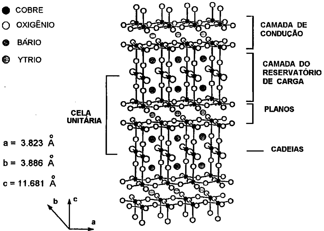
Figura (5.1) Estrutura química do \text{YBa}_2\text{Cu}_3\text{O}_{6+x} mostrando as camadas de condução alternadas com camadas que funcionam como reservatórios de carga. As camadas de condução consistem de 2 planos de \text{CuO}_2 separados por átomos de Y. Os reservatórios de carga consistem de cadeias de \text{CuO}_x estendidas ao longo da direção b. O oxigênio contido nas cadeias de \text{CuO}_x varia entre 0 a 1.
