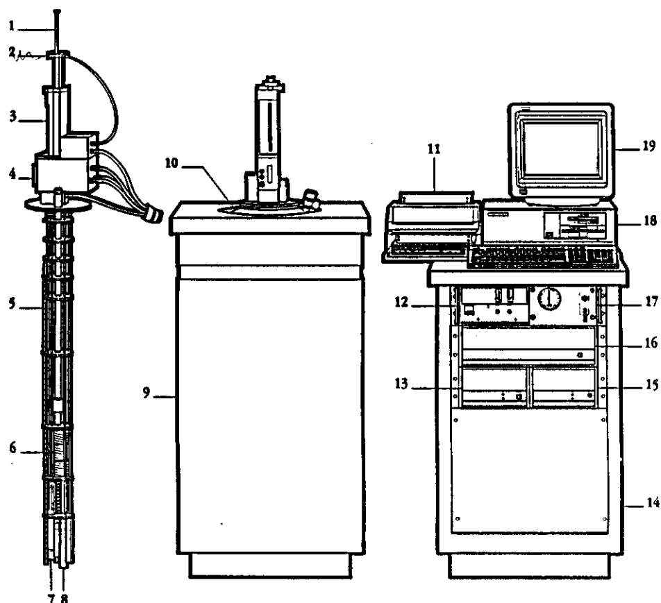
Figura (3.1) Diagrama do magnetômetro-SQUID mostrando os diversos componentes. 1)Suporte de amostra, 2)Mecanismo para girar a amostra, 3)Mecanismo para o transporte da amostra, 4)Visor, 5)Sensor de nível do He, 6)Magneto supercondutor, 7)Impedância de fluxo (para controle de temperatura), 8)Capsula do sensor SQUID, 9)Gabinete do Dewar, 10)Dewar, 11)Impressora, 12)Fonte do magneto, 13)Controlador de temperatura, 14)Gabinete, 15)Unidade de controle geral de potência, 17)Unidade de controle do fluxo de gás, 18)Computador, 19)Monitor. (extraído da ref. [48])
