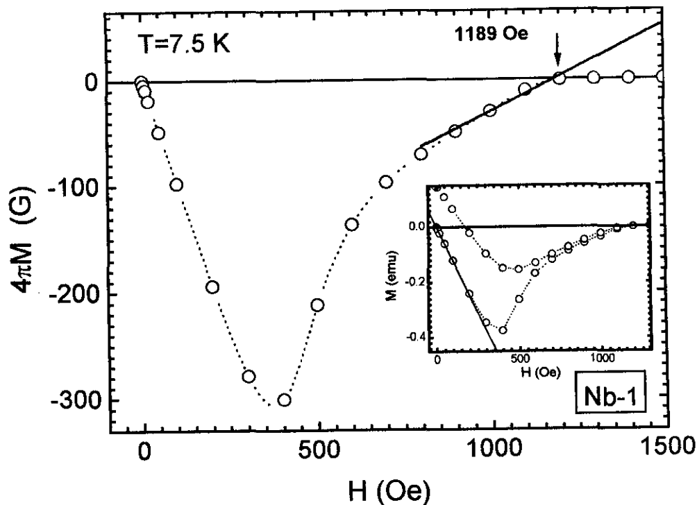
Figura (3.12) Curva de 4\pi M vs. H , com a magnetização dada em Gauss, tomada a temperatura constante, T=7.5 K, na subida do campo magnético. Esta curva foi integrada e o valor do H_c , H_c=544 G, obtido utilizando-se a equação (4.4). O valor de H_{c2} , H_{c2}=1189 Oe, também é indicado nesta curva. Na inserção temos a curva original (subida e descida), com a M dada em “emu”. A reta contínua é o ajuste dos primeiros pontos da curva de magnetização e mostra inclinação do trecho diamagnético, H_{c1} , utilizado na normalização da curva.
