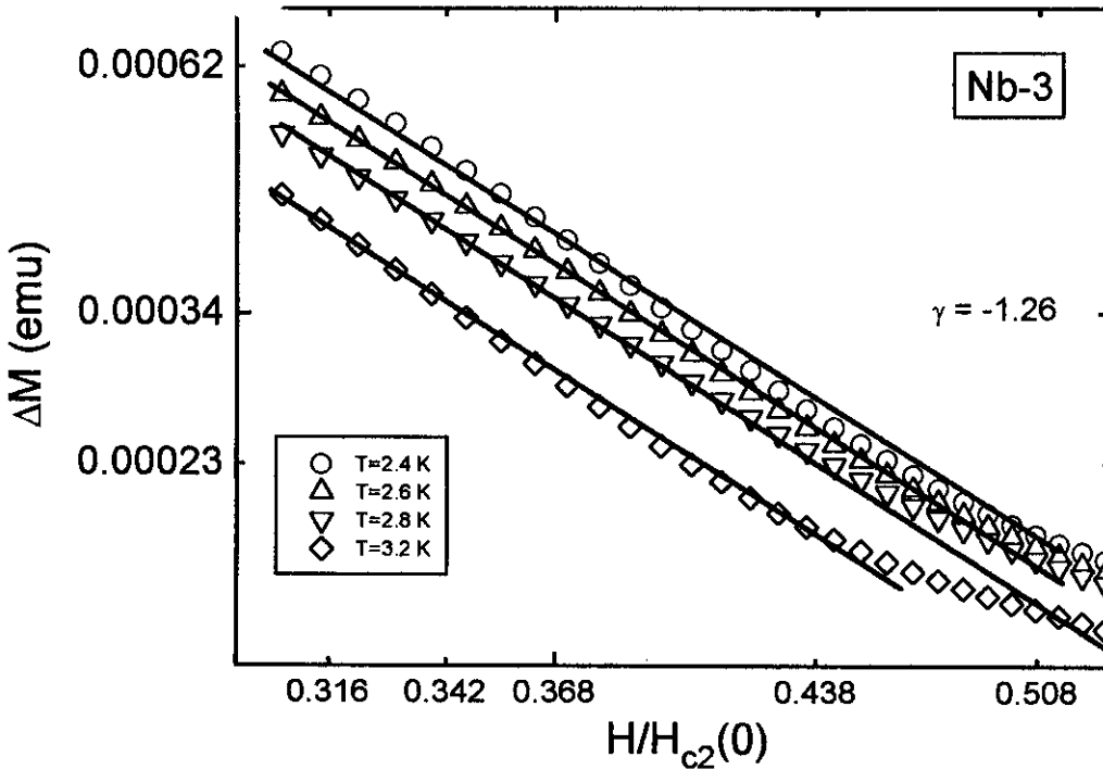
Figura (4.10) Gráfico de \Delta M vs. H/H_{c2}(0) em escala logarítmica dupla ( \ln ), para diferentes temperaturas. Como H_{c2}(0) foi utilizado aqui H_{c2} obtido do ajuste da aproximação linear para H_{c2} . As linhas cheias são paralelas e sua inclinação corresponde ao expoente \gamma da equação (2.7), \gamma = -1.26 .
