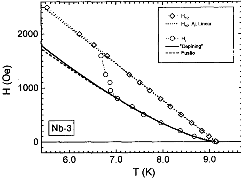
Figura (4.5) Linha de irreversibilidade (círculo) e de H_{c2} (losango) da amostra Nb-3. A linha pontilhada mostra o ajuste da aproximação linear para H_{c2}(T) (eq. 4.1), com H_{c2}^* = 6174 Oe e T_c = 9.13 K. A linha tracejada mostra o ajuste da equação para a fusão da rede (eq. 2.23) ao dados da linha de irreversibilidade, com c_L = 0.0036 e a linha contínua mostra o ajuste da equação para o "depining" termicamente ativado (eq. 2.22), com n = 1.40 .
