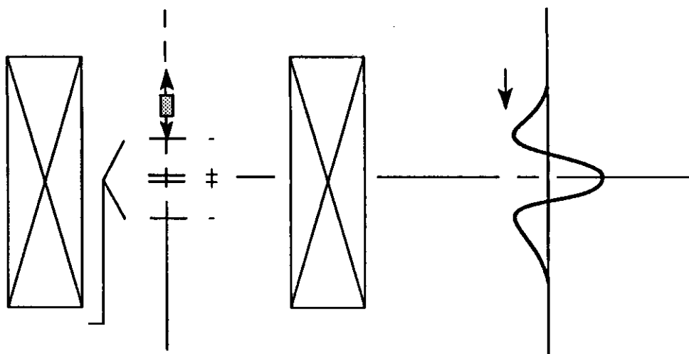
Figura (3.2) Esquema mostrando a bobina coletora do magnetômetro-SQUID e a movimentação da amostra no seu interior. Ao lado temos uma curva típica de tensão vs. posição da amostra. (extraído da ref. [48])
