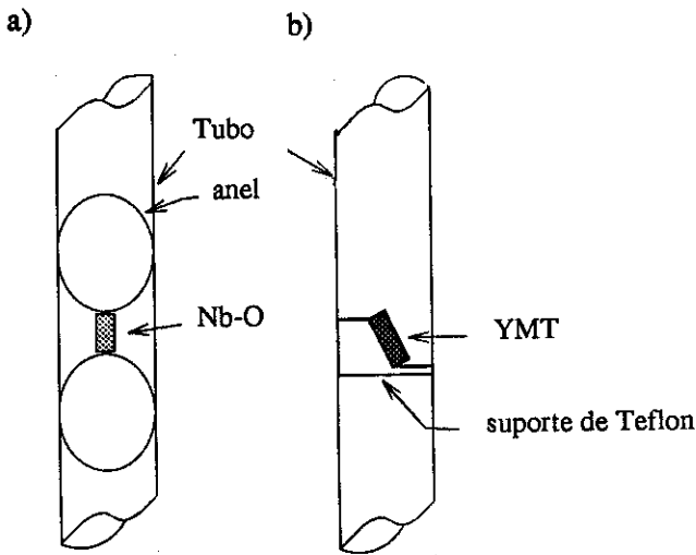
Figura (3.4) Alguns dos suportes de amostra utilizados para as medidas no magnetômetro-SQUID. a) Suporte da amostra Nb-O, similar aos utilizados com as amostras Nb-2 e Nb-3. b) Suporte da amostra de \text{YBa}_2\text{Cu}_3\text{O}_{7.8} (amostra YMT)
