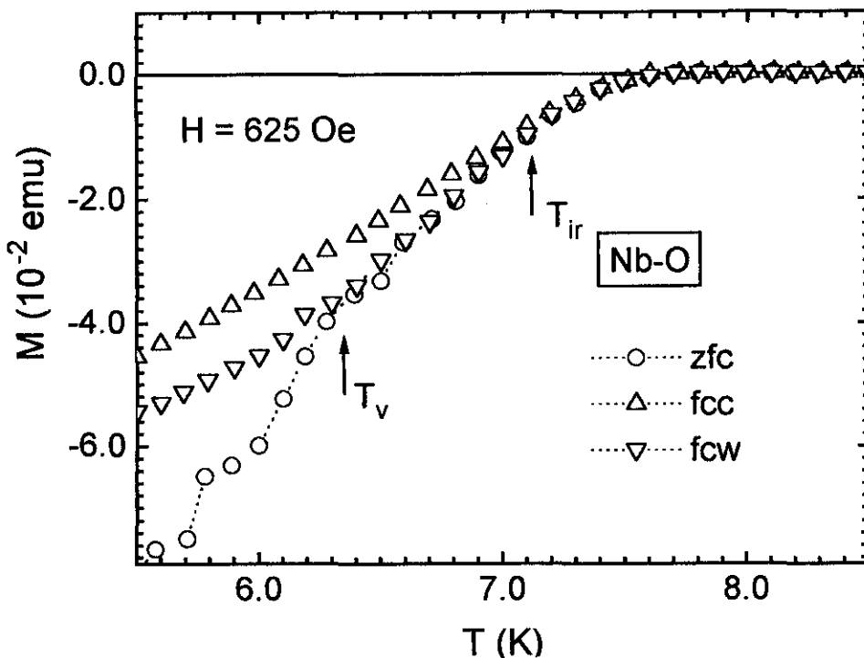
Figura (3.18) Curvas M vs. T obtidas com diferentes histórias termo-magnéticas. Amostra Nb-O com um campo aplicado de 625 Oe.
