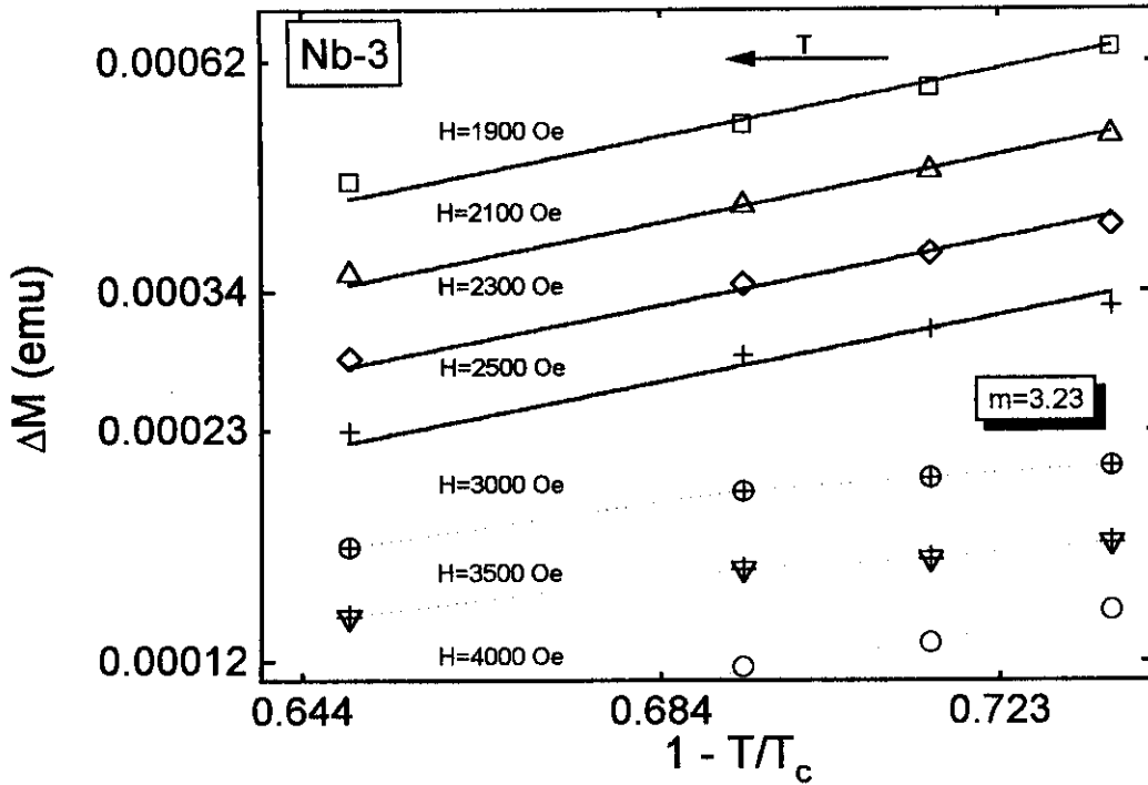
Figura (4.9) Gráfico de \Delta M vs. (1-T/T_c) em escala logarítmica dupla ( \ln ), para diferentes valores do campo magnético. As linhas cheias são paralelas e sua inclinação corresponde ao expoente m da equação (2.7), m = 3.23 . A seta no topo do gráfico indica o sentido de aumento da temperatura.
