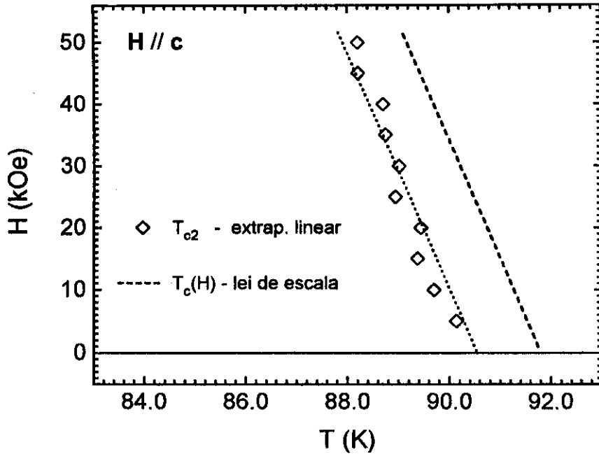
Figura (5.4) Diagrama H vs. T , para a amostra YMT, mostrando o deslocamento da linha H_{c2}(T) para temperaturas mais elevadas, como resultado do ajuste da lei de escala para flutuações do parâmetro de ordem (ver seção 5.2).
