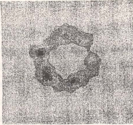
Figura (2.4) Padrão de difração de neutrons da rede de fluxóides de um monocristal de \text{Bi}_{2.15}\text{Sr}_{1.95}\text{Ca}_2\text{O}_{8+x} , em um campo H = 475 Oe e T = 1.1 K (extraído da ref. [26]).
