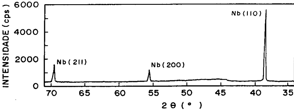
Figura (3.14) Difratoograma \theta - 2\theta para o pó Nb-O mostrando os principais picos de difração de raios-x.
