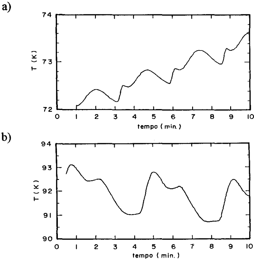
Figura (3.8) Comportamento típico da temperatura em função do tempo no magnetômetro-SQUID em altas temperaturas (intervalo de 70-100 K), quando a temperatura é variada em passos de 0.4 K: a)aquecimento e b)resfriamento. Pode-se observar que o tempo de estabilização da temperatura é muito maior no resfriamento.
