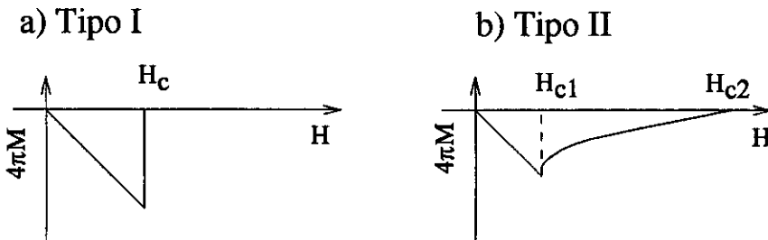
Figura (2.1) Curvas de magnetização reversível ( M vs H ) típicas, mostrando os campos críticos: a) supercondutor do tipo I, b) supercondutor do tipo II.
