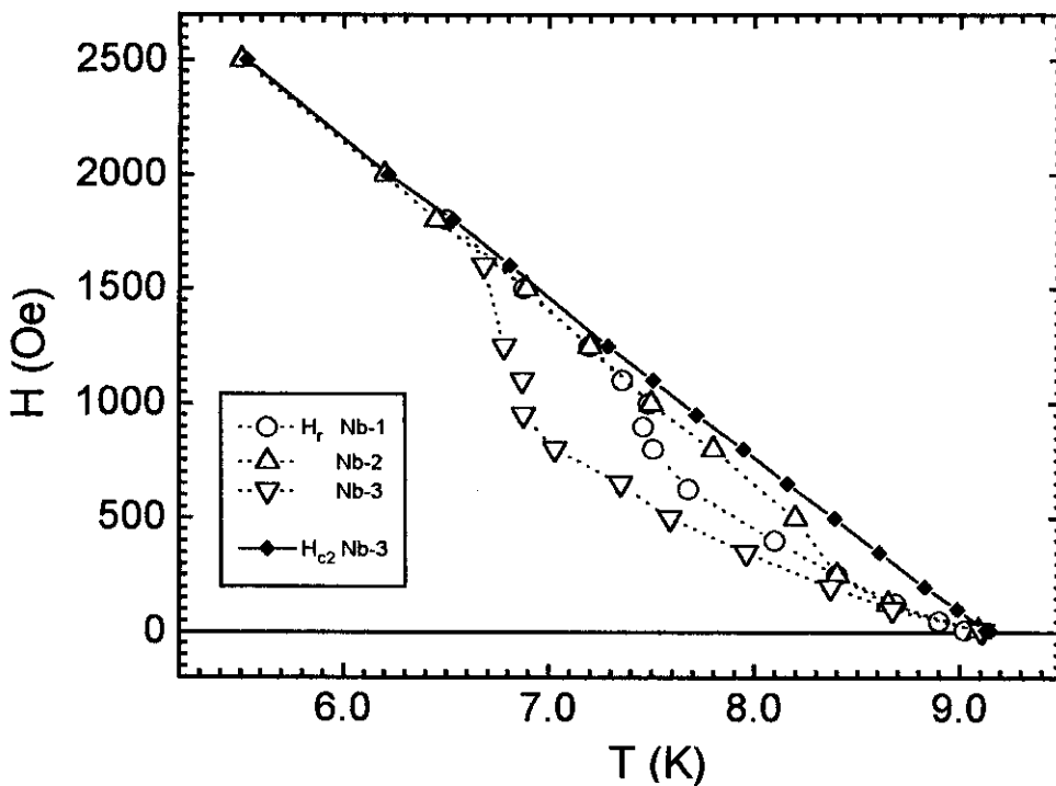
Figura (4.7) Linha de irreversibilidade para as amostras Nb-1 (circulo), Nb-2 (triângulo para cima) e Nb-3 (triângulo para baixo) e linha de H_{c2} para a amostra Nb-3 (losango preenchido).
