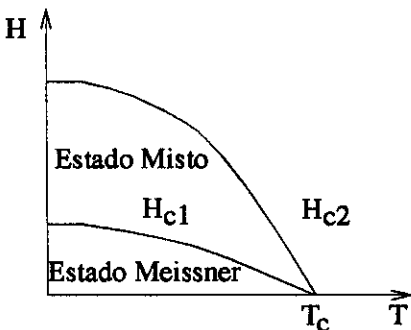
Figura (2.2) Diagrama de Fase ( H vs. T ) para um supercondutor do tipo II
