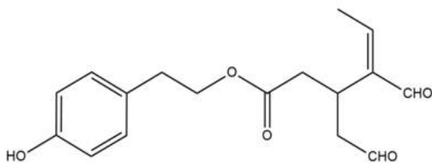
ligstrosídeo aglicona decarboximetilado
