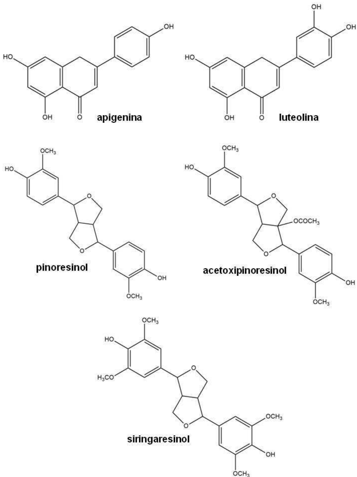
Figura 1.5. Estrutura de compostos fenólicos previamente identificados em azeite de oliva extravirgem (continuação).
