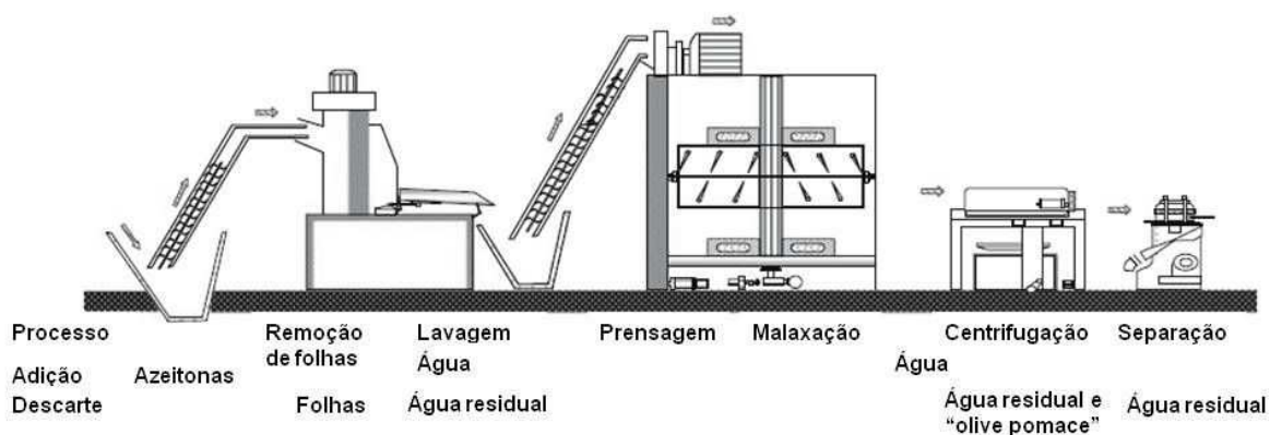
Figura 1.1. Planta de extração de azeite de oliva extravirgem moderna. Fonte: Adaptado de Kapellakis, Tsagarakis & Crowther (2008).
