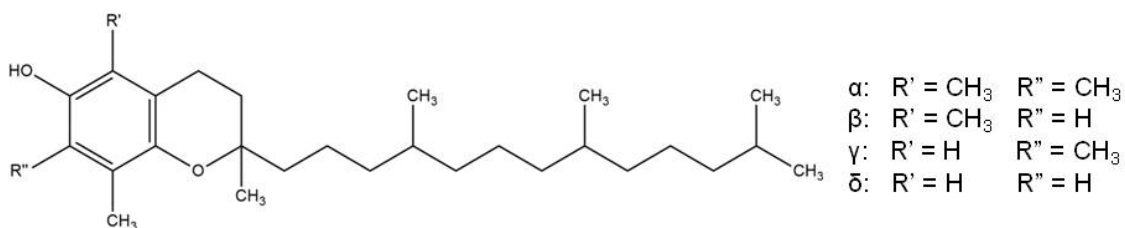
Figura 1.6. Estrutura dos quatro principais isômeros de tocoferóis presentes em azeite de oliva extravirgem.
