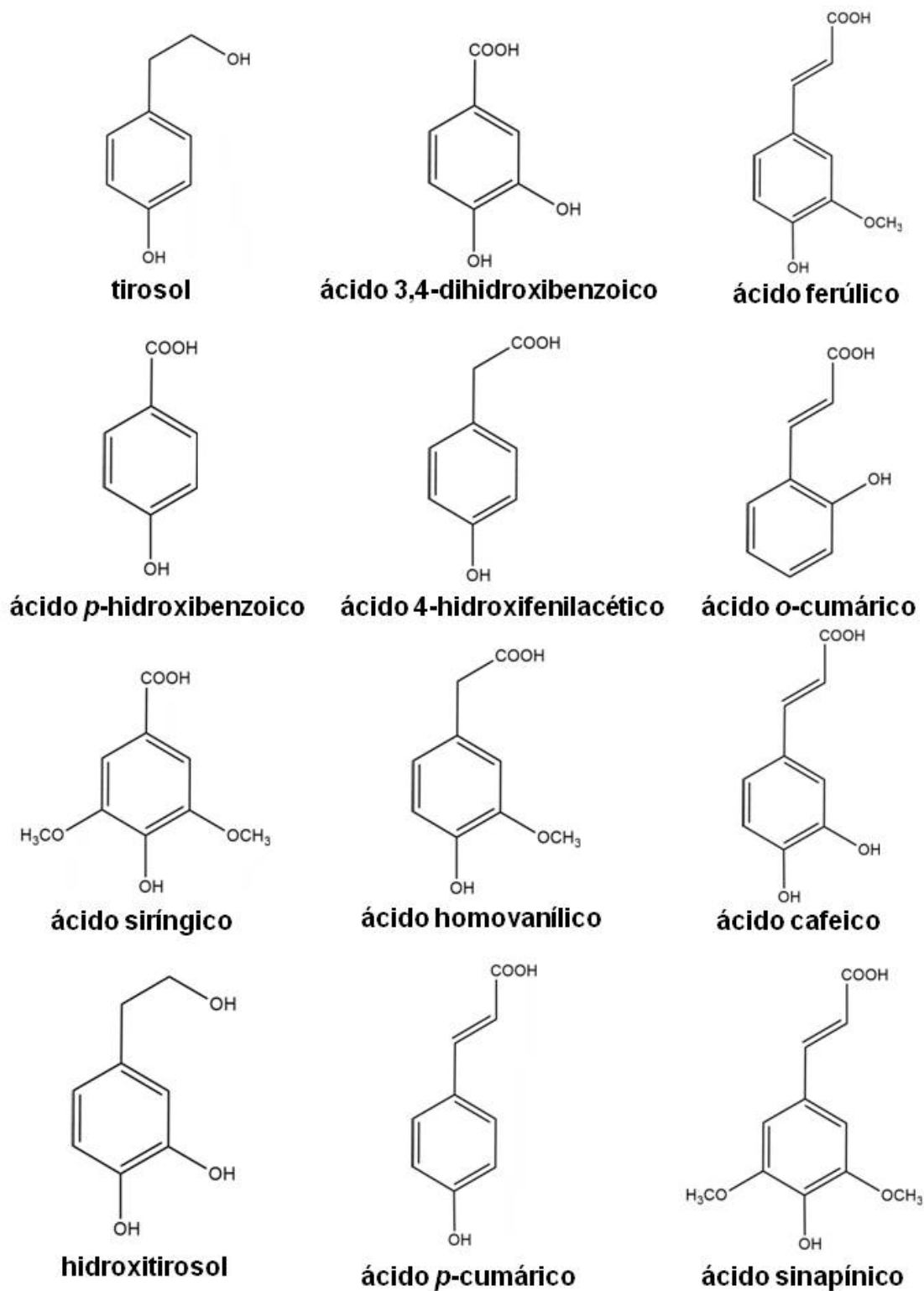
Figura 1.2. Estrutura de compostos fenólicos previamente identificados em azeite de oliva extravirgem.
