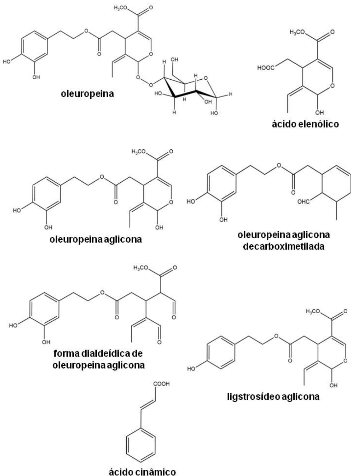
Figura 1.3. Estrutura de compostos fenólicos previamente identificados em azeite de oliva extravirgem (continuação).
