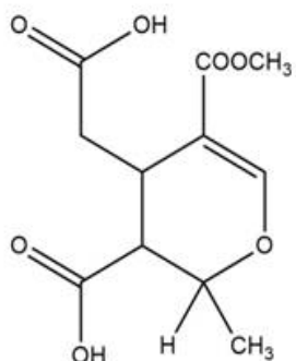
ácido elenólico hidroxilado
