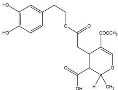
forma hidroxilada de oleuropeina aglicona
