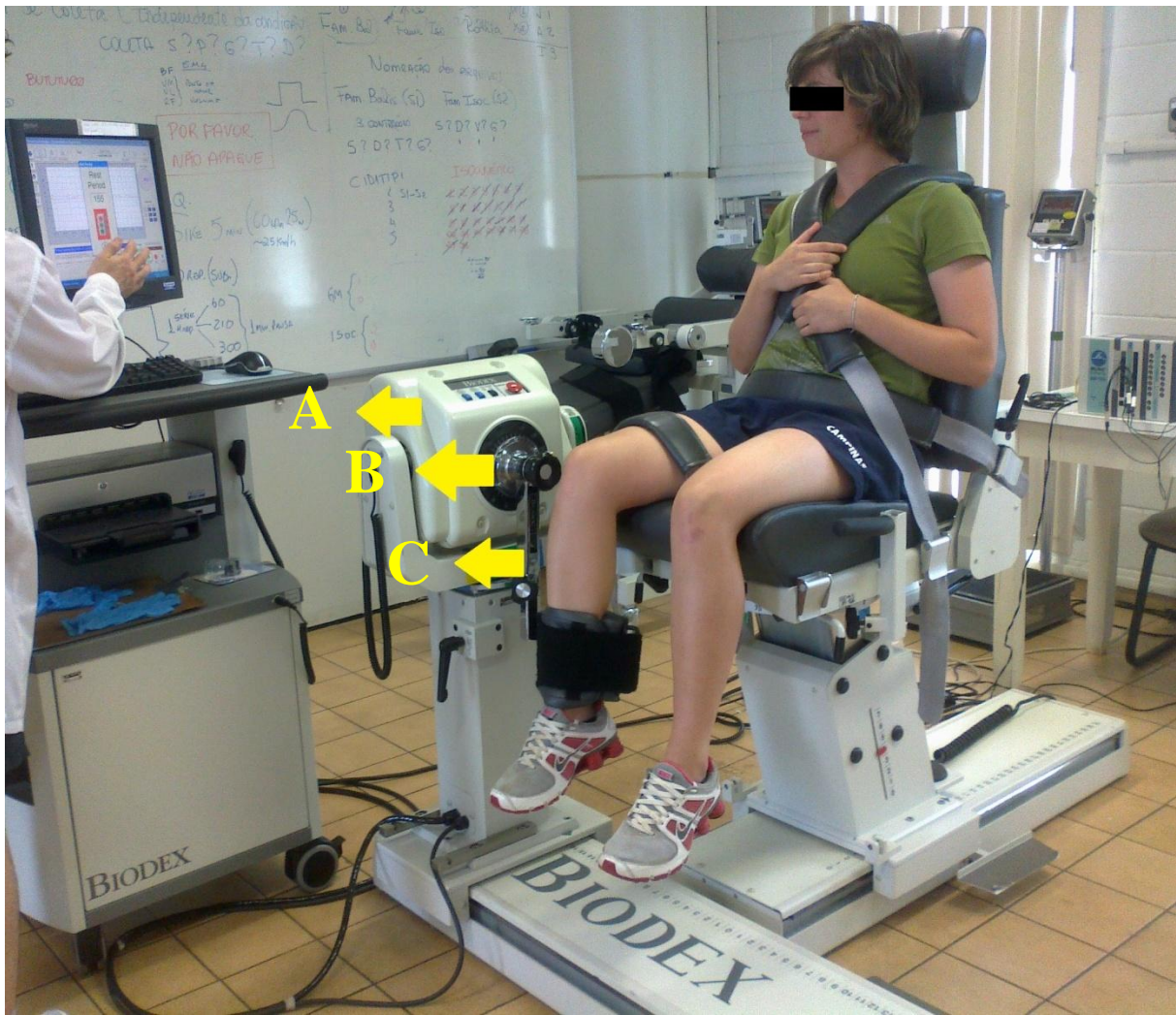
Figura 1. Exemplo de um dinamômetro isocinético. A = Braço de alavanca; B = localização da célula de carga; C = Unidade de aceitação de força.
