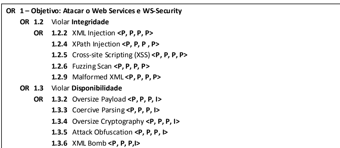
Figura 8.2 Árvore de ataque textual para Web Services com WS-Security.
