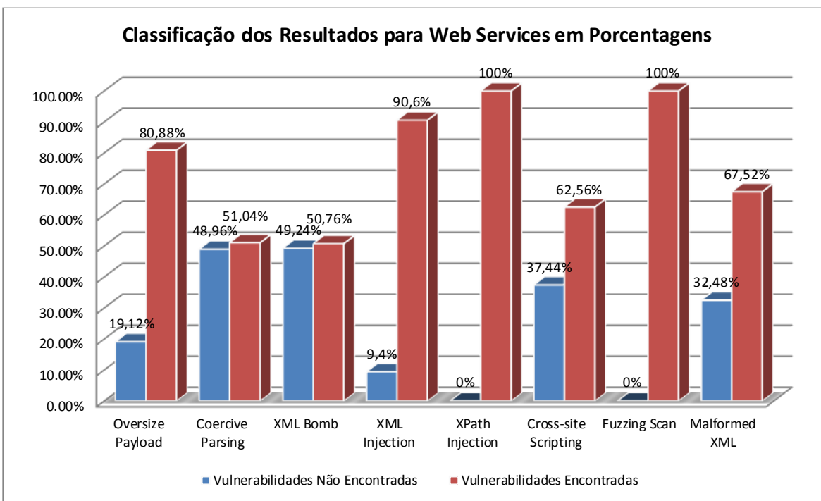
Figura 8.11 Análise dos resultados para Web Services.
