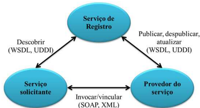
Figura 2.3 Atores e operações de Web Services.
