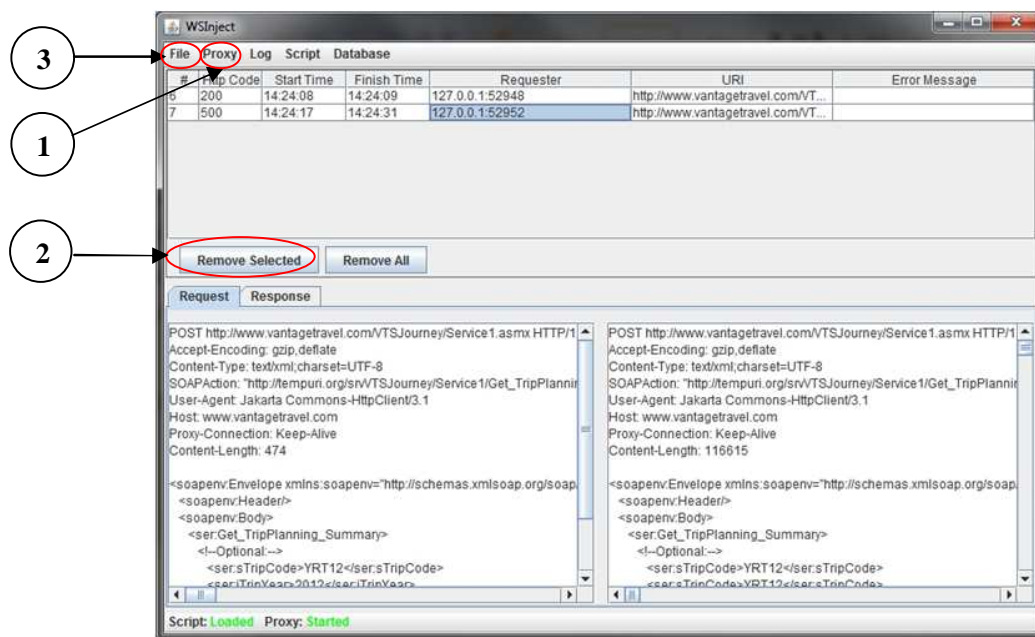
Figura 6.3 WSInject em funcionamento.
