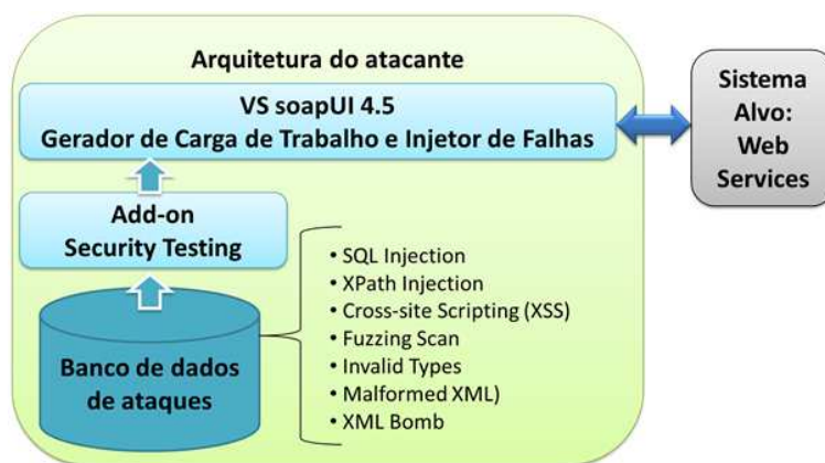
Figura 7.3 Arquitetura do VS soapUI com add-on Security Testing.
