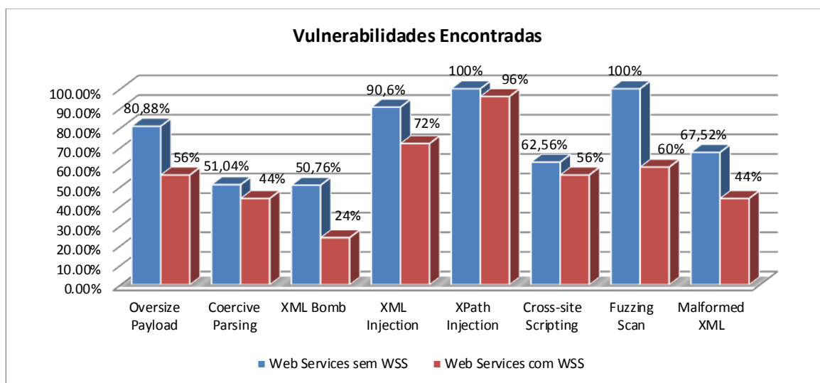
Figura 8.14 Comparação das duas abordagens para ataques bem sucedidos AS.
