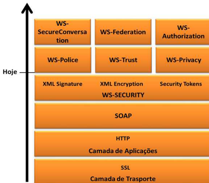
Figura 3.3 Mecanismos de segurança para Web Services.
