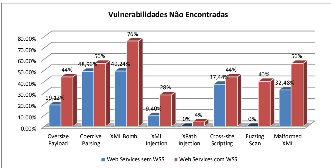
Figura 8.13 Comparação das duas abordagens para Vulnerabilidades Não Encontradas.
