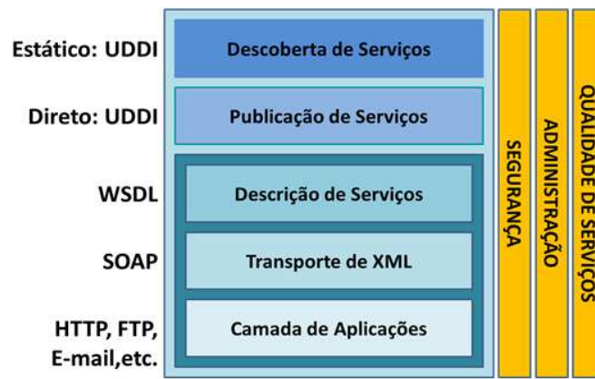
Figura 2.2 Pilha de padrões de Web Service.
