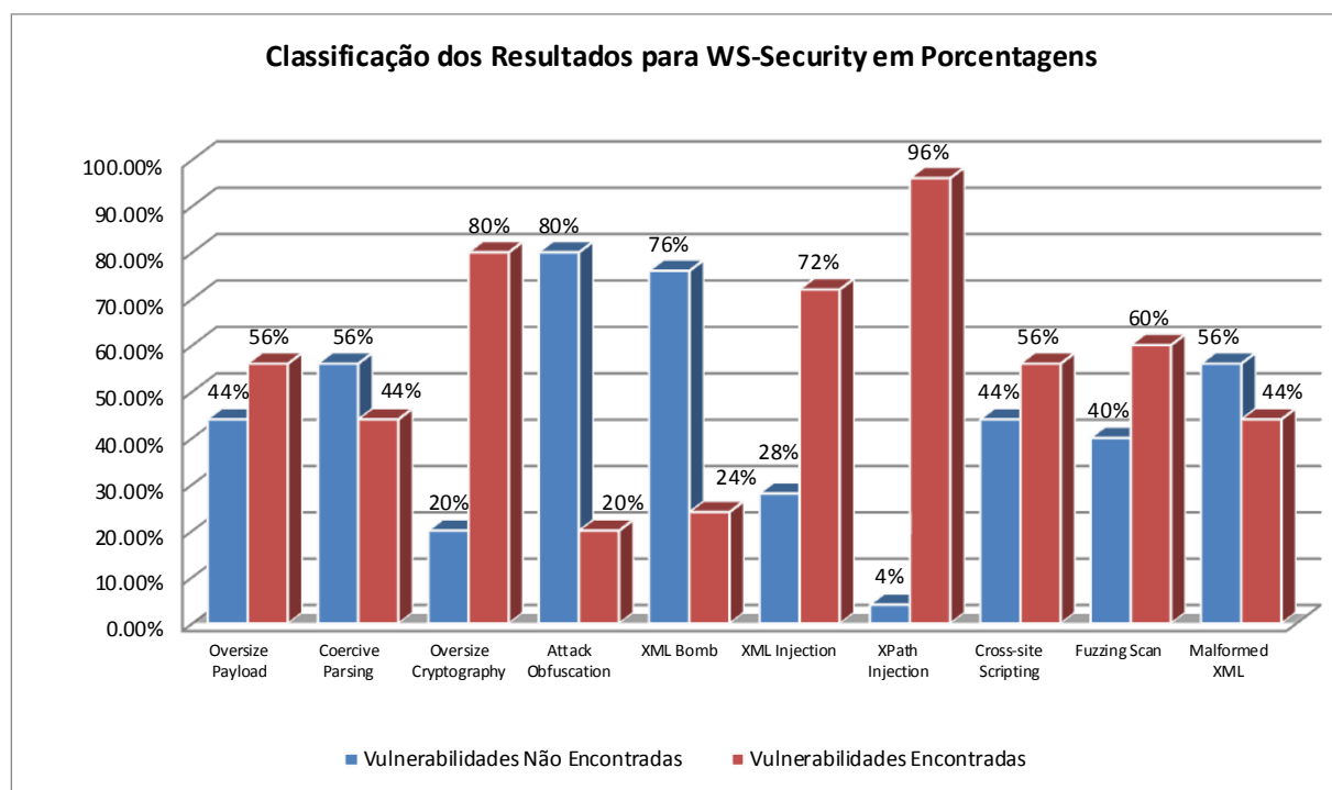
Figura 8.12 Análise dos resultados para WS-Security.
