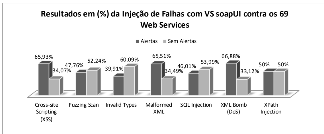
Figura 7.5 Ataques contra os 69 Web Services.
