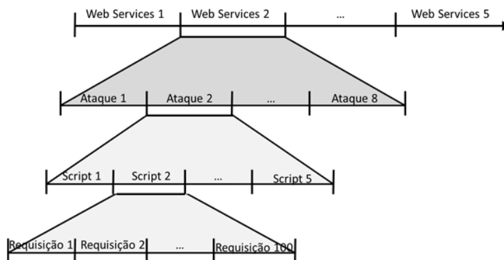
Figura 8.7 Campanha de Injeção de Ataques contra Web Services.
