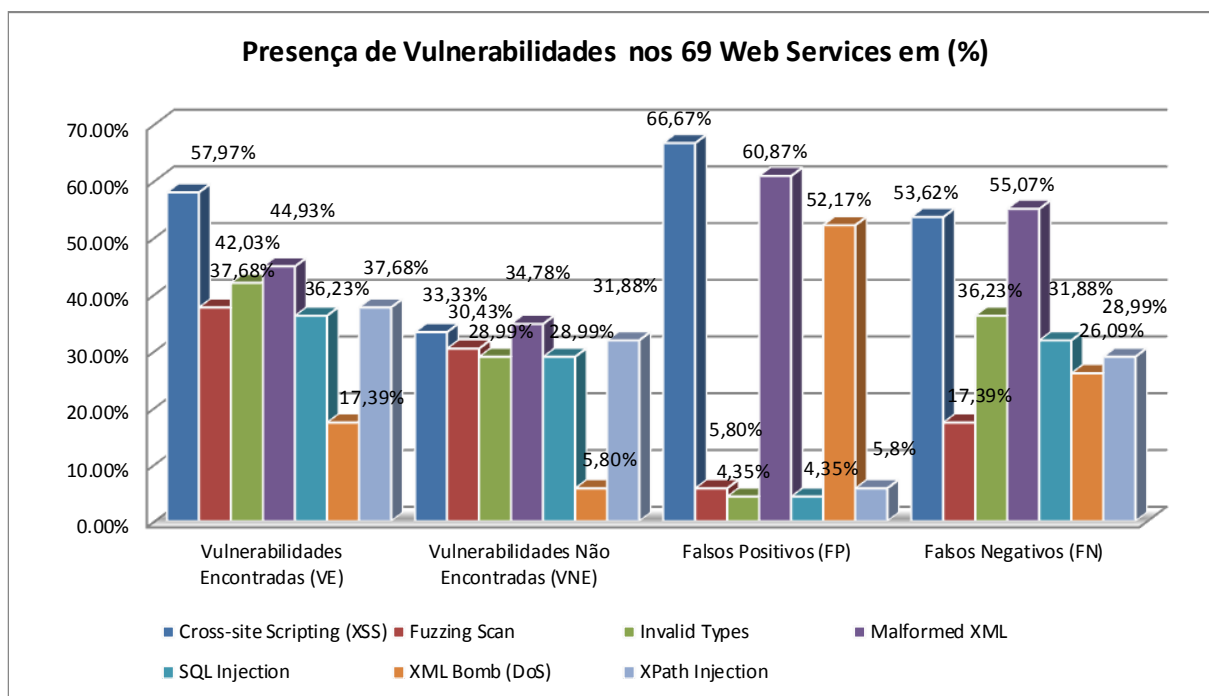
Figura 7.14 Presença de vulnerabilidades detectadas nos 69 Web Services em porcentagens.
