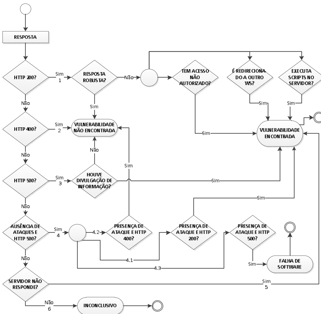
Figura 7.8 Análise de repostas para Web Services.
