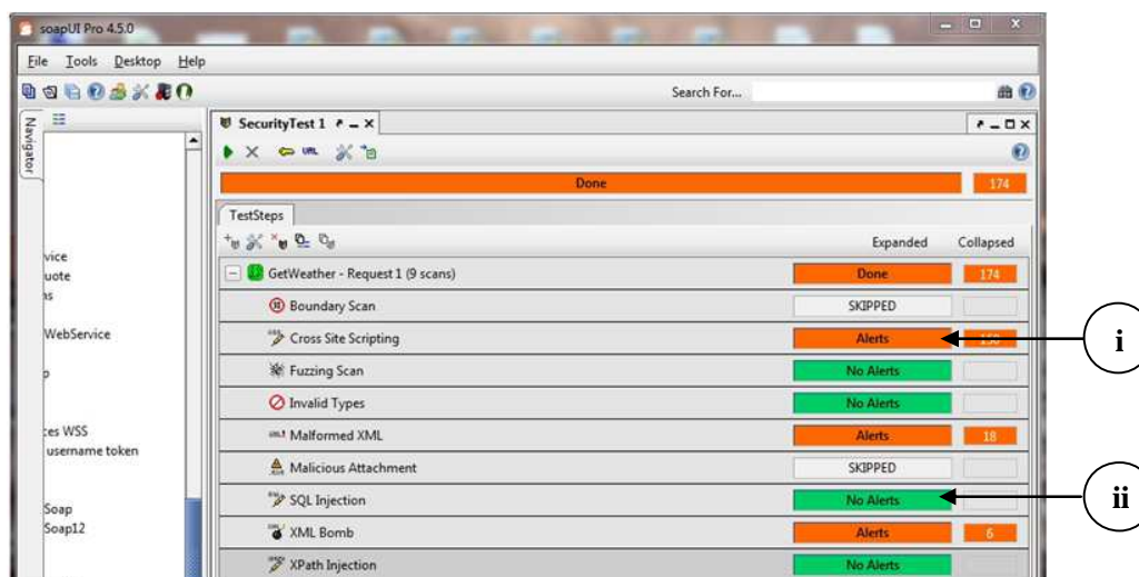
Figura 7.4 Execução do Security Testing no soapUI em um Web Service.
