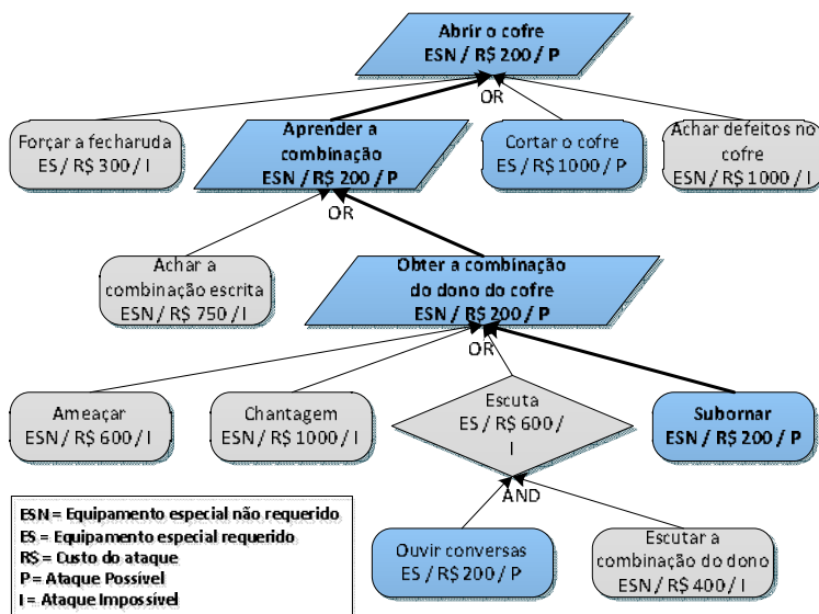
Figura 3.15 Árvore de ataques para abrir o cofre.
