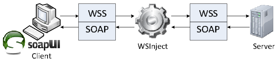
Figura 8.1 Arquitetura de testes para a fase de injeção de falhas.
