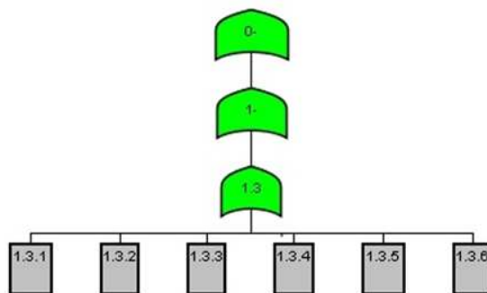
Figura 6.8 Sub-árvore de Ataques gráfica que Não são rejeitados por WS-Security.
