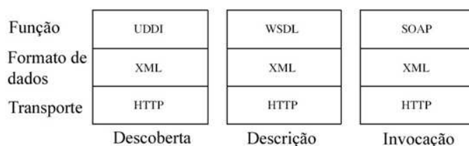
Figura 2.4 Pilha de protocolos de Web Service.
