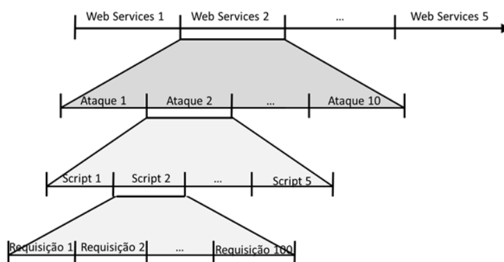
Figura 8.8 Campanha de Injeção de Ataques contra WS-Security.
