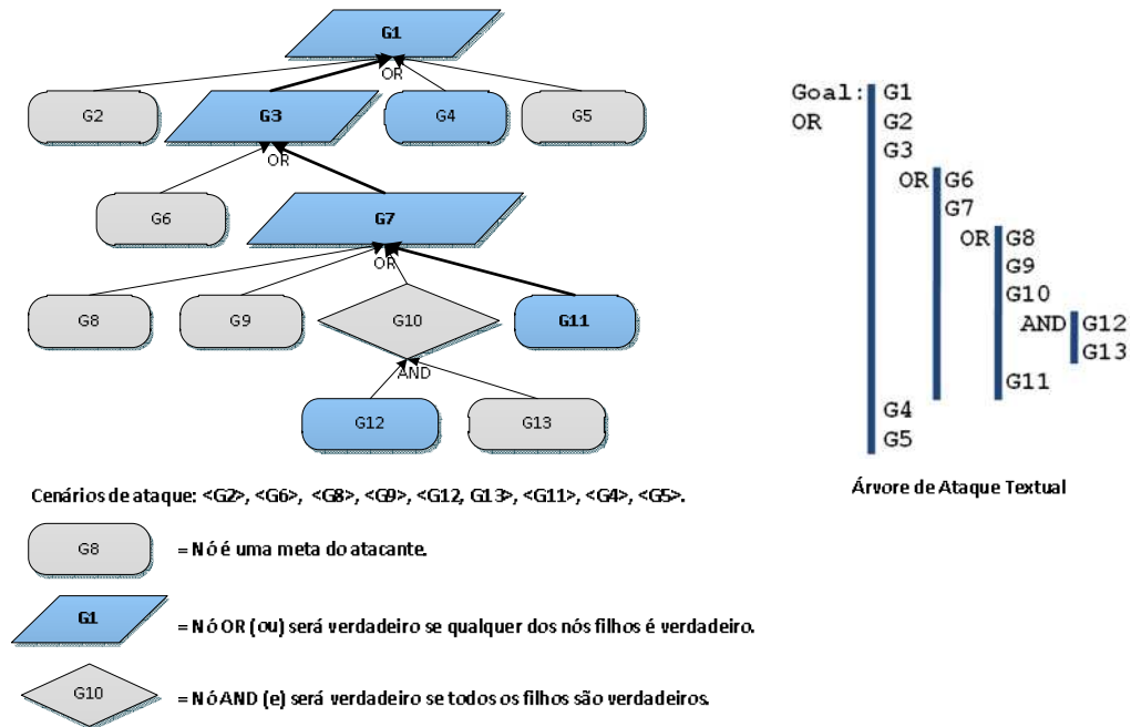
(a) Árvore de ataques gráfica
