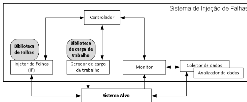
Figura 4.1 Ambiente de Injeção de Falhas.
