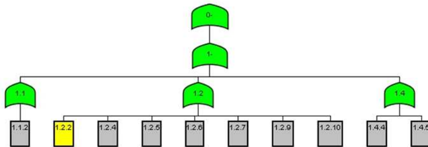
Figura 6.7 Sub-árvore gráfica de Ataques que são rejeitados por WS-Security.
