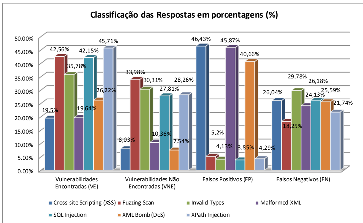
Figura 7.13 Ataques injetados pelo VS soapUI contra Web Services em (%).
