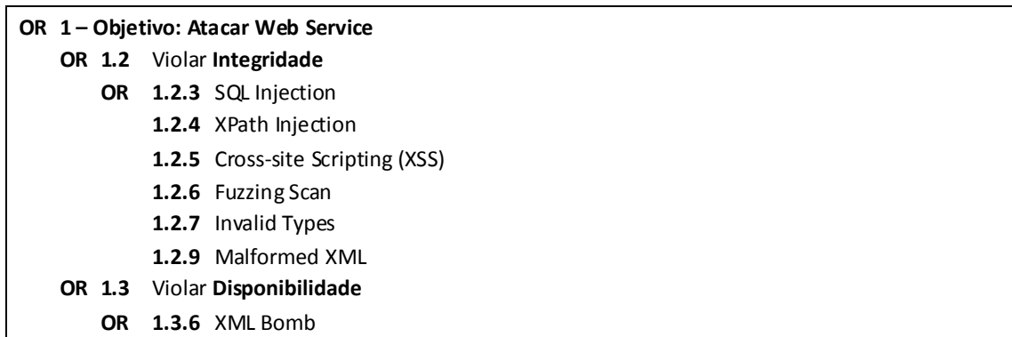
Figura 7.2 Árvore de ataque textual para o VS soapUI.
