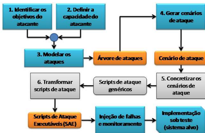
Figura 5.1 Metodologia de testes de Segurança.
