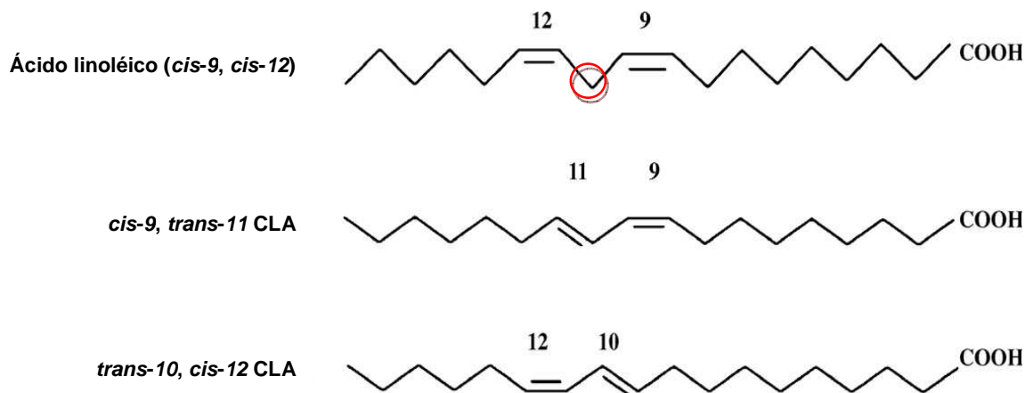
Figura 1. Estrutura do ácido linoléico ( cis -9, cis -12) e dos isômeros do CLA cis -9, trans -11 e trans -10, cis -12. Adaptado de Pariza, Park e Cook (2001).
