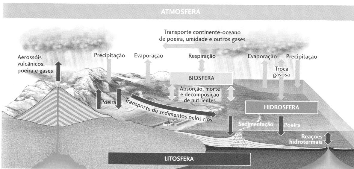
Figura 23.9 Processos de transporte entre os componentes do sistema do clima.
