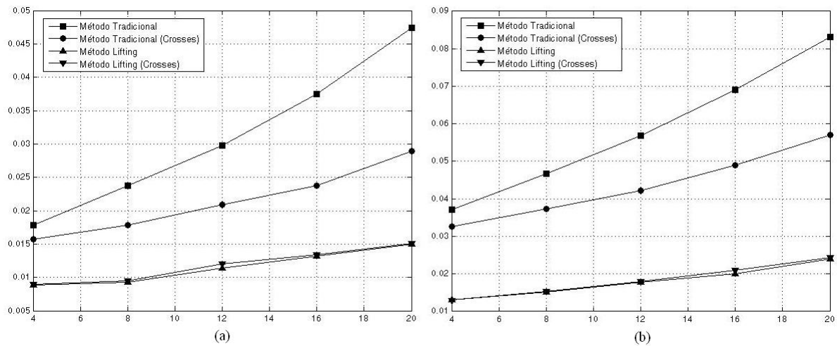
Figura 10.5: Comparação T_p \times n para wavelets Biortogonais (ordem3) para a imagem Crosses: (a) Decomposição; (b) Decomposição e reconstrução.
