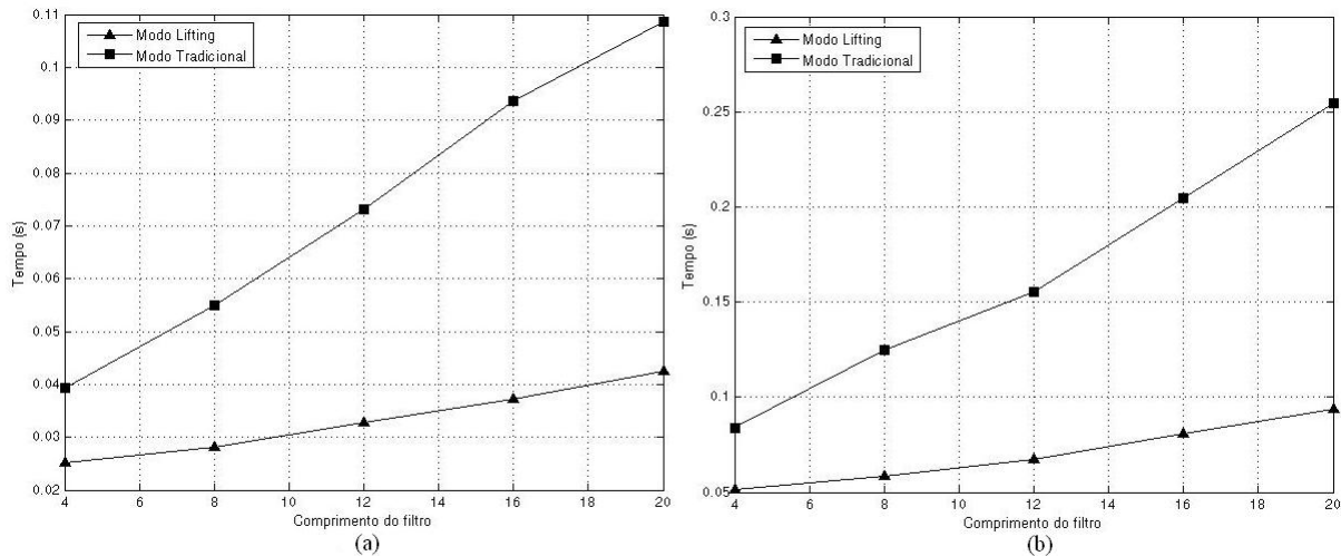
Figura 9.13: Comparação T_p \times n para wavelets Biortogonais (ordem3) utilizando ferramenta compilada: (a) Decomposição; (b) Decomposição e reconstrução.
