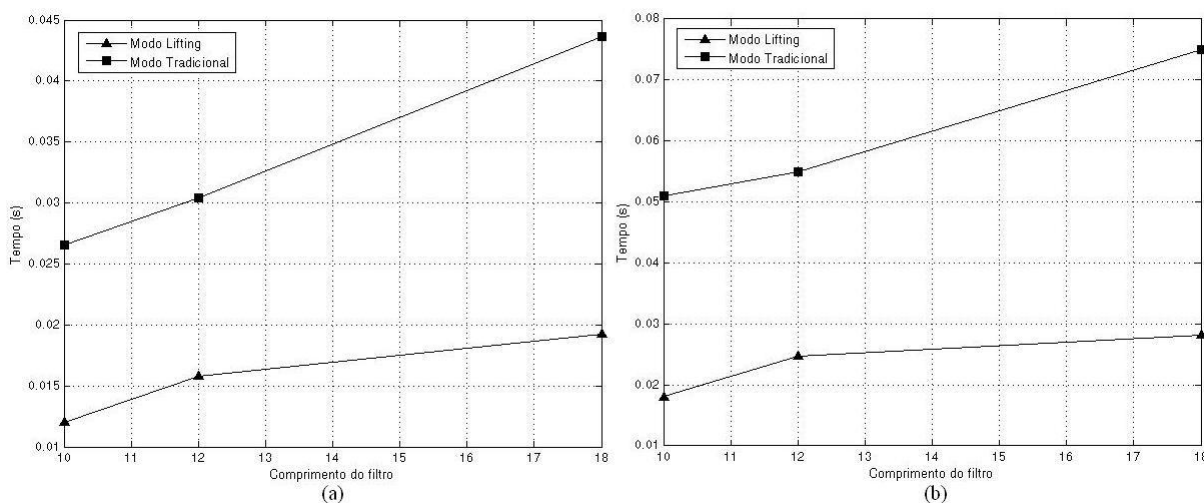
Figura 9.20: Comparação T_p \times n para wavelets Biortogonais utilizando ferramenta interpretada: (a) Decomposição; (b) Decomposição e reconstrução.
