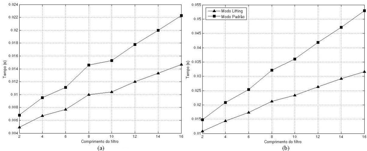
Figura 9.3: Comparação T_p \times n para wavelets Daubechies utilizando ferramenta compilada: (a) Decomposição; (b) Decomposição e reconstrução.
