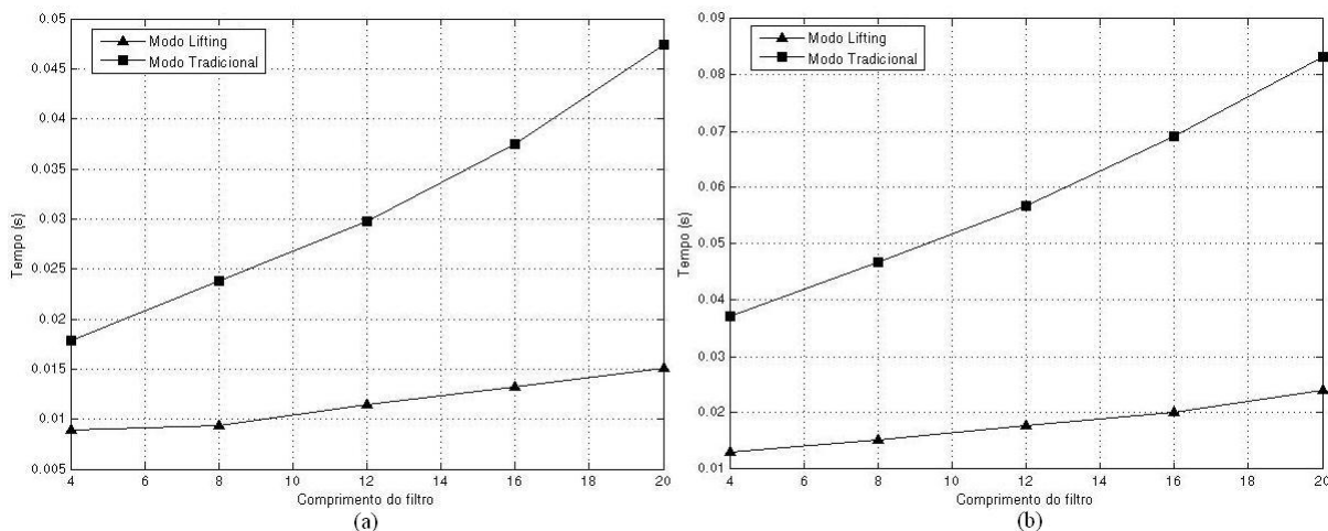
Figura 9.19: Comparação T_p \times n para wavelets Biortogonais (ordem3) utilizando ferramenta interpretada: (a) Decomposição; (b) Decomposição e reconstrução.
