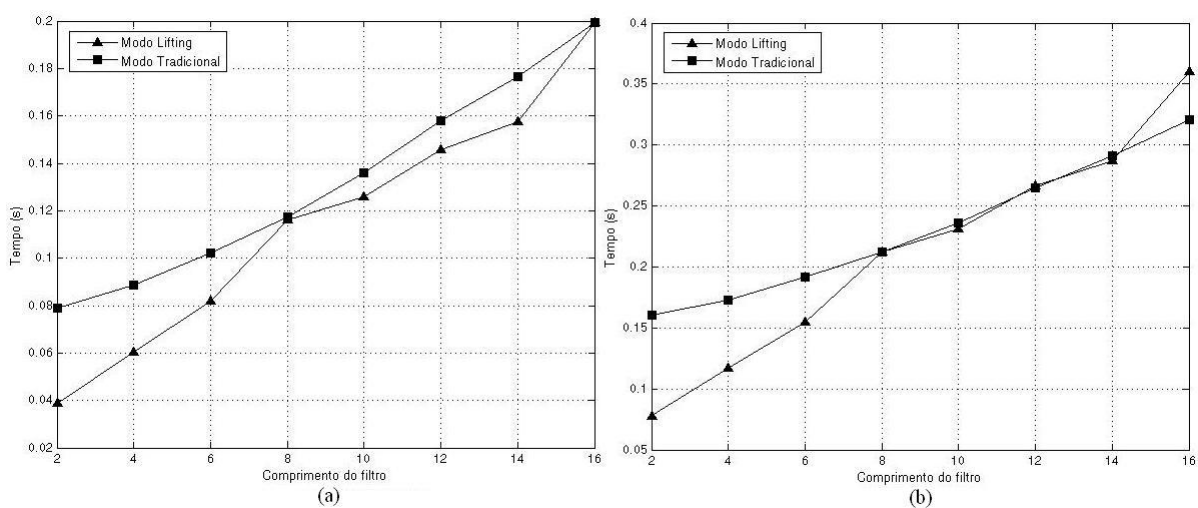
Figura 9.21: Comparação T_p \times n para wavelets de Daubechies utilizando ferramenta interpretada: (a) Decomposição; (b) Decomposição e Reconstrução.
