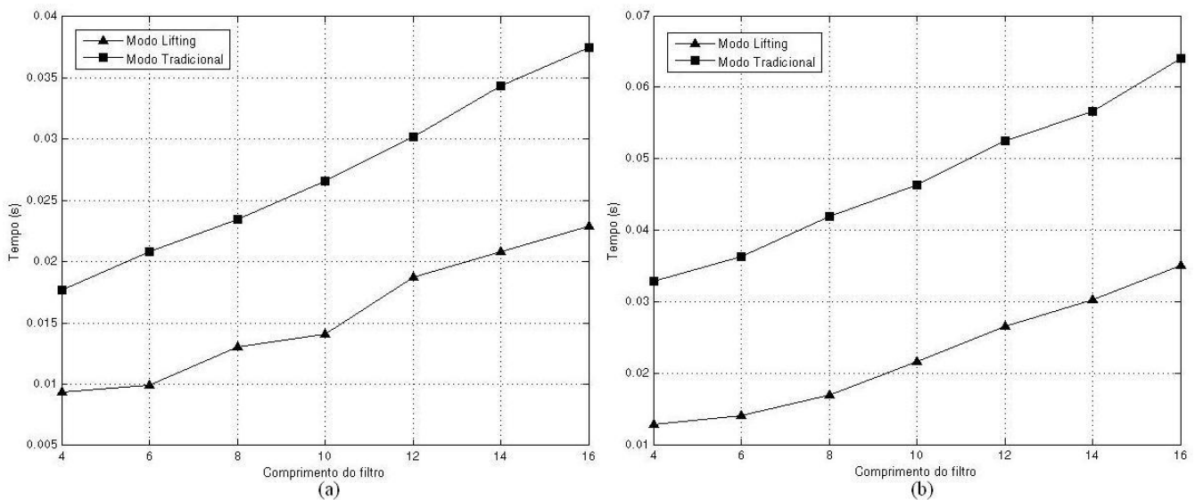
Figura 9.16: Comparação T_p \times n para wavelets Symlets utilizando ferramenta interpretada: (a) Decomposição; (b) Decomposição e reconstrução.
