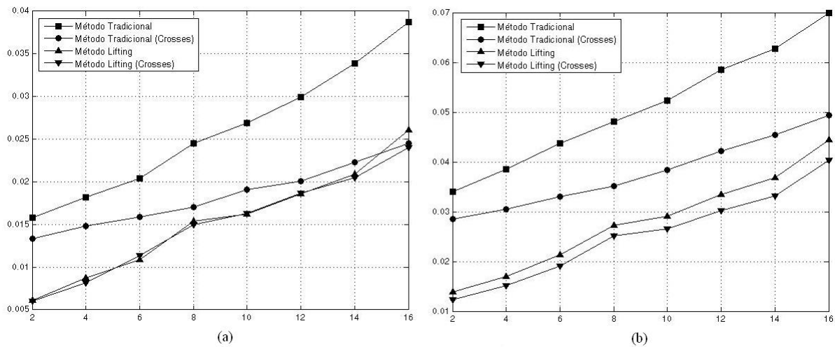
Figura 10.1: Comparação T_p \times n para wavelets de Daubechies para a imagem Crosses : (a) Decomposição; (b) Decomposição e Reconstrução.
