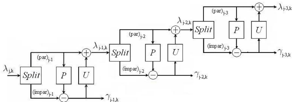
Figura 8.4: TWD em 3 níveis ( j=3 ) [82].
