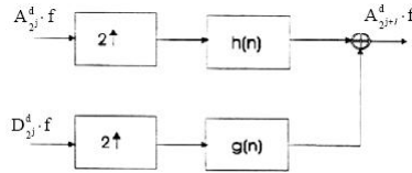
Figura 5.4: Diagrama em blocos do esquema de reconstrução da representação wavelet [24].
