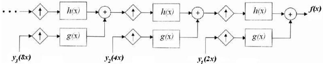
Figura 4.4: Algoritmo de Mallat (TWD inversa) [24].
