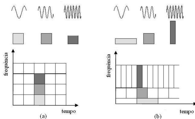
Figura 3.1: Tipos de transformadas (a) Transformada de Fourier Janelada (b) Transformada Wavelet [43].
