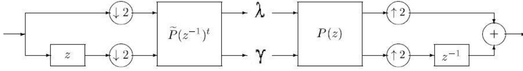
Figura 8.7: Representação polifásica da transformada wavelet [1].
