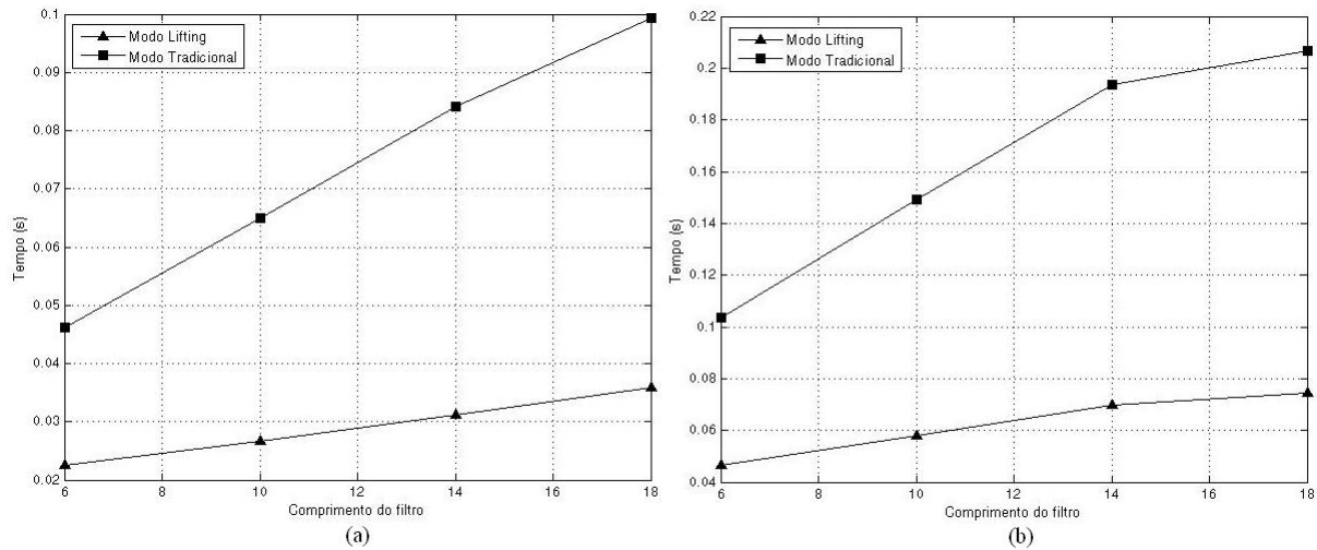
Figura 9.12: Comparação T_p \times n para wavelets Biortogonais (ordem2) utilizando ferramenta compilada: (a) Decomposição; (b) Decomposição e reconstrução.
