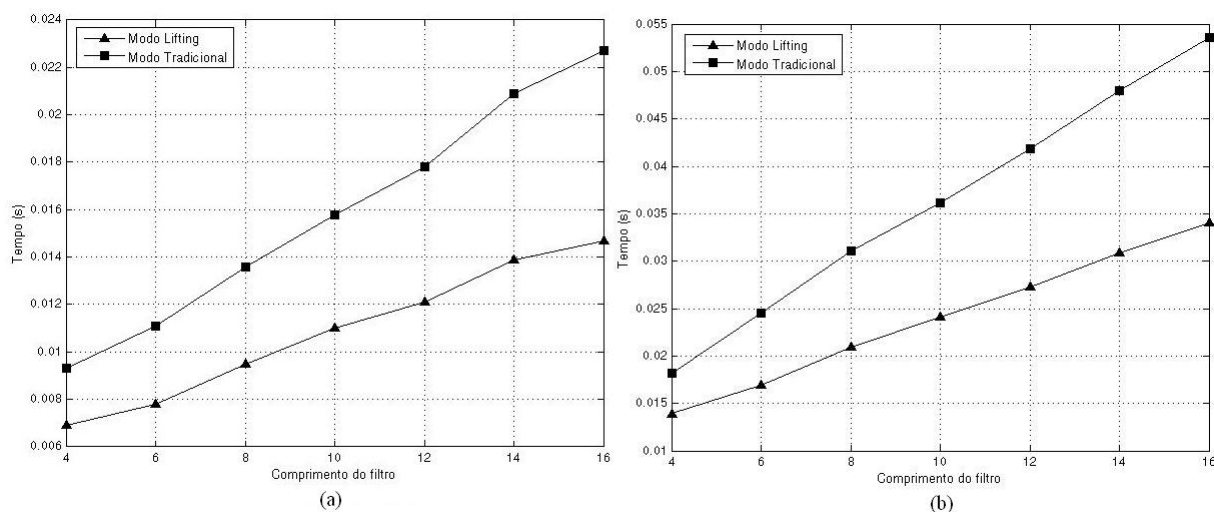
Figura 9.4: Comparação T_p \times n para wavelets Symlets utilizando ferramenta compilada: (a) Decomposição; (b) Decomposição e reconstrução.
