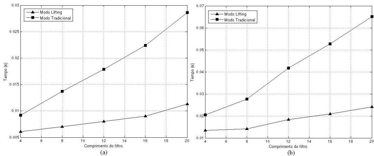
Figura 9.7: Comparação T_p \times n para wavelets Biortogonais (ordem 3) utilizando ferramenta compilada: (a) Decomposição; (b) Decomposição e reconstrução.
