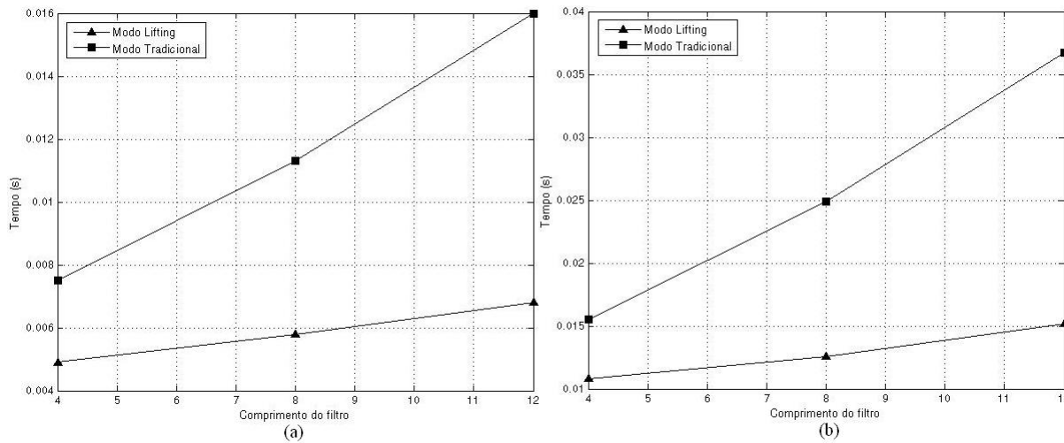
Figura 9.5: Comparação T_p \times n para wavelets Biortogonais (ordem 1) utilizando ferramenta compilada: (a) Decomposição; (b) Decomposição e reconstrução.
