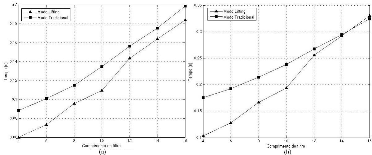
Figura 9.22: Comparação T_p \times n para wavelets Symlets utilizando ferramenta interpretada: (a) Decomposição; (b) Decomposição e Reconstrução.
