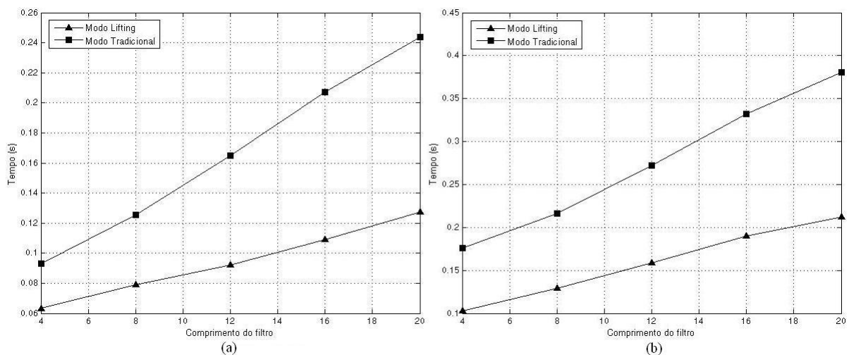
Figura 9.25: Comparação T_p \times n para wavelets Biortogonais (ordem3) utilizando ferramenta interpretada: (a) Decomposição; (b) Decomposição e reconstrução.
