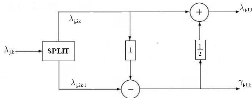
Figura 8.3: Implementação do esquema lifting da transformada de Haar [81].
