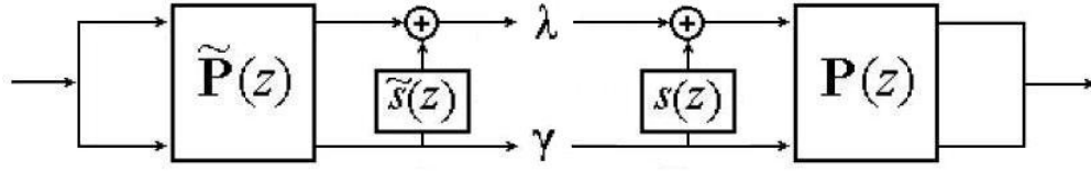
Figura 8.8: Esquema primal lifting .
