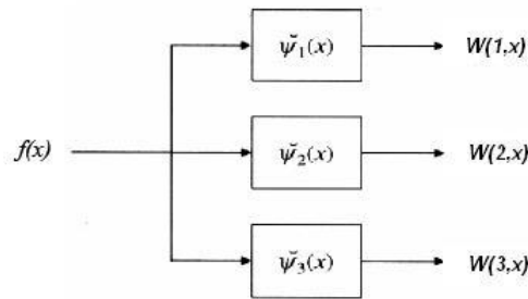
Figura 3.2: Interpretação da TWC por analogia de um banco de filtros [3].
