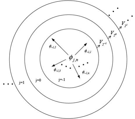
Figura 5.1: Esquema ilustrativo da relação entre \phi_{j,n}(x) e V_{2^j} para j \in [-1, 1] [3].
