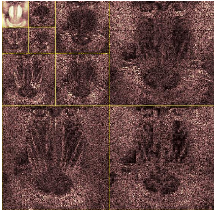
Figura 5.8: Representação wavelet ortogonal bidimensional para j=3 .
