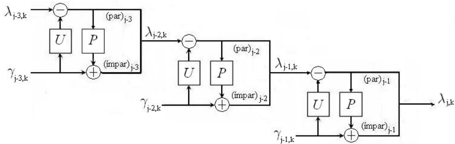
Figura 8.5: Reconstrução do sinal em 3 níveis [82].
