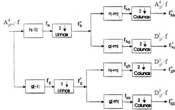
Figura 5.5: Diagrama de blocos de um estágio de decomposição wavelet de uma imagem [24].
