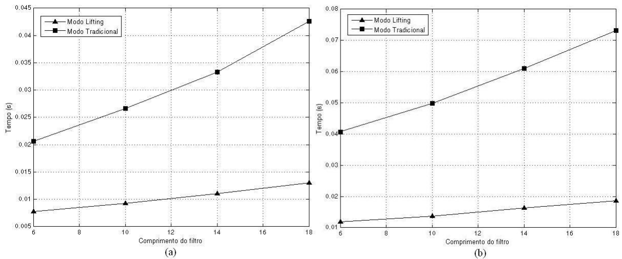
Figura 9.18: Comparação T_p \times n para wavelets Biortogonais (ordem2) utilizando ferramenta interpretada: (a) Decomposição; (b) Decomposição e reconstrução.
