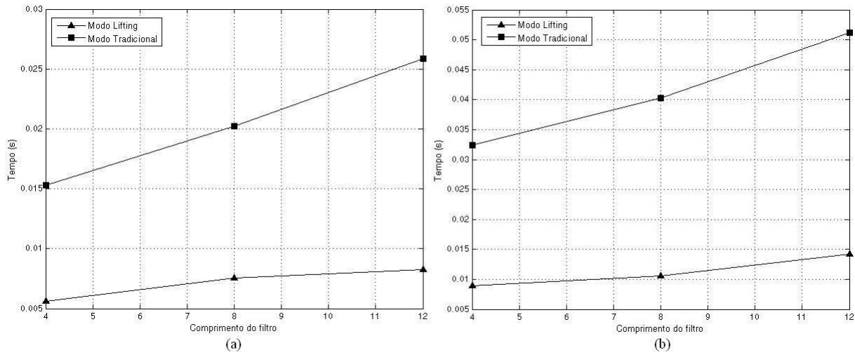
Figura 9.17: Comparação T_p \times n para wavelets Biortogonais (ordem1) utilizando ferramenta interpretada: (a) Decomposição; (b) Decomposição e reconstrução.
