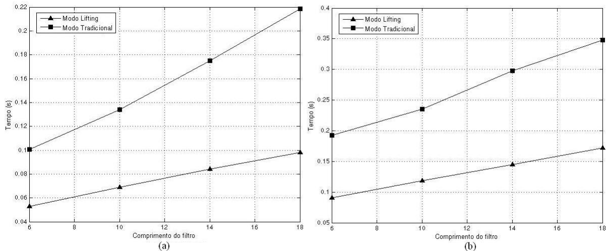
Figura 9.24: Comparação T_p x n para wavelets Biortogonais (ordem2) utilizando ferramenta interpretada: (a) Decomposição; (b) Decomposição e reconstrução.
