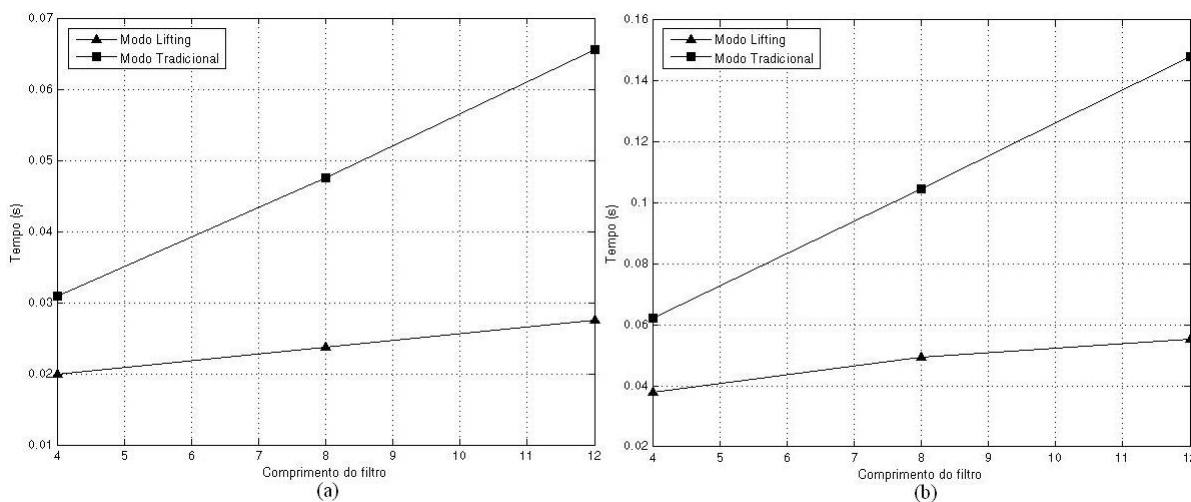
Figura 9.11: Comparação T_p \times n para wavelets Biortogonais (ordem1) utilizando ferramenta compilada: (a) Decomposição; (b) Decomposição e reconstrução.
