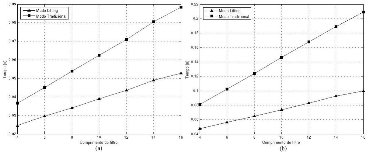
Figura 9.10: Comparação T_p \times n para wavelets Symlets utilizando ferramenta compilada: (a) Decomposição; (b) Decomposição e reconstrução.
