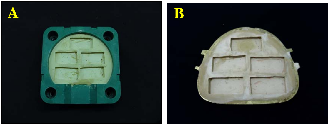
Figura 3. Moldes no gesso deixados pela matriz de cera na mufla plástica (A) e metálica (B).
