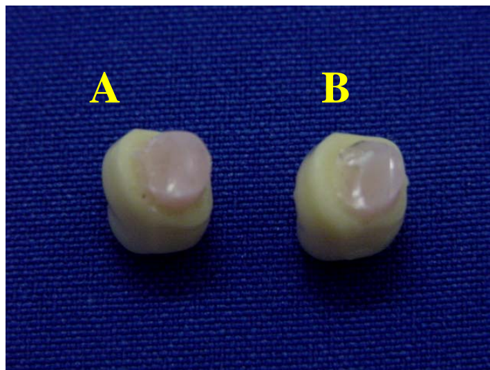
Figura 18. Tipos de falhas da união dente-resina: coesiva na resina (A) e mista (B).
