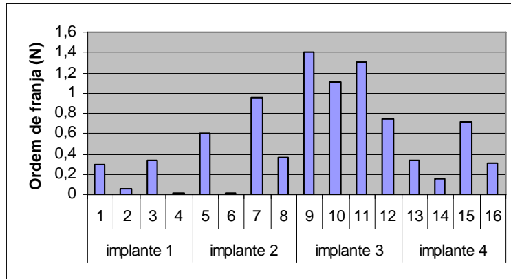
Figura 17: Valores de ordem de franja (N) para os pontos selecionados em cada implante para os pilares Ucla.
