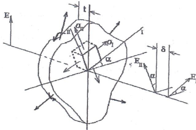
Figura 14- Retardação causada pelo estado das tensões ( \delta )
