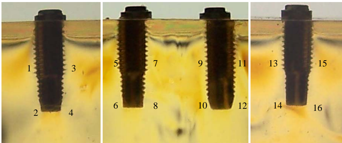
Figura 12- Áreas selecionadas ao redor de cada implante para a determinação da ordem de franjas inteiras (N).
