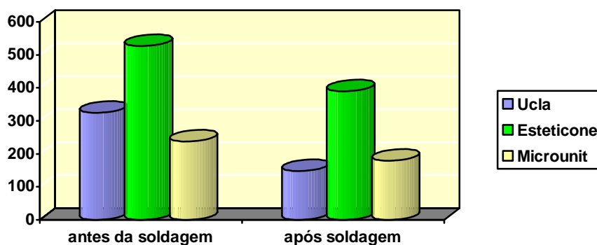
Figura 15: Ilustração gráfica da média em micrometros da desadaptação linear vertical para as interfaces avaliadas antes e após soldagem vertical a laser das estruturas.
