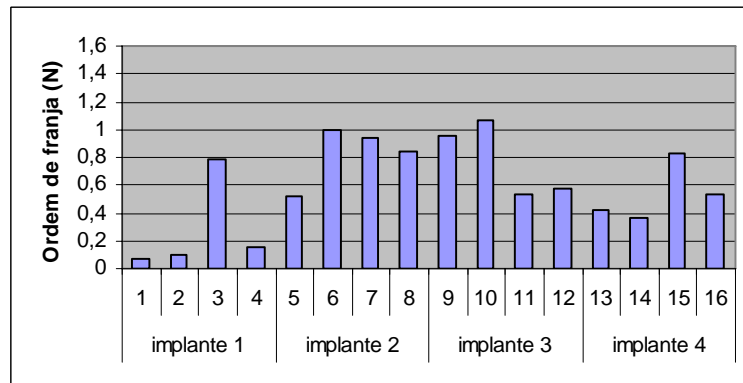
Figura 18: Valores de ordem de franja (N) para os pontos selecionados em cada implante para os pilares Esteticone.
