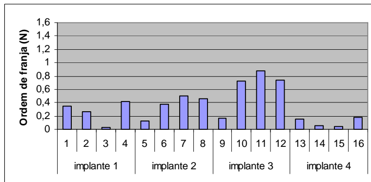
Figura 18: Valores de ordem de franja (N) para os pontos selecionados em cada implante para os pilares Esteticone.
