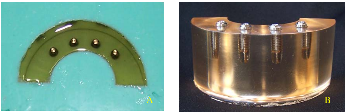
Figura 6: Resina Araldite vertida no interior do molde da matriz (A) e o respectivo modelo fotoelástico obtido após completa polimerização da mesma (B).
