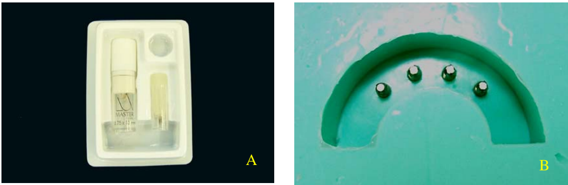
Figura 5: Implantes Master Screw (Conexão) utilizados (A) e sua adaptação nos respectivos transferentes do molde da matriz (B).
