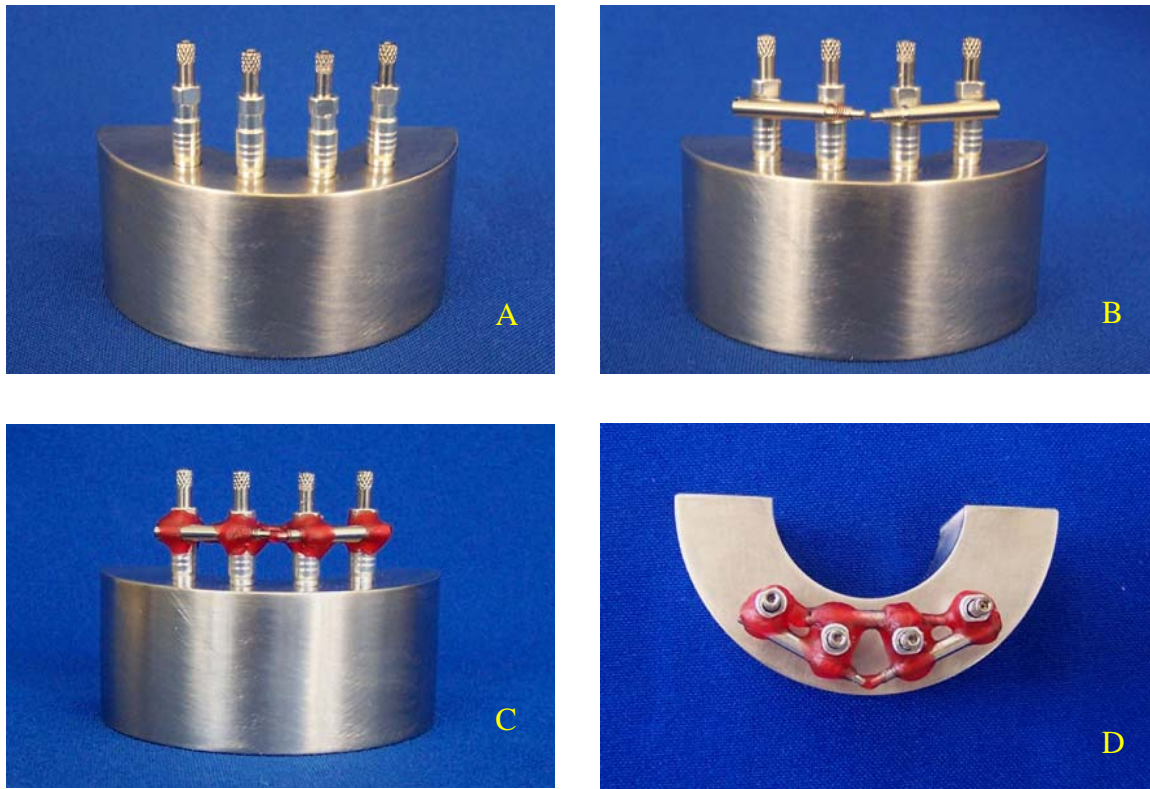
Figura 2: Transferentes de moldagem posicionados sobre os análogos de implantes (A), unidos entre si com pinos metálicos (B), e posteriormente revestidos com resina acrílica ativada quimicamente (C) e (D)
