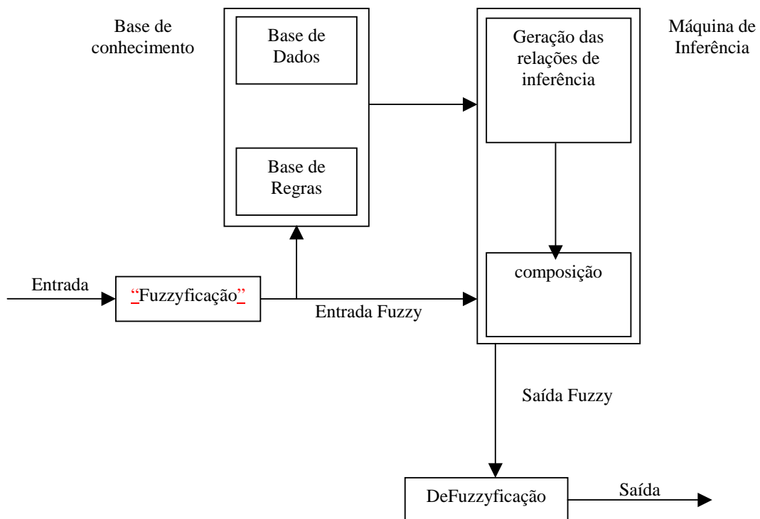
Figura 5 – Configuração de um controlador “Fuzzy” Fonte: Azevedo (1999)
