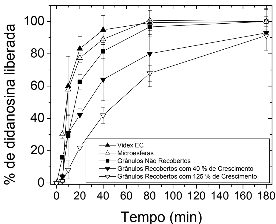
FIGURA 91. Liberação da didanosina em suco entérico simulado (pH = 7,40).
