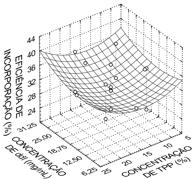
FIGURA 23. Superfície de resposta para a eficiência de incorporação em função das concentrações de quitosana e tripolifosfato de sódio (TPP).
