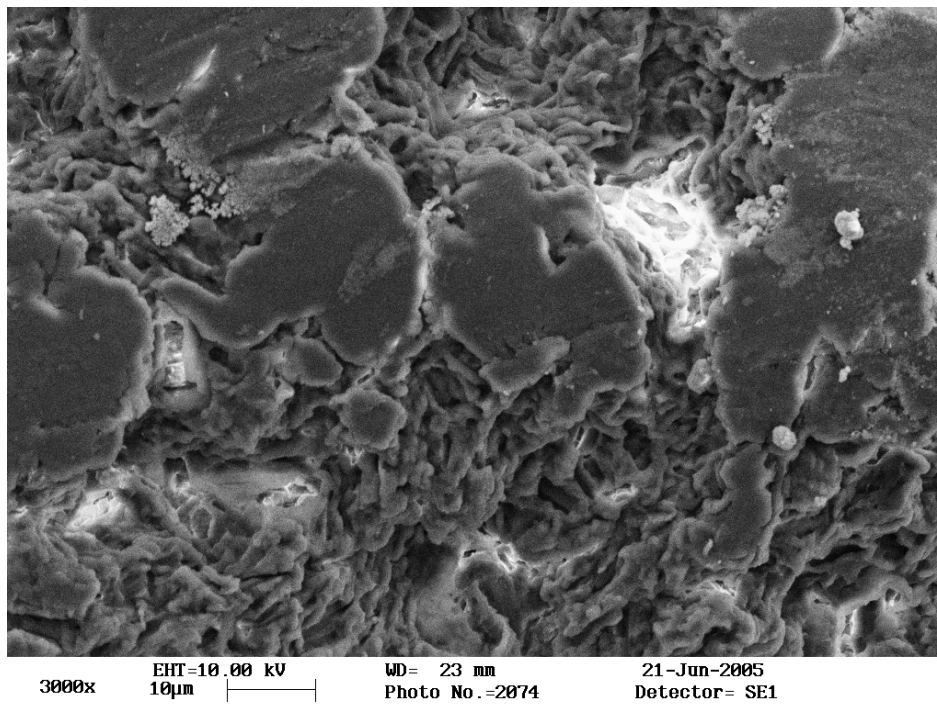
FIGURA 68. Micrografia da superfície dos grânulos contendo microesferas de quitosana, didanosina e 4,8 % de amido pré-gelificado após a liberação da ddi em suco entérico simulado com pancreatina.
