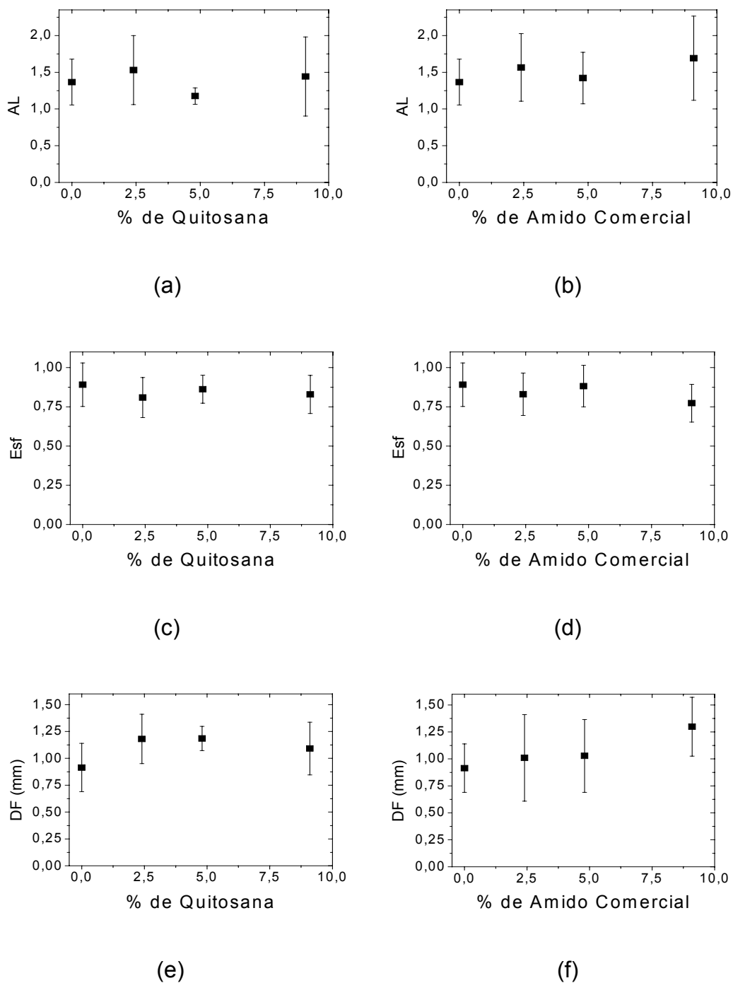
FIGURA 51. Variações dos parâmetros geométricos em função da concentração dos excipientes quitosana e amido comercial. (a) e (b) Alongamento-AL; (c) e (d) Esfericidade-Esf; (e) e (f) Diâmetro de Feret-DF.
