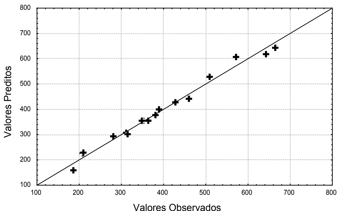
FIGURA 26. Valores preditos versus valores observados experimentalmente para o carregamento.
