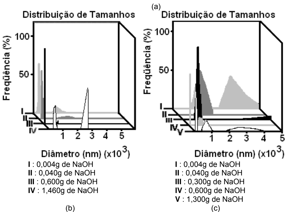
FIGURA 9. Influência do hidróxido de sódio (NaOH) no diâmetro médio e distribuição de tamanhos das partículas: (a) diâmetro médio; (b) distribuição de tamanhos para 0,10 % (m/v) de NaOH; (c) distribuição de tamanhos para 1,00 % (m/v) de NaOH.
