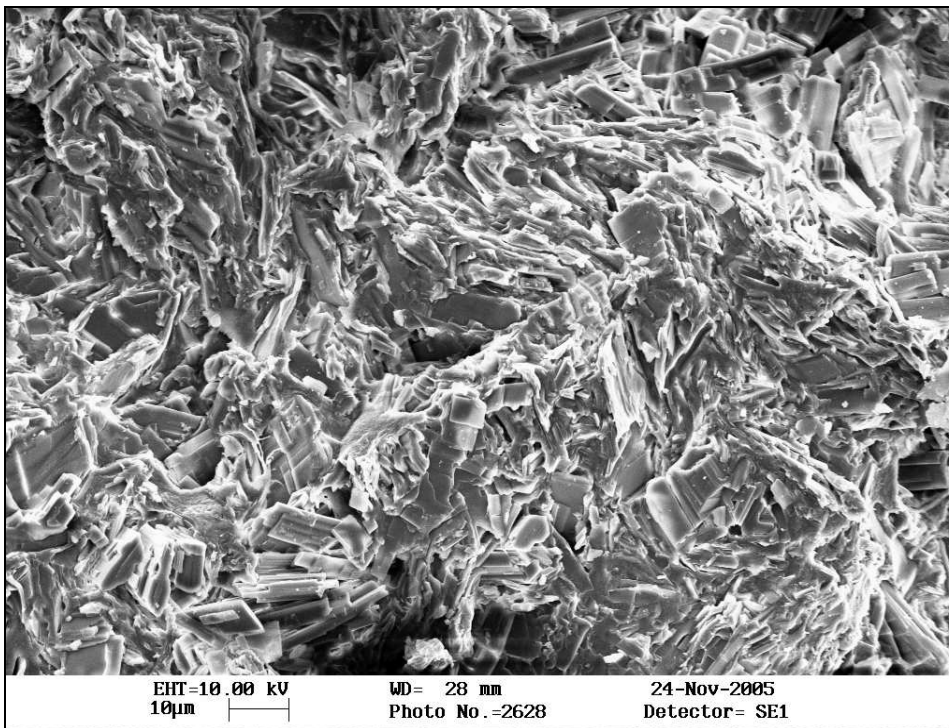
FIGURA 66. Micrografia da estrutura interna do grânulo não recoberto (aumentada 2.000 vezes).
