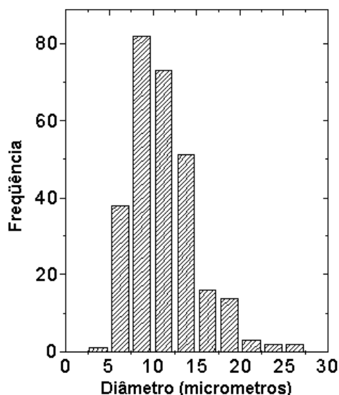
FIGURA 36. Histograma da distribuição de diâmetros das partículas obtido a partir da imagem de microscopia ótica, correspondente ao experimento 5 (25,00 mg de didanosina/ \text{cm}^3 / 2,00 % (m/v) de quitosana / 10,00 % de tripolifosfato de sódio).
