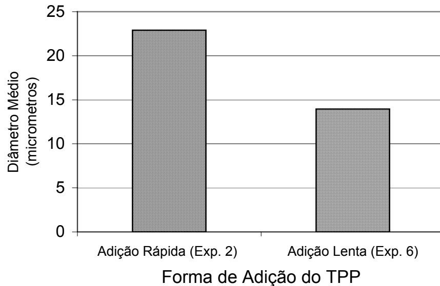
FIGURA 15. Comparação entre os diâmetros médios das partículas para duas formas de adição de uma mesma quantidade de tripolifosfato de sódio (TPP).
