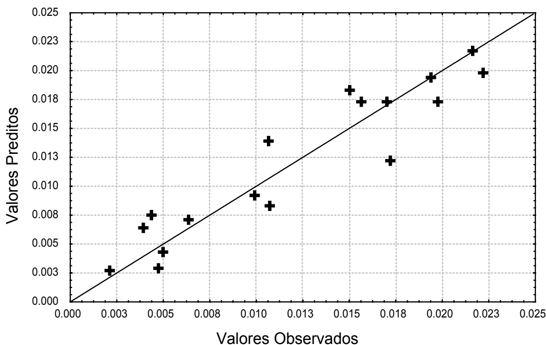
FIGURA 31. Valores previstos pelo modelo versus valores observados experimentalmente para o coeficiente de permeabilidade.
