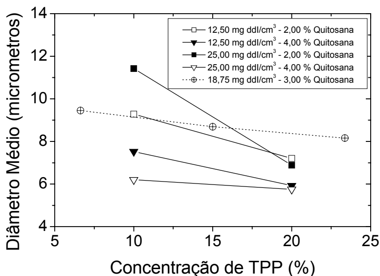
FIGURA 38. Variação do diâmetro das partículas em função da concentração de tripolisfosfato de sódio (TPP) para diferentes concentrações de quitosana e didanosina.
