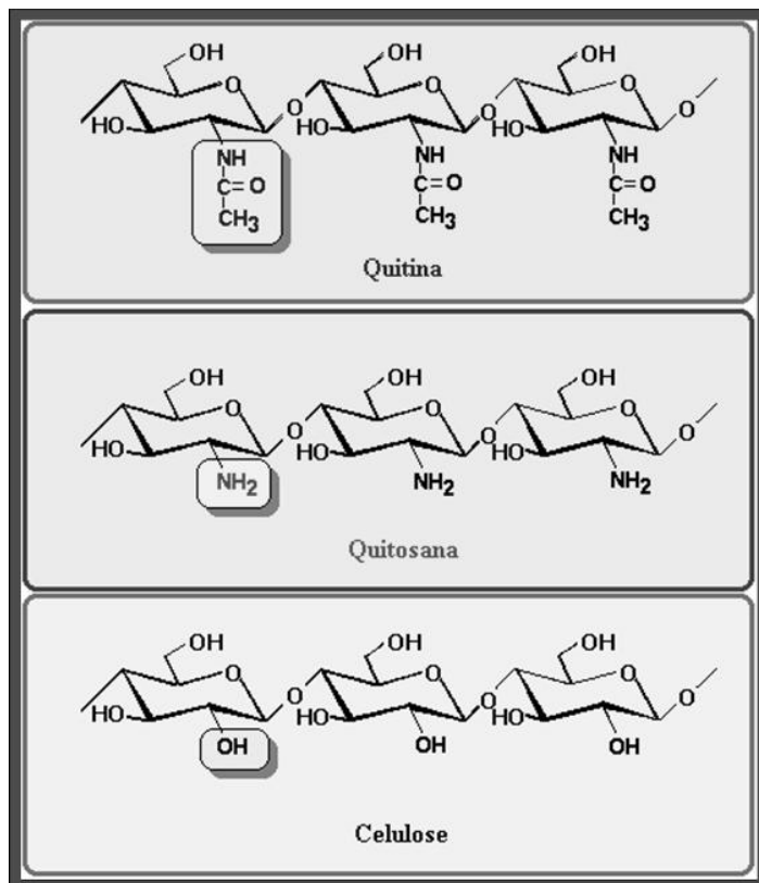
FIGURA 6. Estrutura da quitina, quitosana e celulose (adaptação do site http://user.chol.com/~chitin/cellulose.gif , acessado em 10/02/2006).
