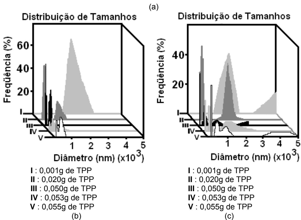
FIGURA 10. Influência do tripolifosfato de sódio (TPP) no diâmetro médio das partículas: (a) diâmetro médio; (b) distribuição de tamanhos para 0,10 % (m/v) de TPP; (c) distribuição de tamanhos para 1,00 % (m/v) de TPP.
