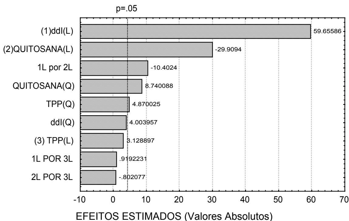
FIGURA 25. Gráfico de Pareto para o carregamento, com 95 % de intervalo de confiança, obtido para o planejamento fatorial.
