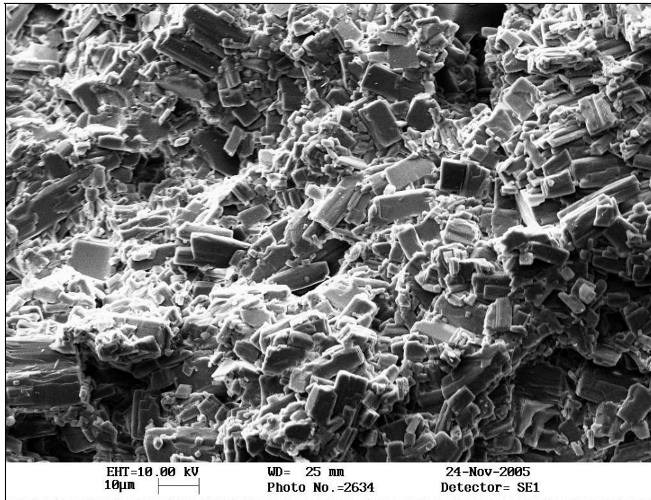
FIGURA 65. Micrografia da estrutura interna do grânulo de Videx® EC (aumentada 2.000 vezes).
