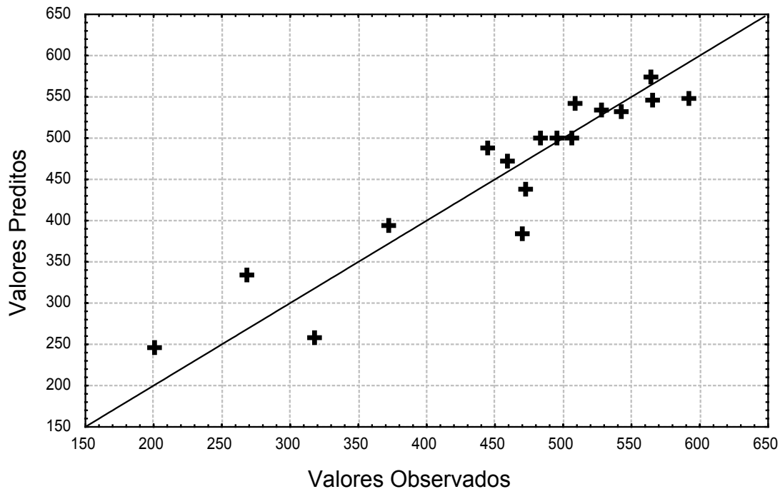
FIGURA 42. Valores previstos pelo modelo versus valores observados experimentalmente para o grau de intumescimento.
