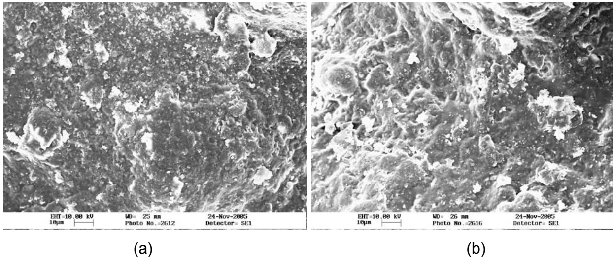
FIGURA 89. Micrografia da superfície dos grânulos recobertos: (a) 50 % de crescimento; (b) 125 % de crescimento (aumentadas 2.000 vezes).
