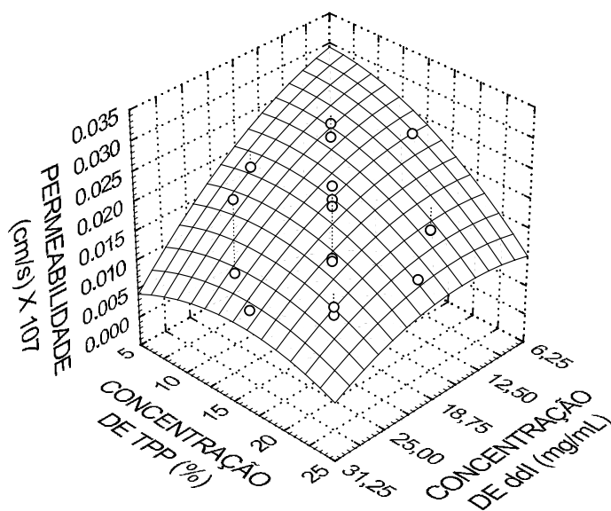
FIGURA 33. Superfície de resposta do coeficiente de permeabilidade em função das concentrações de quitosana e tripolisfosfato de sódio (TPP).
