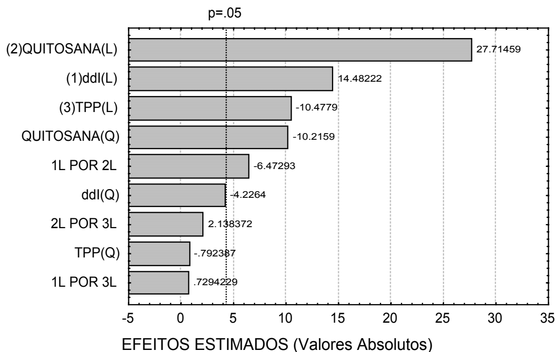
FIGURA 41. Gráfico de Pareto, com intervalo de confiança de 95 %, para o modelo quadrático do grau de intumescimento obtido do planejamento composto central.
