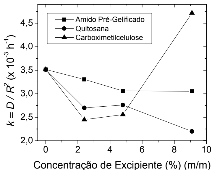
FIGURA 60. Variação da constante k do modelo difusivo em função da concentração de excipientes nos grânulos.
