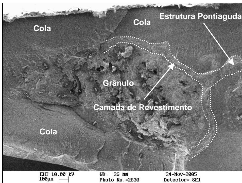
FIGURA 90. Micrografia da fratura de um grânulo com 125 % de revestimento (aumentada 200 vezes).
