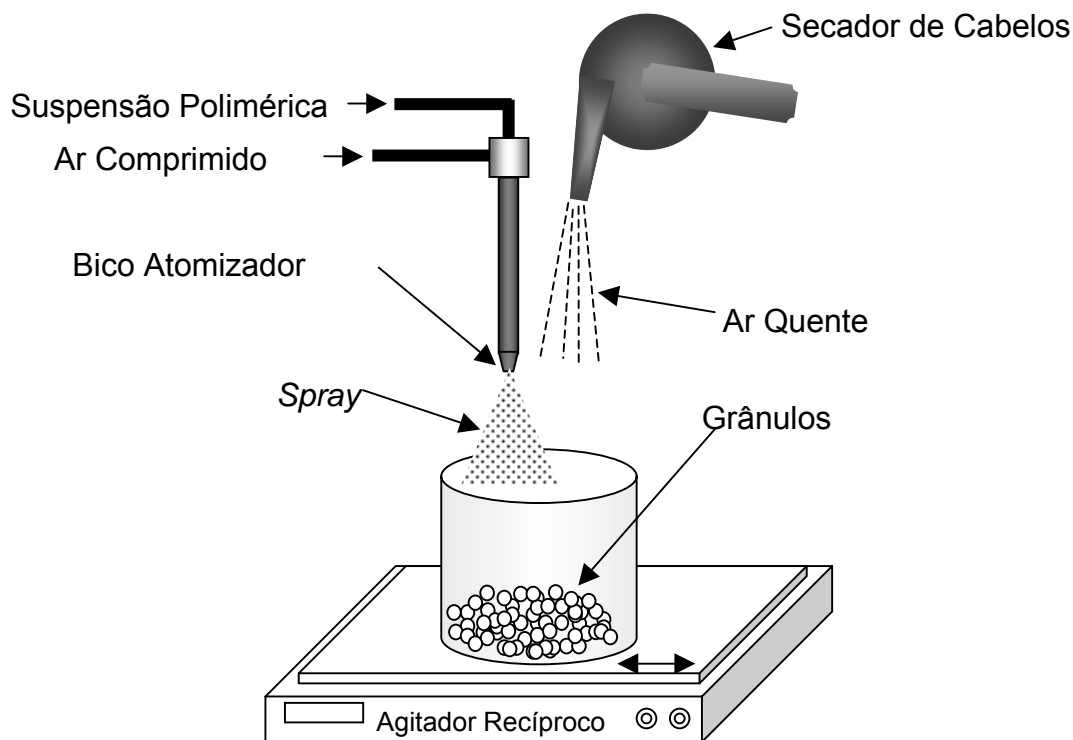
FIGURA 83. Sistema artesanal para o revestimento dos grânulos.
