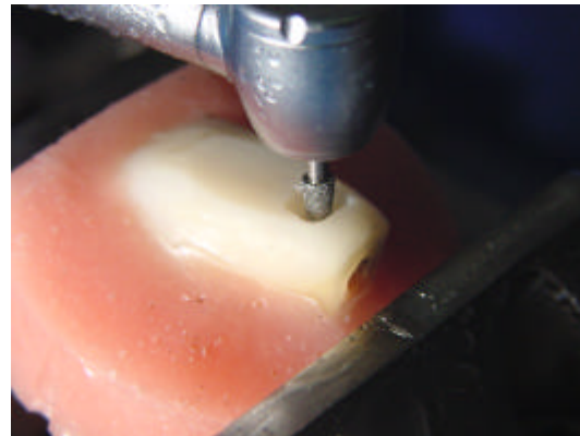
Figura 11 – Preparo cavitário pronto, com corpo-de-prova ainda fixado na máquina.
