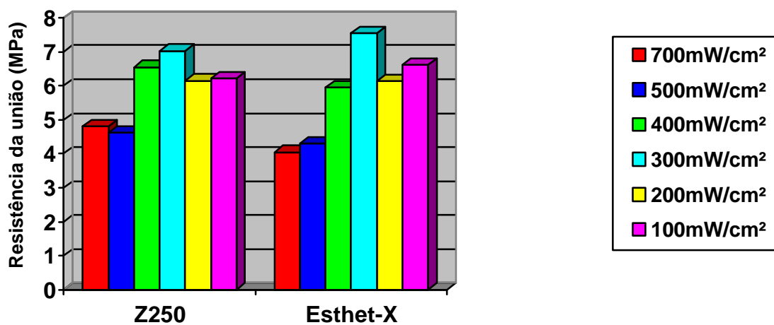
Figura 23 – Ilustração gráfica das médias de resistência de união (MPa) para interação entre as combinações tempo X intensidade de luz, para os dois compósitos, usando o aparelho de lâmpada halógena.
