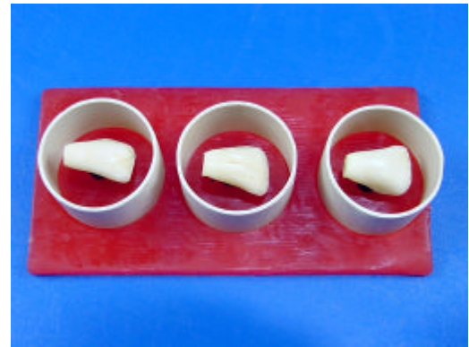
Figura 7 – Tubos de PVC sobre a base de cera.
