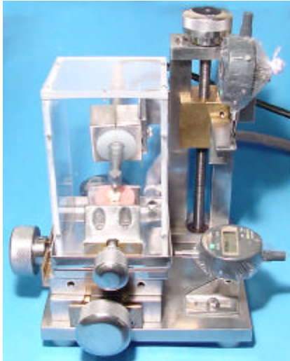
Figura 10 – Máquina específica para confecção de preparos cavitários padronizados.
