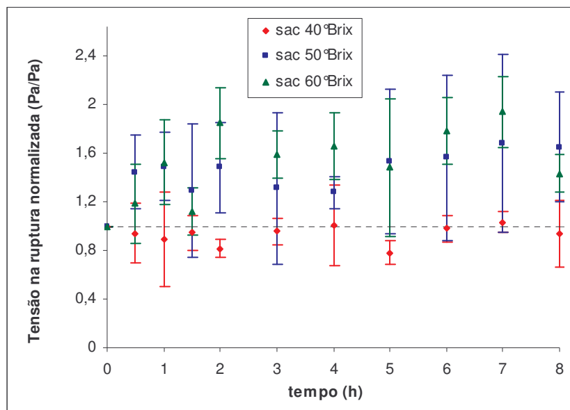
Figura 4.11 – Variação da Tensão na Ruptura durante 8 horas de processo para os ensaios realizados com sacarose a 30°C
