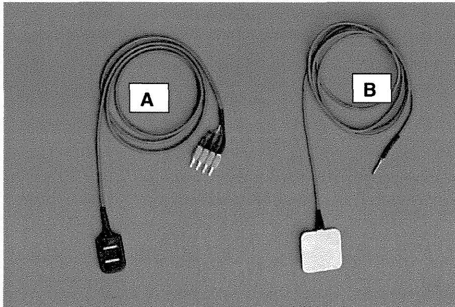
Figura 3. Eletrodo ativo diferencial simples de superfície ( Lynx Tecnologia Eletrônica Ltda ) – (A) e eletrodo terra (B).
