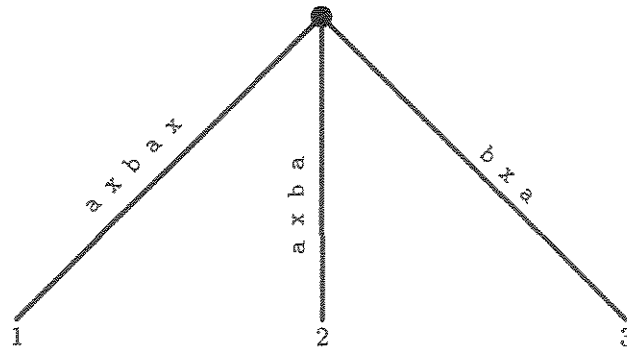
Figura 3.3: Árvore de Sufixos para a seqüência xabxa (sem o símbolo especial).
