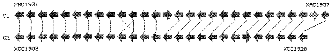
Figura 5.14: Visualização gráfica de uma RO encontrada na comparação das Xanthomonas . Os candidatos a genes falsos são aqueles de Xac que não possuem matches na região.
