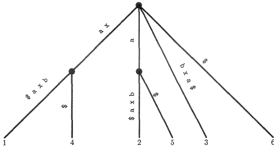
Figura 3.2: Árvore de Sufixos para a seqüência xabxa\$
