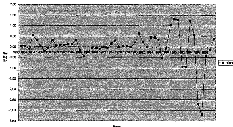
Primeira Diferença do Ln dos Preços Relativos
