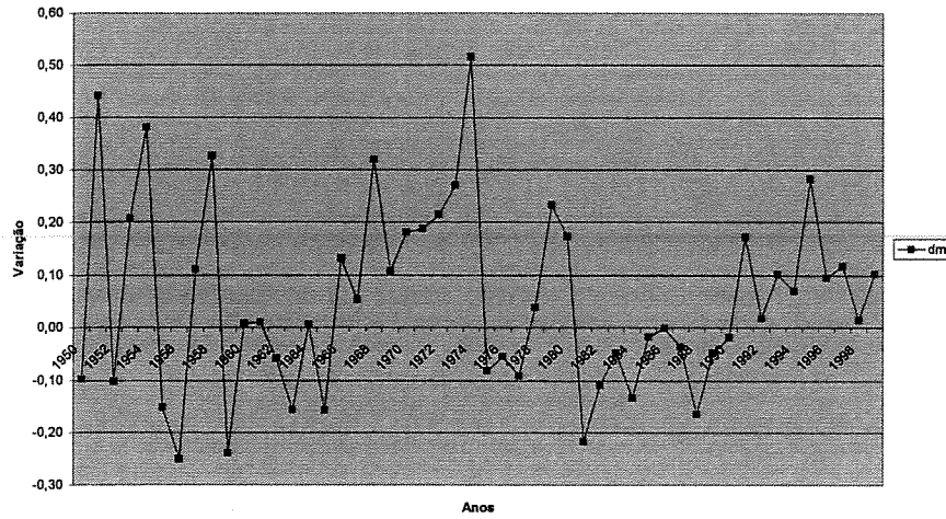
Primeira Diferença do Ln das Importações
