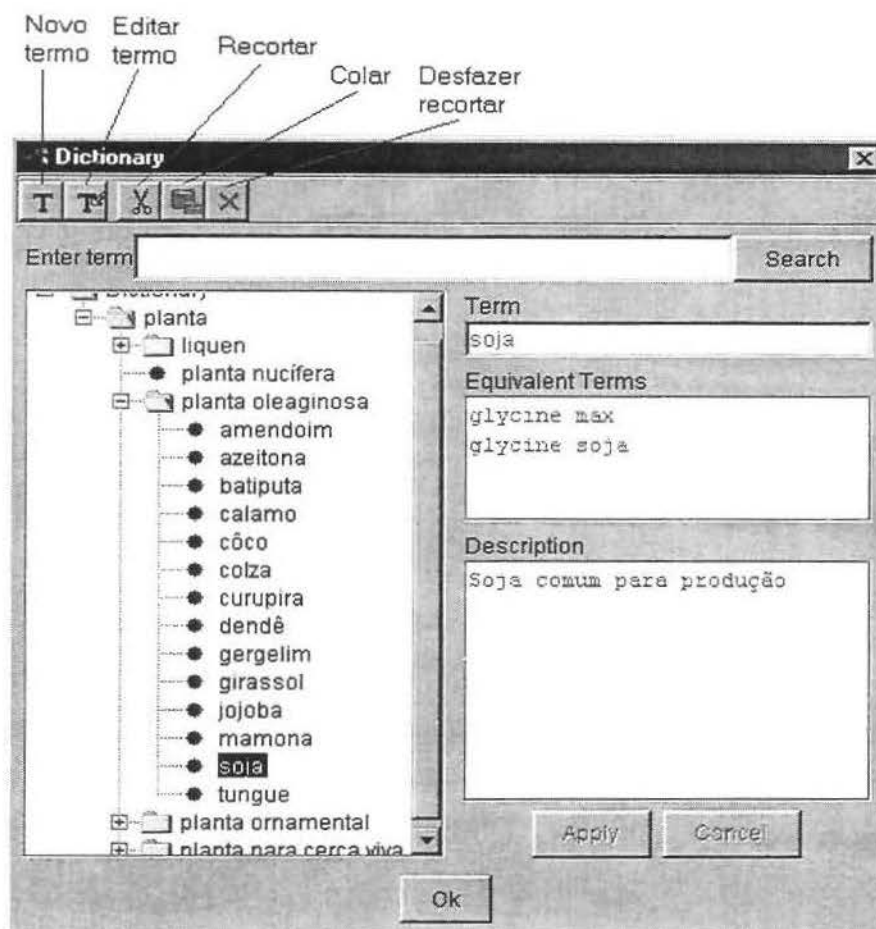
Figura 5.6: Janela para manipulação de termos do dicionário.
