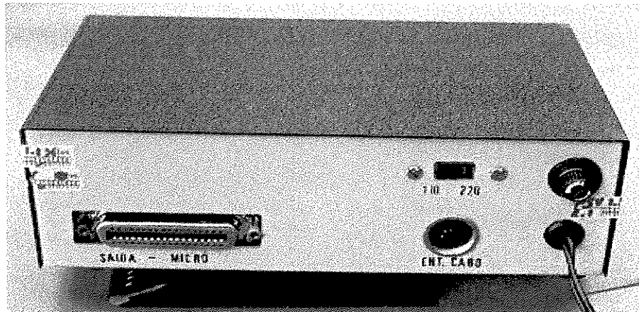
Foto 5. Vista posterior da Interface
