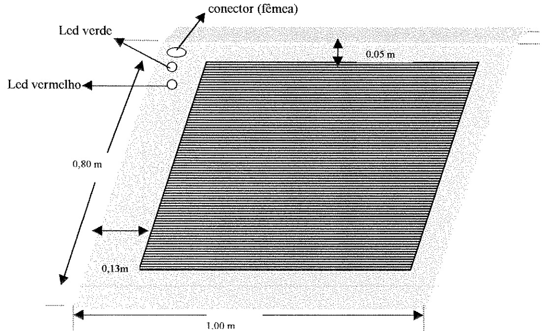
Figura 2: Representação esquemática da Plataforma PSV-20, suas dimensões e conexões.
