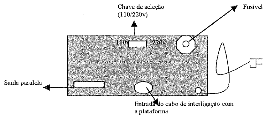
Figura 3 (B): vista posterior da interface
