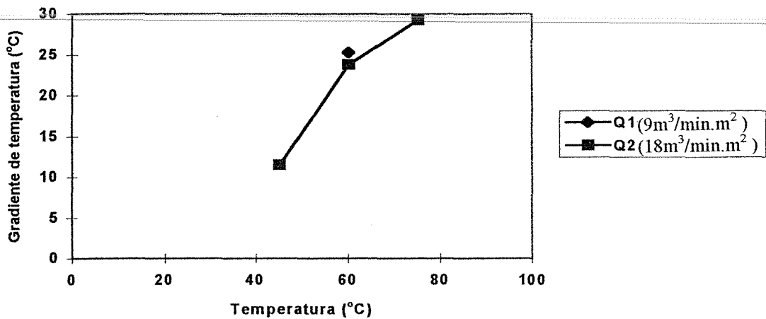
Figura 15 - Gradiente de temperatura no final da secagem do grão de sorgo com teor de umidade inicial de aproximadamente 21,0%.
