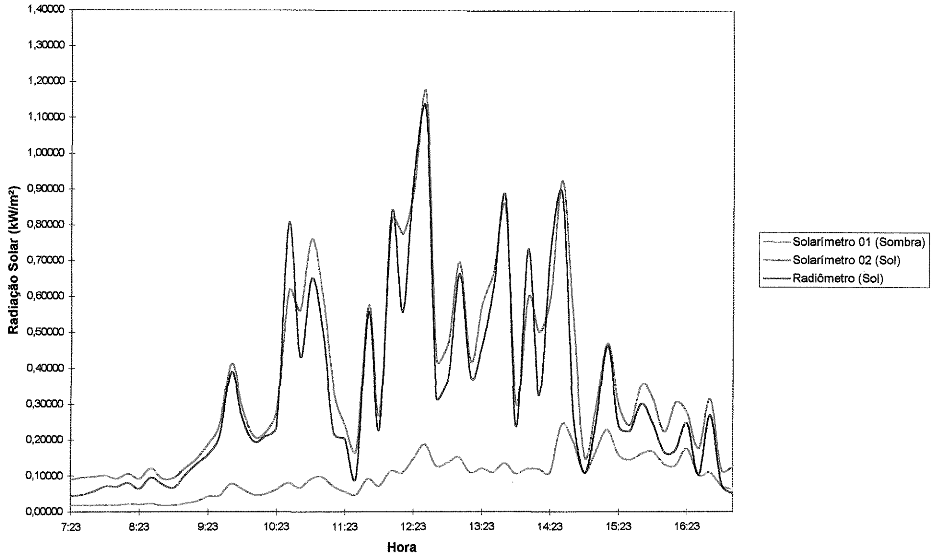
FIGURA 42 - Radiação solar (Magnólia) 19/março/1998.
