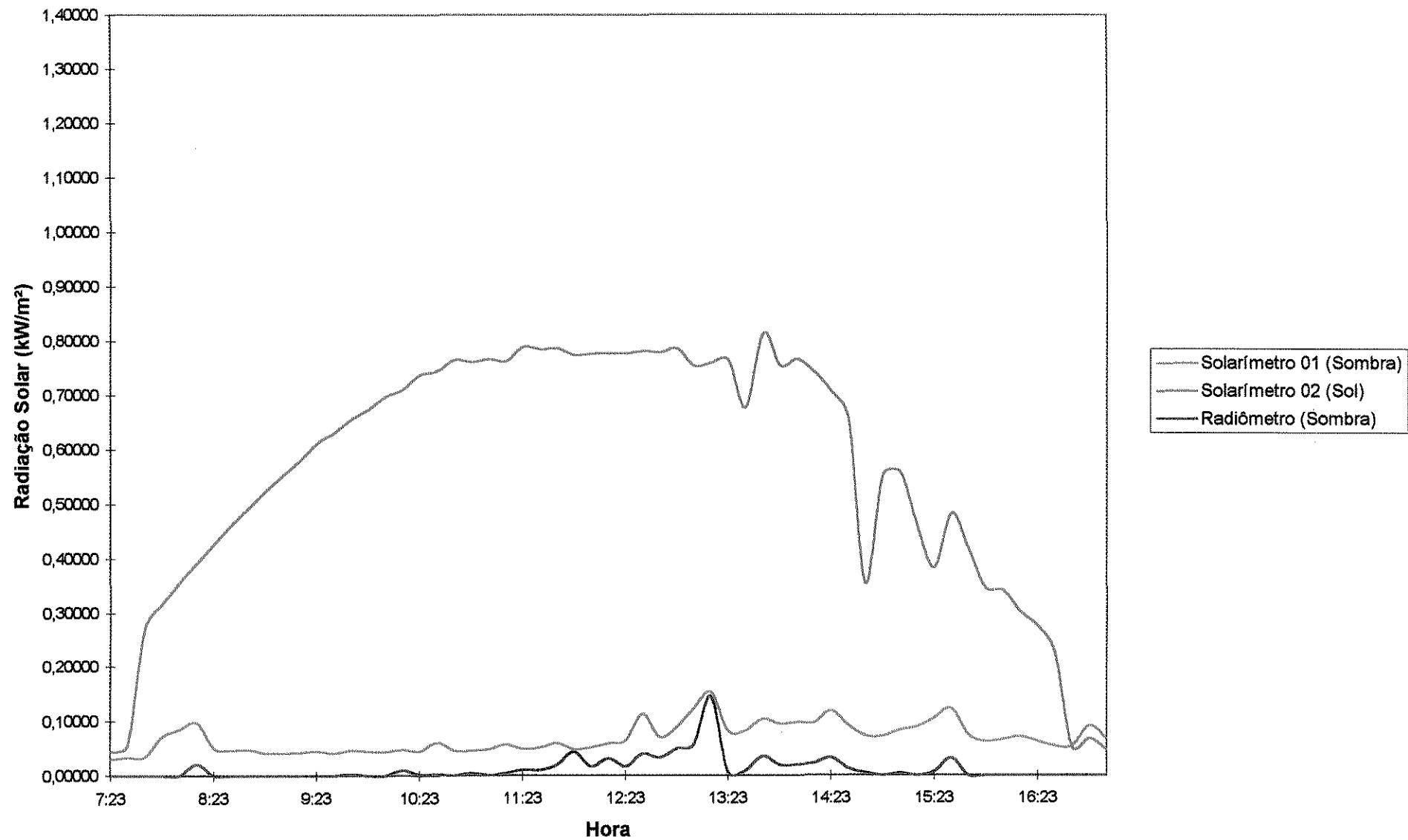
FIGURA 48 - Radiação solar (Sibipiruna) 21/abril/1998.
