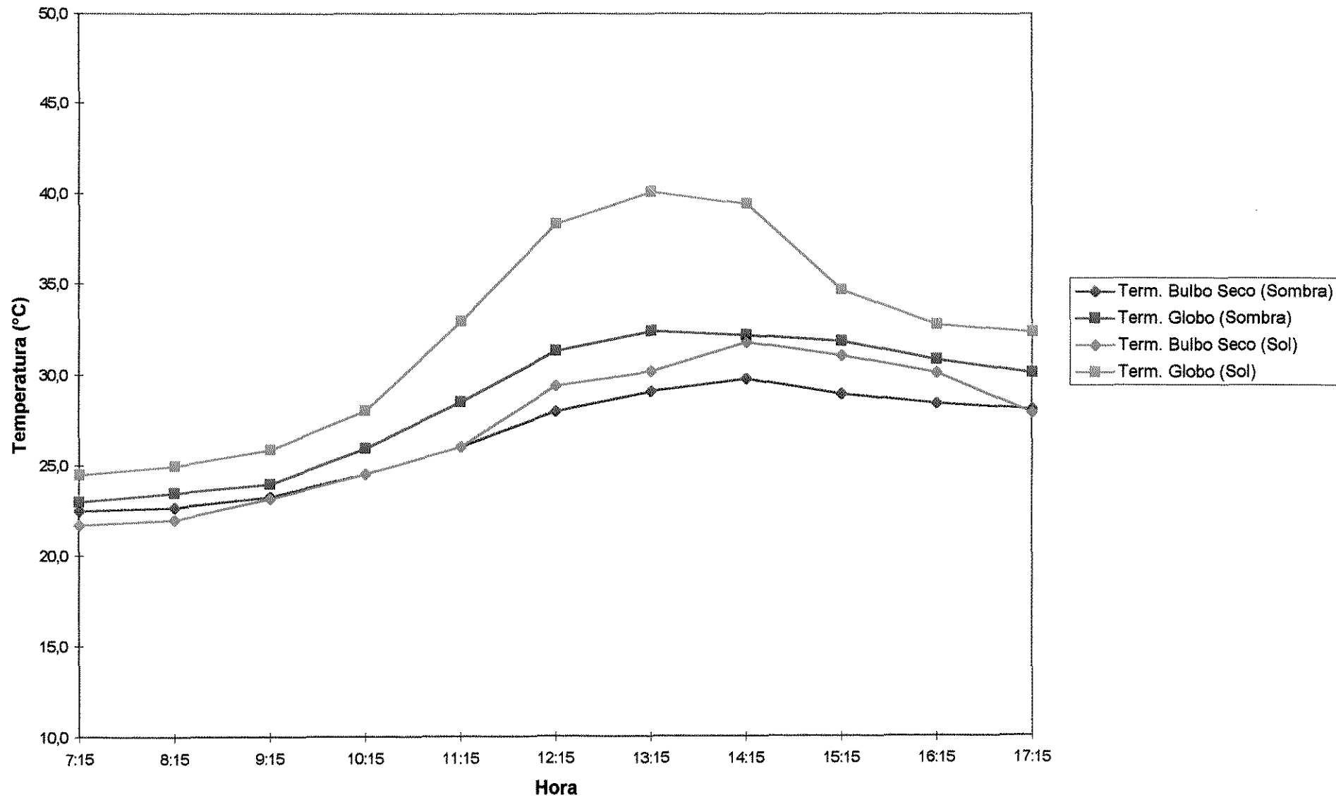
FIGURA 43 - Temperaturas (Magnólia) 19/março/1998.
