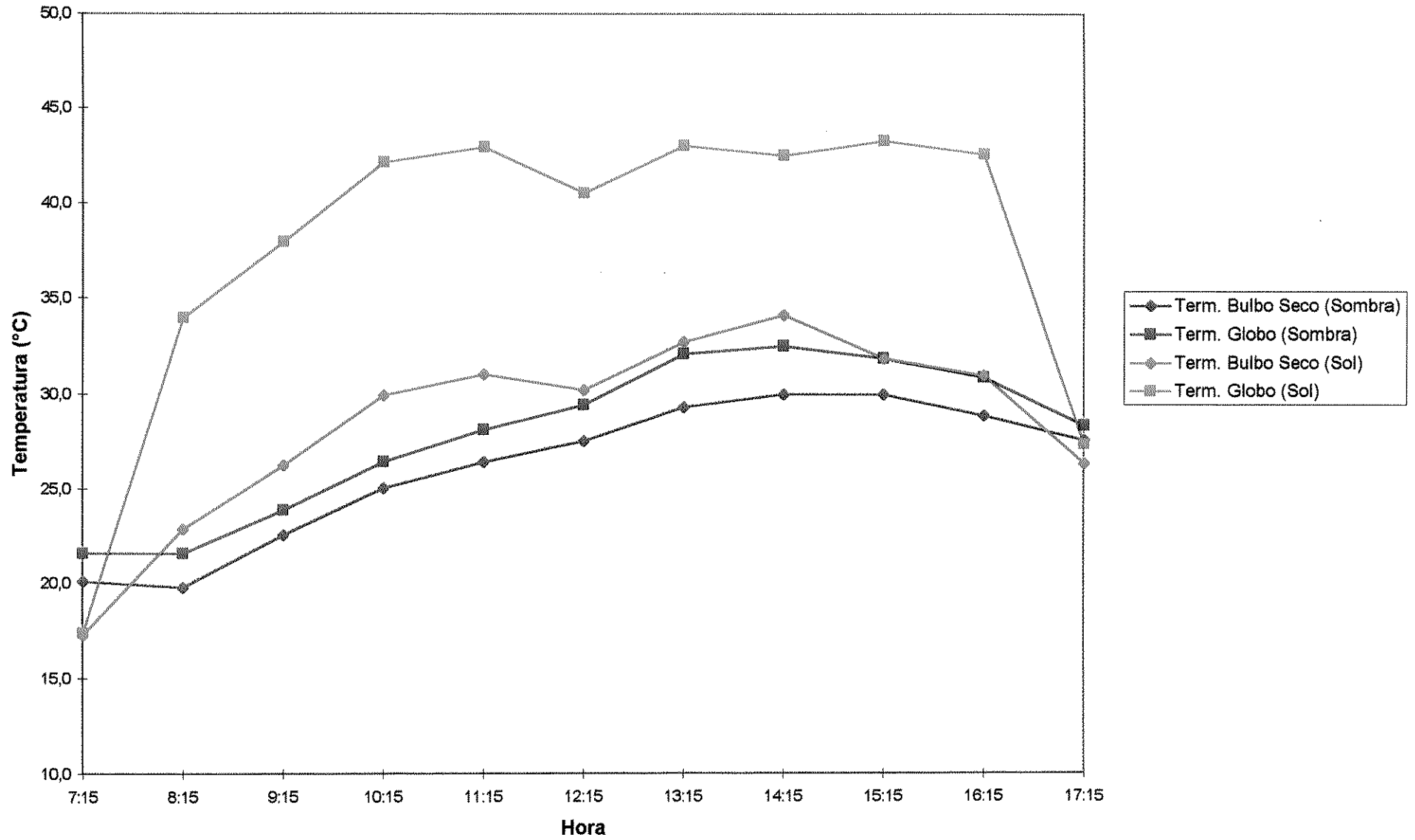
FIGURA 49 - Temperaturas (Sibipiruna) 21/abril/1998.
