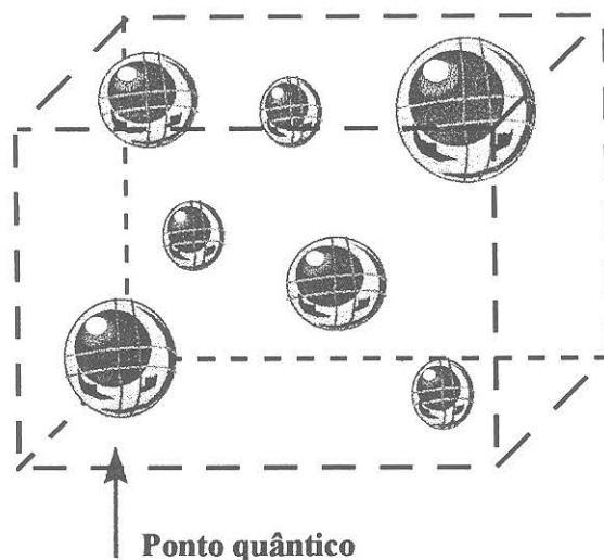
Figura 1-1: Nanocristais semicondutores (pontos quânticos) destacados pela seta, embebidos em uma matriz vítrea (modelo esquemático).
