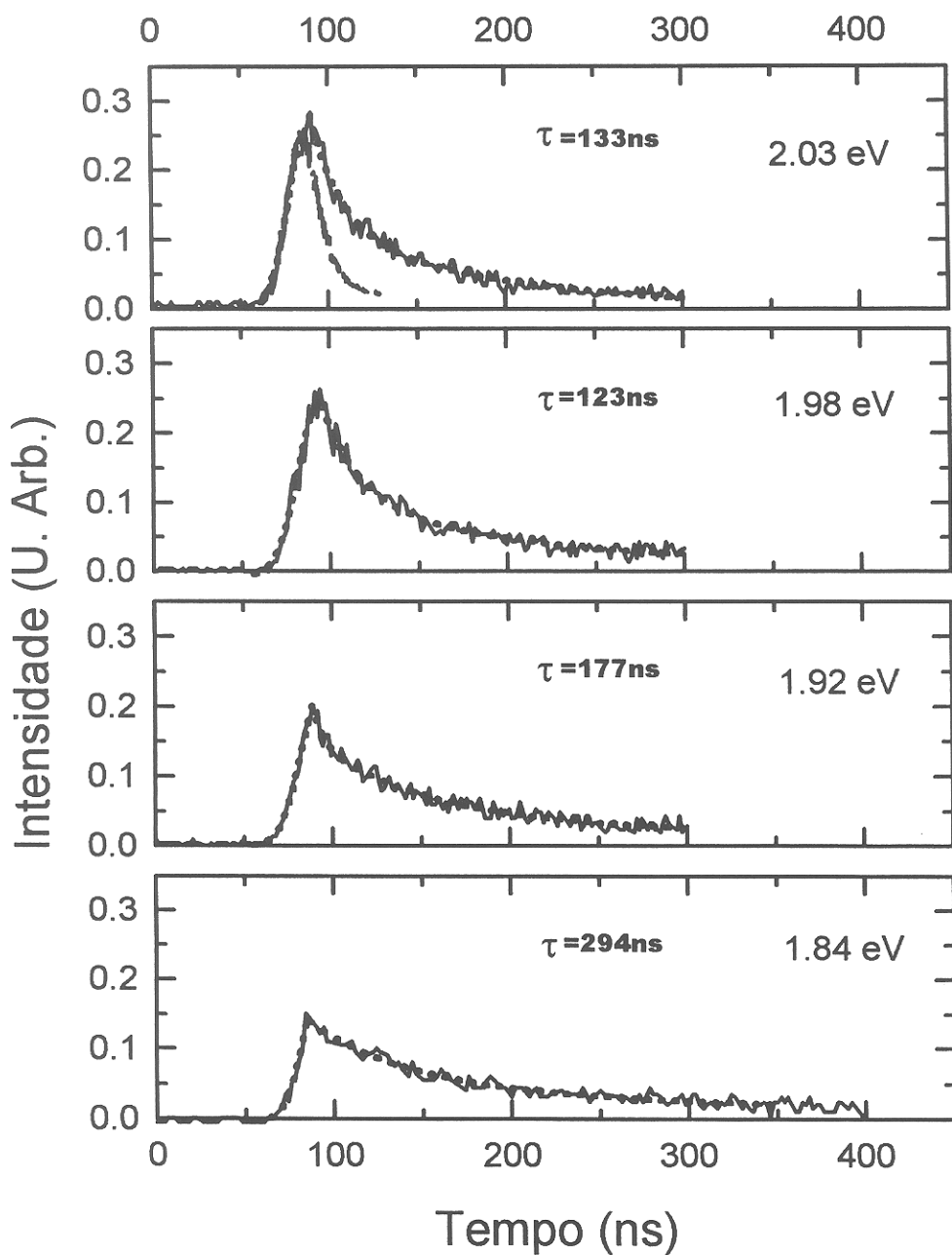
Figura 4-11: Fotoluminescência resolvida no tempo para a amostra VDS39-60h: 660min, a 20K. As curvas pontilhadas representam a convolução feita para obter o tempo do decaimento. A curva tracejada no primeiro box mostra a resolução do sistema.
