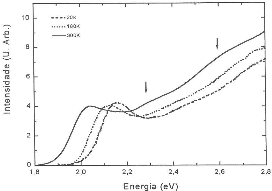
Figura 3-2: Medidas do espectro de absorção da amostra VCS39-60h: 660min, às temperaturas de 20 K (curva tracejada), 180 K (curva pontilhada) e 300 K (curva cheia).
