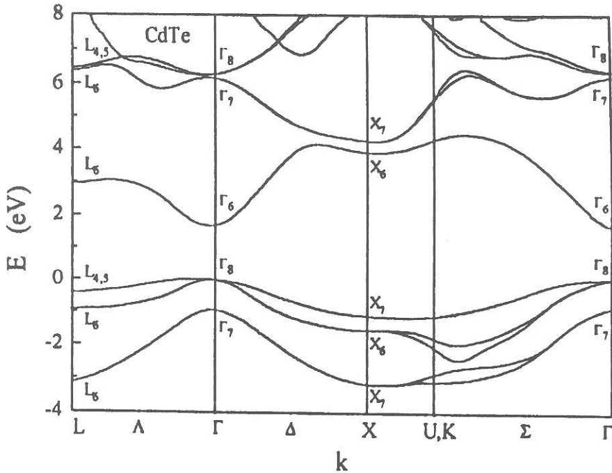
Figura 2-2: Diagrama de bandas do CdTe.
