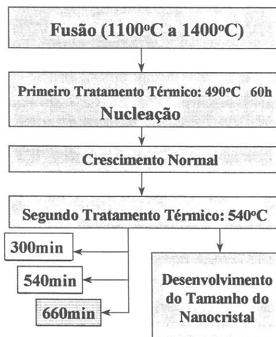
Figura 2-1: Etapas da formação dos vidros dopados com semicondutor
