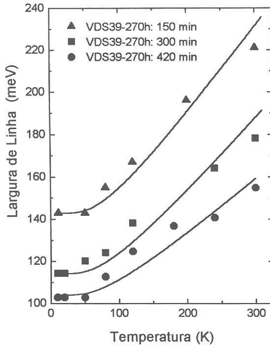
Figura 3-5: Comportamento da largura de linha total da amostra VDS39-270h: 420min, com a temperatura.
