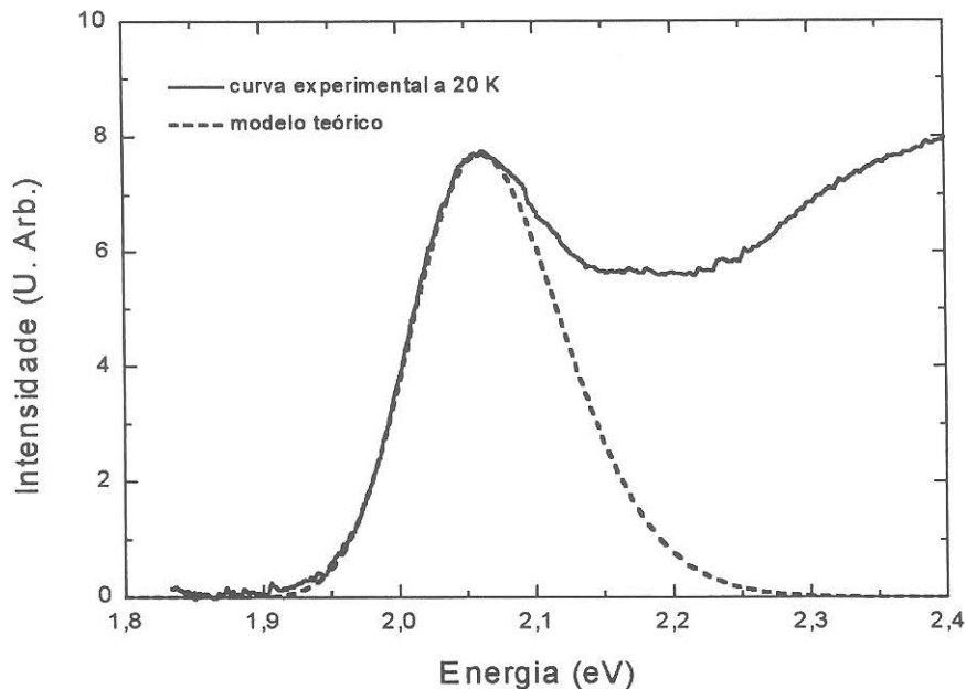
Figura 3-3: Medida de absorção para a amostra VDS39-270h: 420 min, realizada a 120 K (curva cheia) e o modelo teórico aplicado para o primeiro pico (curva tracejada).
