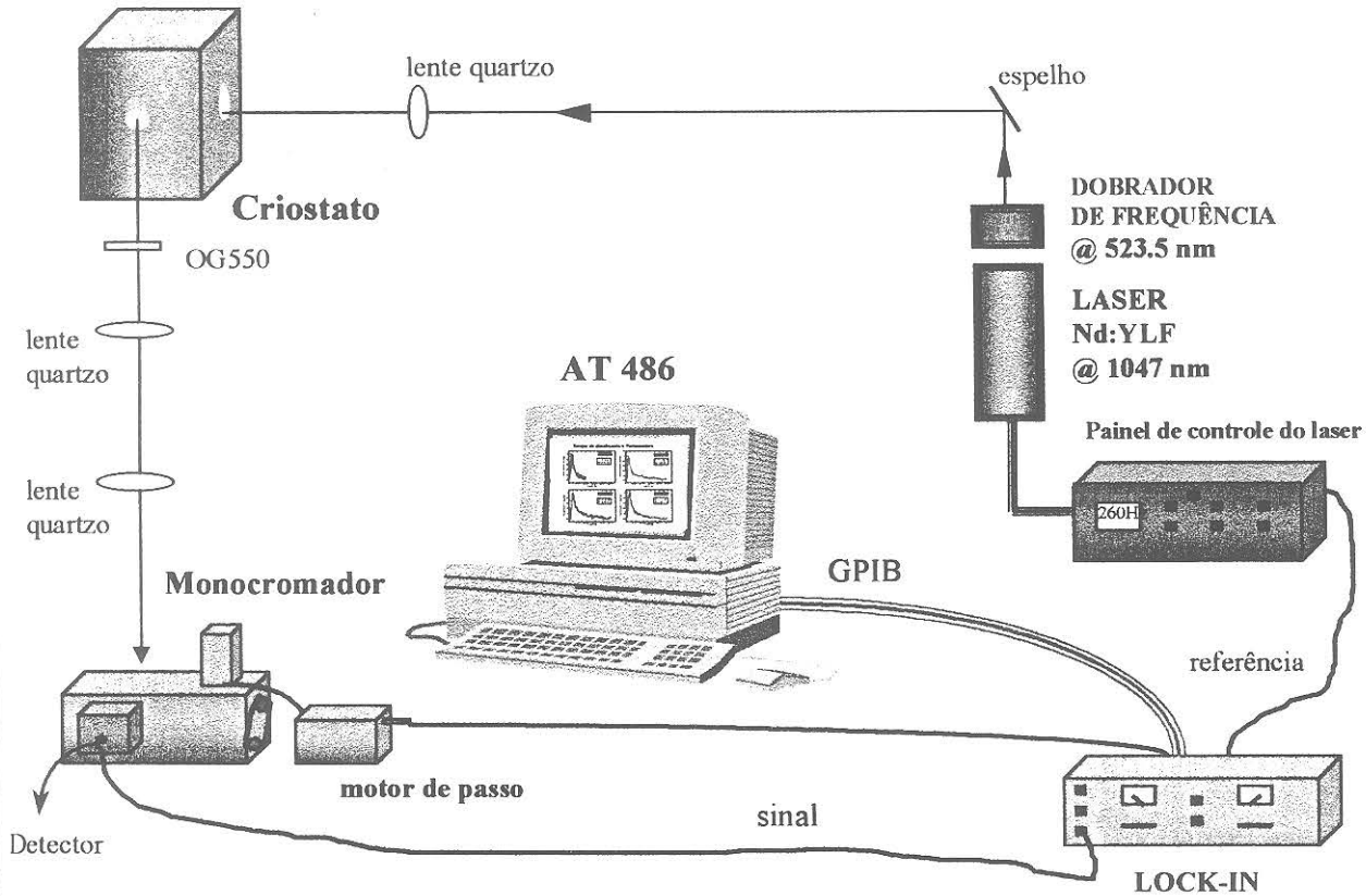
Figura 4-2: Esquema experimental utilizado para a realização das medidas dos espectros de fotoluminescência.
