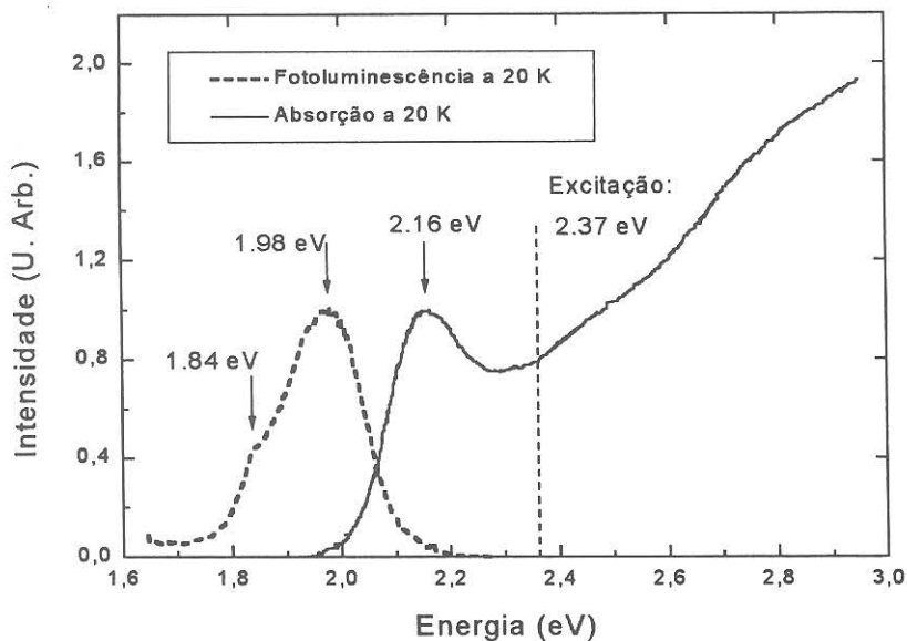
Figura 4-3: Medidas de absorção (curva cheia) e fotoluminescência (curva tracejada) da amostra VDS39-60h: 540min, a 20K. Os espectros foram normalizados para efeito de comparação. A linha tracejada na vertical representa a posição, em energia, do laser de bombeio.
