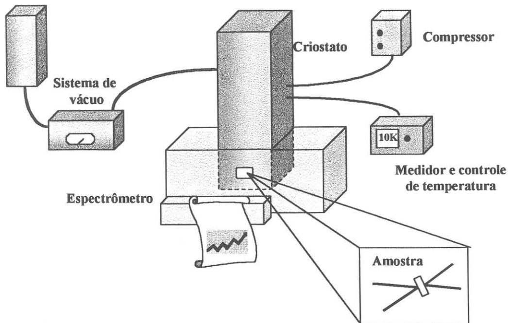
Figura 3-1: Montagem experimental usada para as medidas de absorção.
