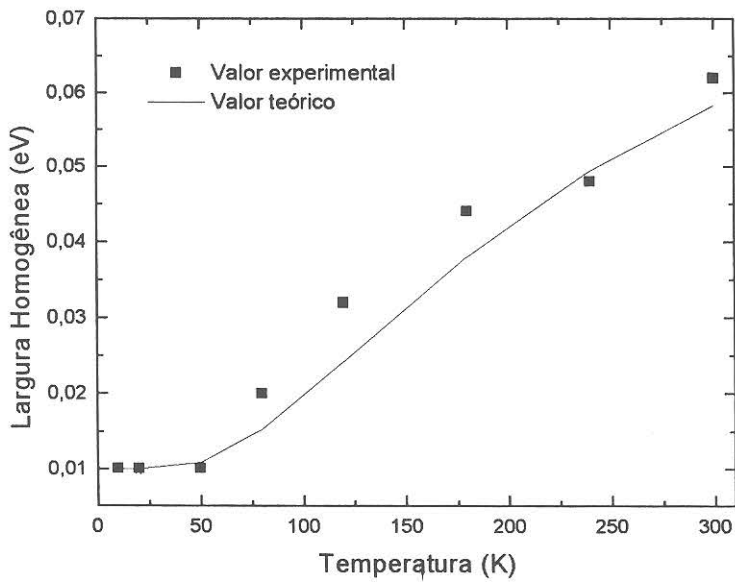
Figura 3-6: Comportamento do alargamento homogêneo com a temperatura, para a amostra VDS39-270h: 420min
