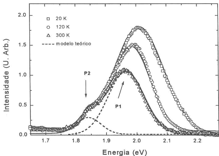
Figura 4-4: Resultados experimentais dos espectros de fotoluminescência da amostra VDS39-270h: 300min, medidos às temperaturas de 20 K (quadrados), 120 K (círculos) e 300 K (triângulos). As linhas tracejadas representam as duas Gaussianas que, somadas (curvas cheias), ajustam os dados experimentais. Os picos P1 e P2 estão indicados pelas setas.
