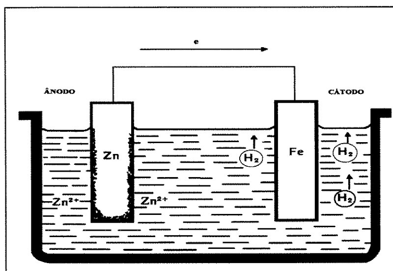
FIG. 3.10- Pilha de eletrodos metálicos
