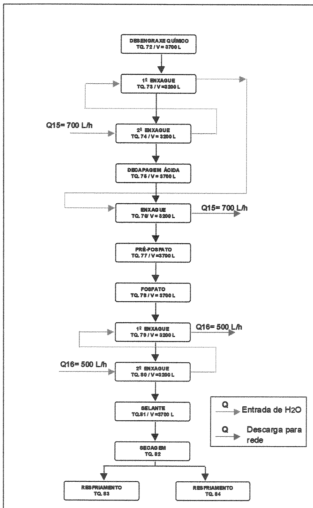
FIG. 4.4- Fluxograma do processo da fosfatização (ala 5) desenvolvido na indústria de Freios Varga
