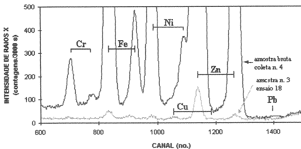
FIG.5.1 Espectros de raios X dos filtros das amostras bruta e da amostra 3 do ensaio 18, obtida com a fonte de Pu-238, em um tempo de excitação/detecção de 3000s
