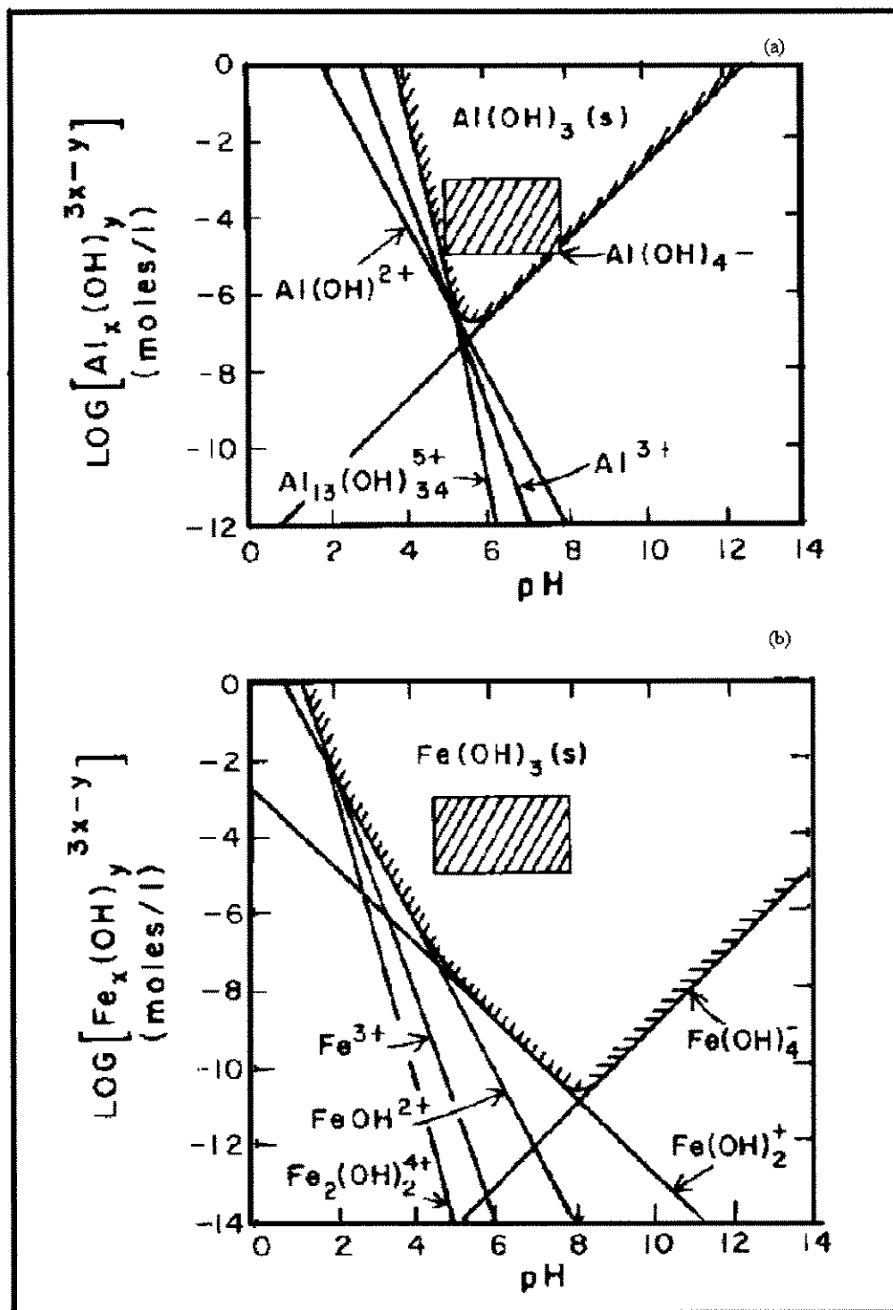
FIG. 3.5- Diagramas de solubilidade do alumínio e do ferro III em função do pH
