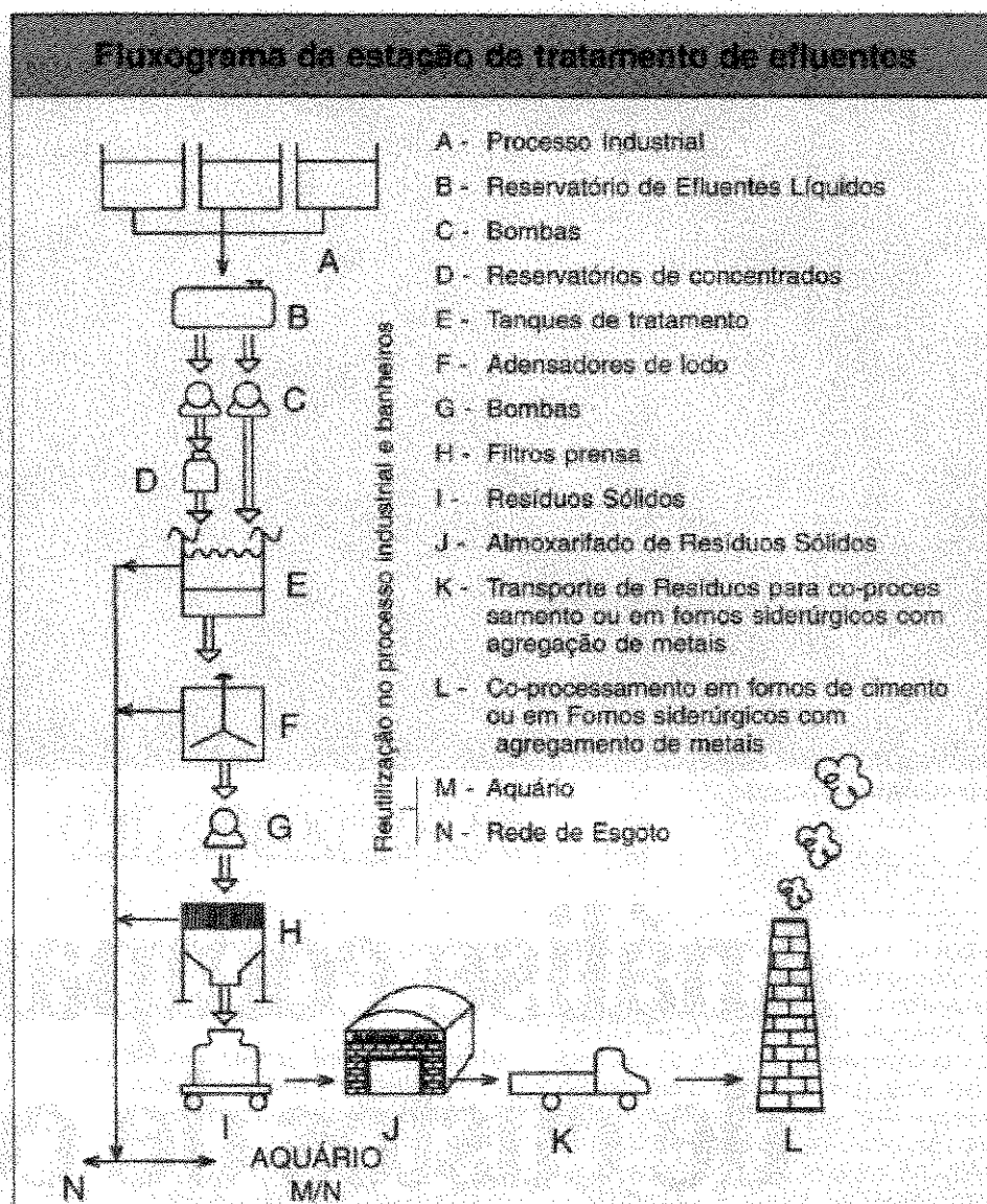
FIGURA 3.11- Fluxograma da estação de tratamento de efluentes da B.S. Continental
