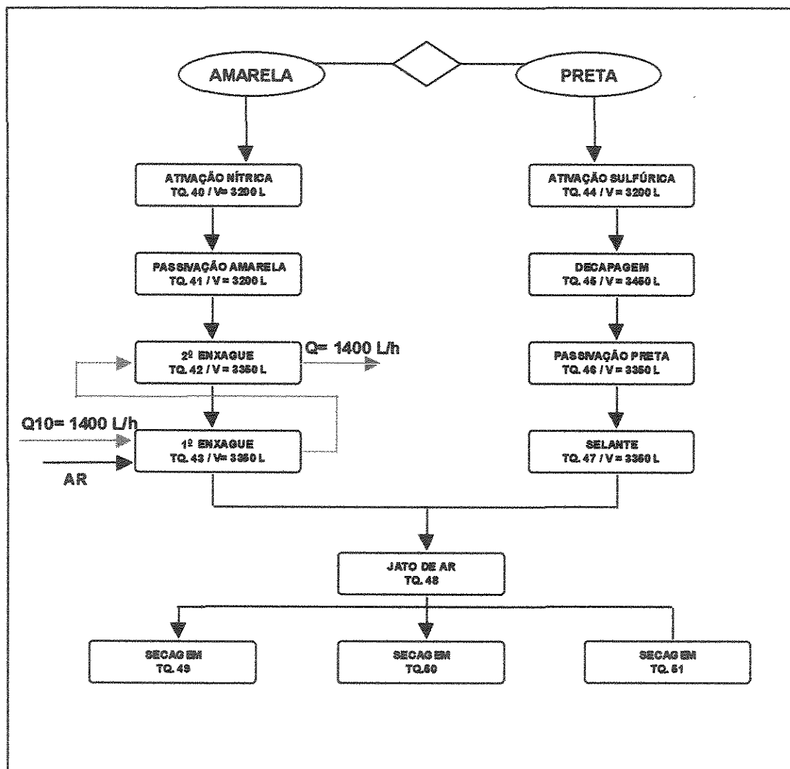
CONT. FIG. 4.2- Fluxograma do processo de zincagem ácida- Zinco-Ácido (ala 4) desenvolvido na indústria de Freios Varga
