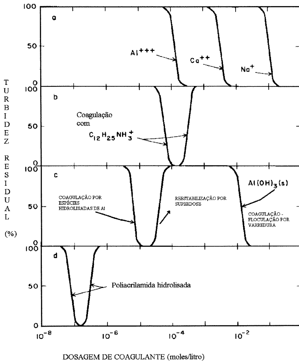
FIG. 3.4- Curvas esquemáticas de coagulação segundo os diversos mecanismos de desestabilização
