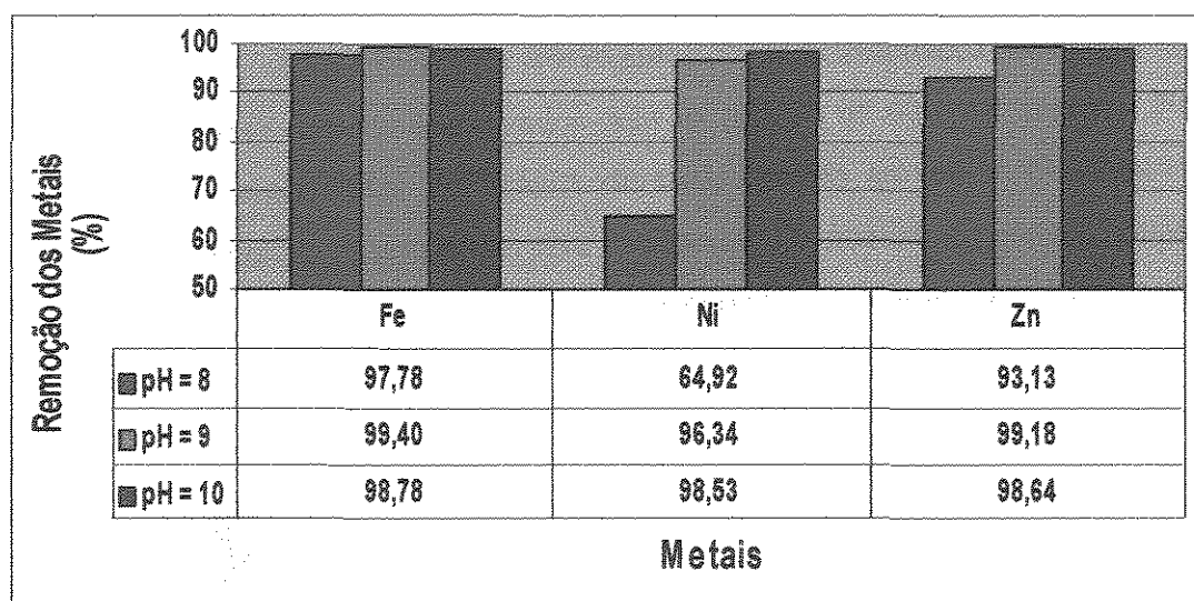
FIG. 6.3- Porcentagem de remoção dos metais, em função do pH, do ensaio 4 para o tempo de sedimentação de 90 minutos.
