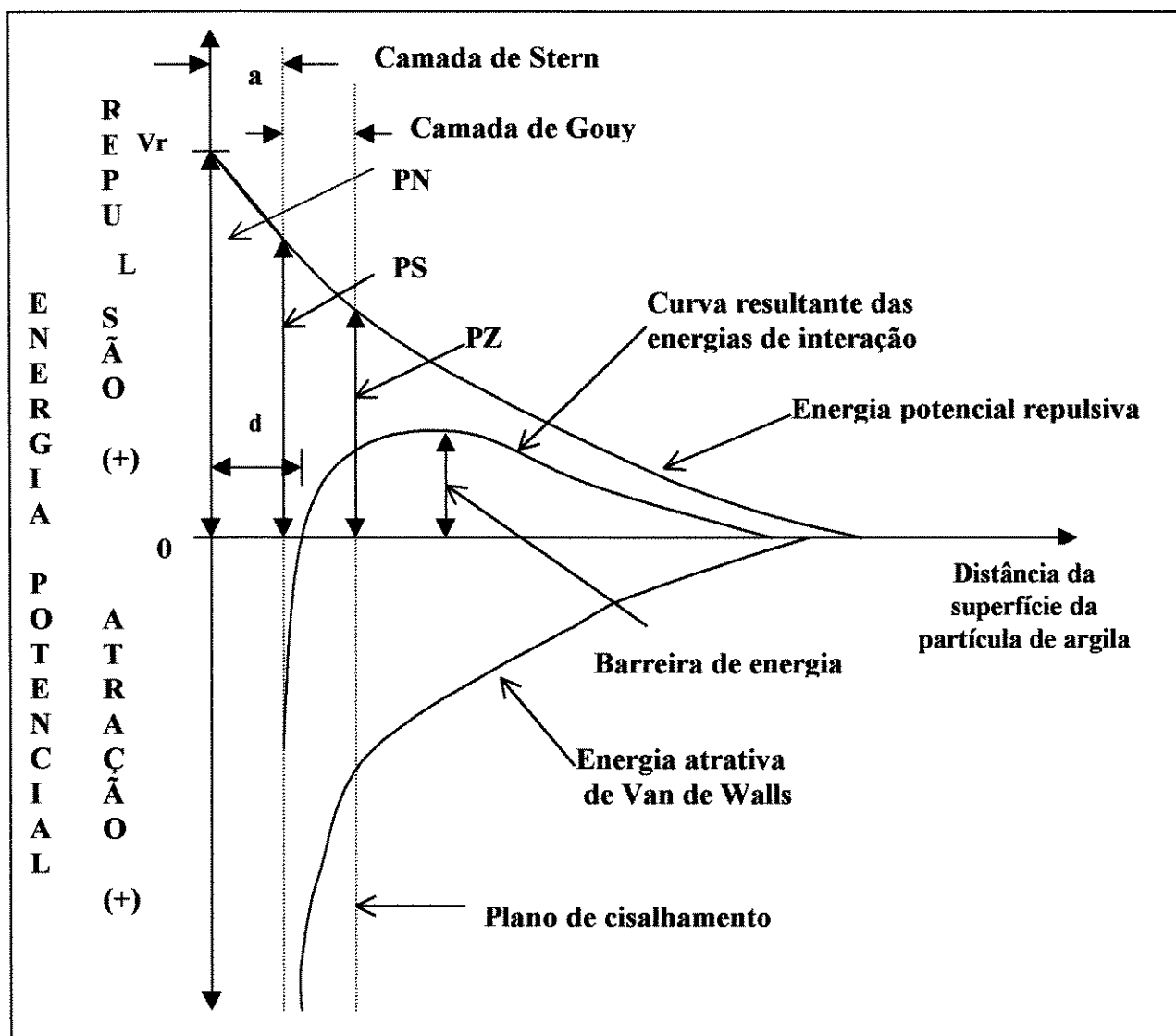
FIG. 3.2 - Energia potencial de interação entre as partículas coloidais.
