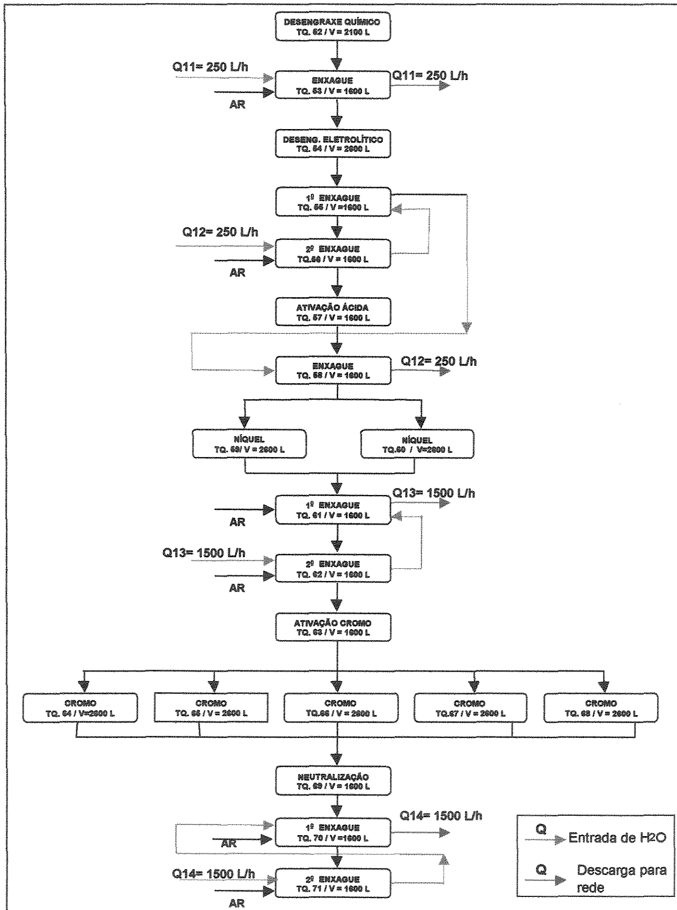
FIG. 4.3- Fluxograma do processo industrial do Níquel-Cromo (ala 4) desenvolvido na indústria de Freios Varga
