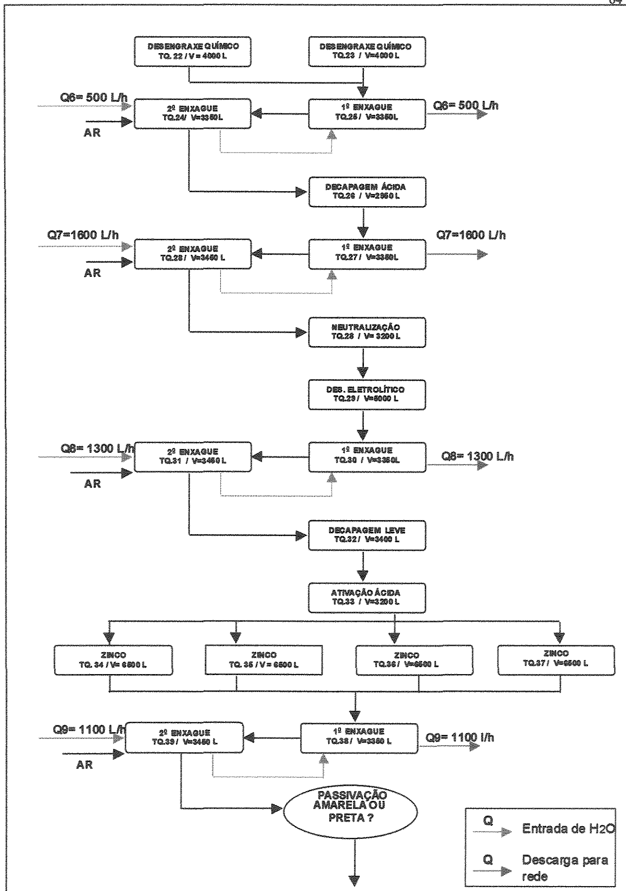
FIG. 4.2- Fluxograma do processo de zincagem ácida- Zinco-Ácido (ala 4) desenvolvido na indústria de Freios Varga
