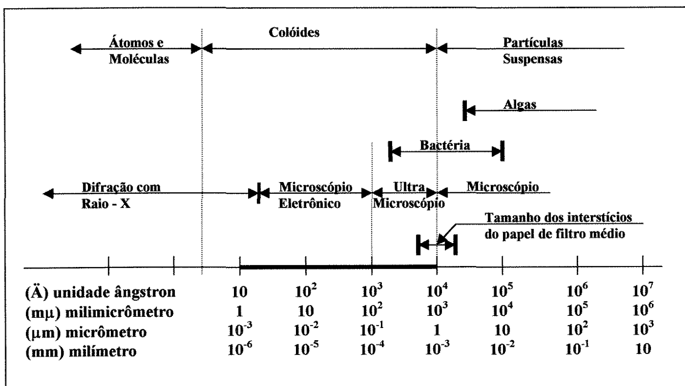
FIG. 3.1- Distribuição dos tamanhos das partículas nas águas.
