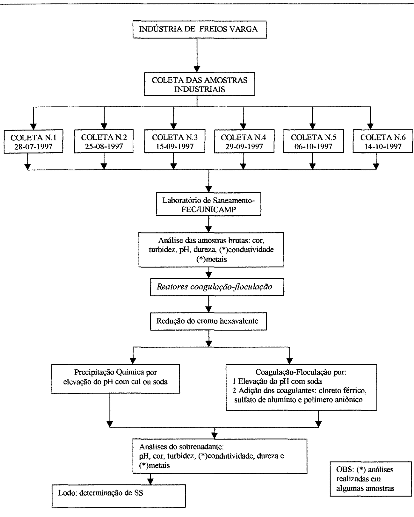
FIG. 4.5- Fluxograma da etapa de coletas das amostras brutas, análises e tratamento físico-químico do trabalho experimental.
