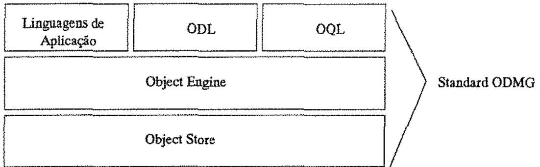
Figura 5.1: Arquitetura ODMG
