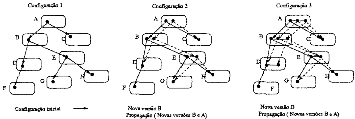
Figura 2.5: Configurações intermediárias
