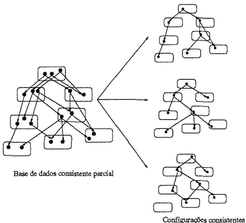
Figura 2.3: Consistência Parcial
