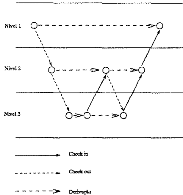
Figura 2.6: Operações de Check-in / Check-out
