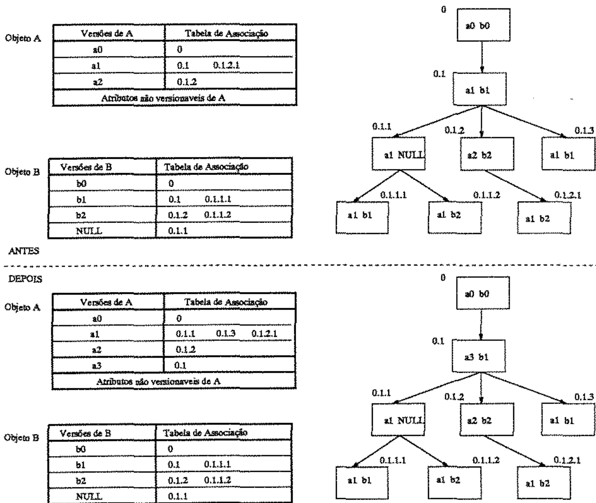
Figura 4.5: Modificação do estado de uma versão lógica
