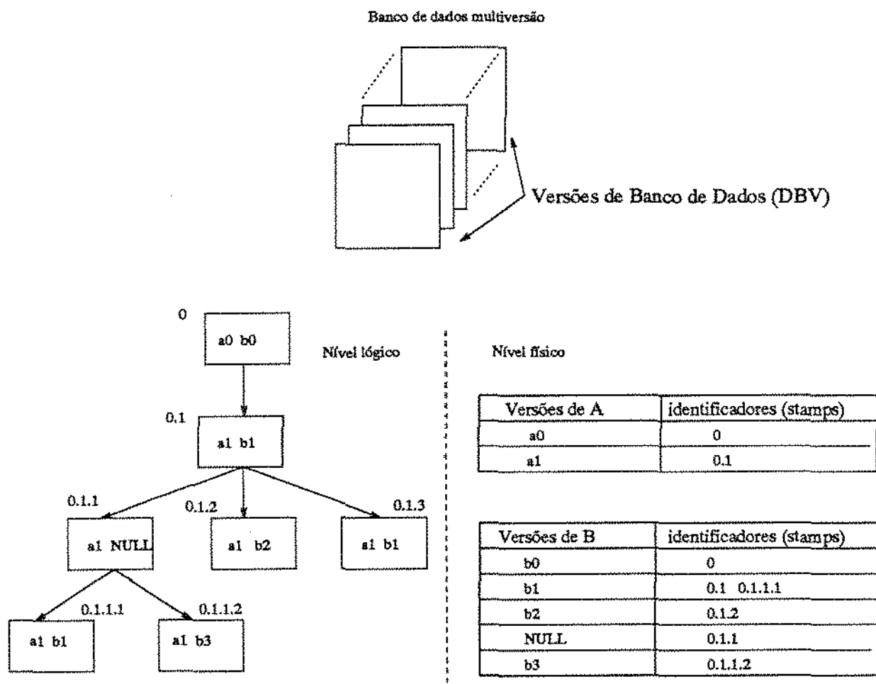
Figura 4.2: O Mecanismo DBV
