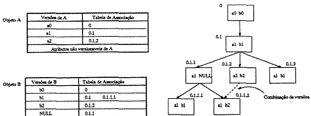
Figura 4.3: Nova estrutura dos objetos
