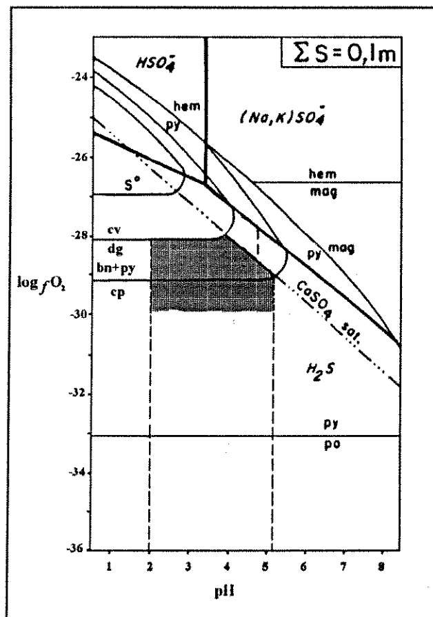
Figura 5.20. Diagrama pH vs. f\text{O}_2 mostrando a estabilidade dos sulfetos de Cu e Fe a 350^\circ\text{C} e a_{\text{H}_2\text{S}}=10^1 (ou S total=0,1 molal). A região preenchida define a estabilidade das assembléias \text{bn}+\text{dg} ( \text{cc} ) e \text{cp} presentes no depósito de Salobo. Adaptado de Haynes e Schrijver (1989).
