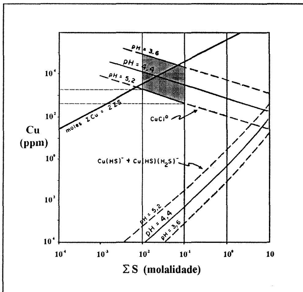
Figura 5.21. Concentrações de complexos de Cu em soluções em equilíbrio com py+cp+bn em função do pH e molalidade total de S. T=350^{\circ}\text{C} , a_{\text{Cl}^-}=1,0 e \gamma_{\text{H}_2\text{S}}=1,0 . As áreas preenchidas mostram as condições de pH e S total definidas para os fluidos aquosos salinos de Salobo. A linha \Sigma\text{Cu} = 2\Sigma\text{S} de solubilidade estequiométrica da calcosita representa o potencial máximo de precipitação deste mineral. Modificado de Crerar e Barnes (1976).
