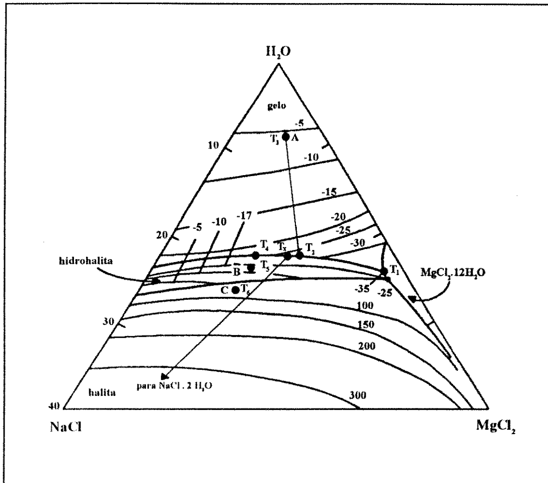
Figura 5.15. Diagrama ternário para o sistema H_2O-NaCl-MgCl_2 , mostrando as relações entre as fases sólidas e isothermas (Borisenko, 1977; Shepherd et al., 1985). Inclusão A: baixa salinidade; B: salinidade moderada; C: salinidade elevada com minerais de saturação. Tie-line Tx-composição da hidrohalita usada na determinação da composição global dos fluidos aquosos de salinidade elevada (veja explicação no texto).
