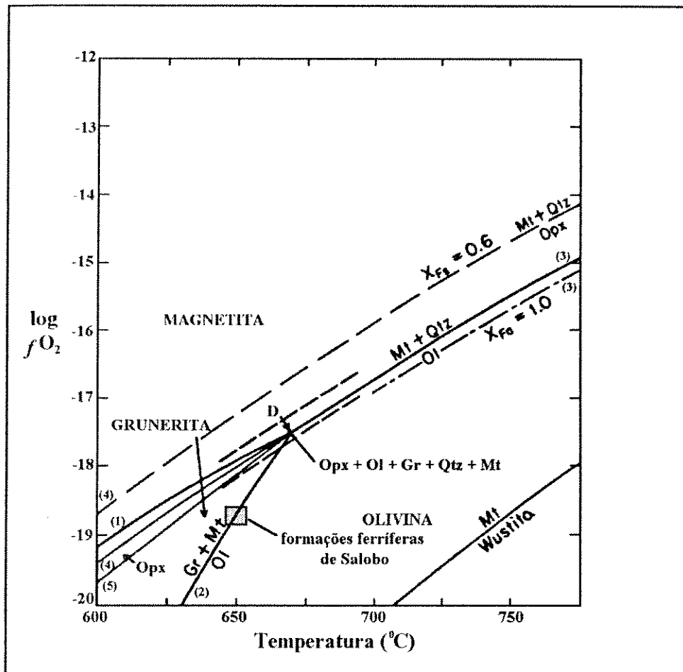
Figura 3.3. Condições de T-fO_2 para o metamorfismo progressivo das formações ferríferas de Salobo. Pressão=3 kbars. Ponto D representa a assembléia Opx-Ol-Qtz-Mt-Gru . Adaptado de Miyano e Klein (1983).
