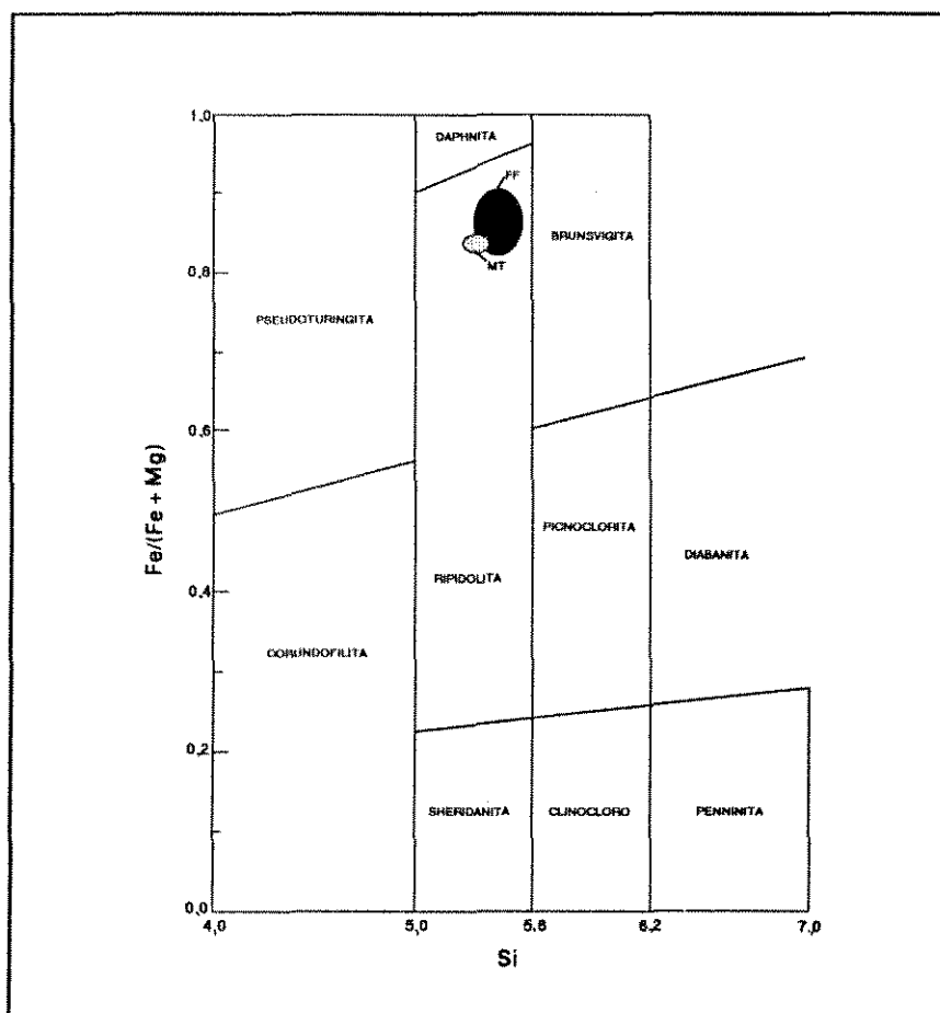
Figura 4.1. Classificação química das cloritas de Salobo demonstrada no diagrama Fe/(Fe+Mg) versus Si no sítio tetraédrico (Hey,1954). Abreviaturas: FF= formações ferríferas; MT= metagrauvascas.
