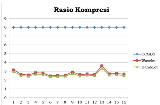
Gambar 3-3: Perbandingan nilai rasio kompresi
