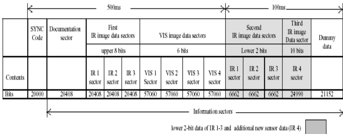
Gambar 2-1: Struktur paket data HiRID MTSAT-1R. Blok berarsir adalah data tambahan pada HiRID
