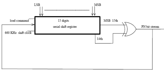
Gambar 2-5:Rangkaian pembangkit pola PN data HiRID
