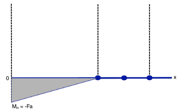
Figura 2 – Construção do diagrama do momento fletor. Durante todo o estudo, a carga de flexão foi mantida constante.
