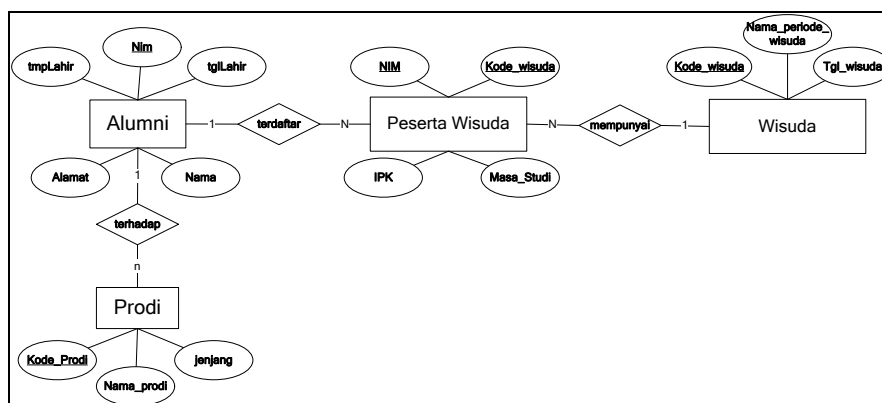
Gambar 2: ERD Pengolahan Data Alumni yang sedang berjalan
