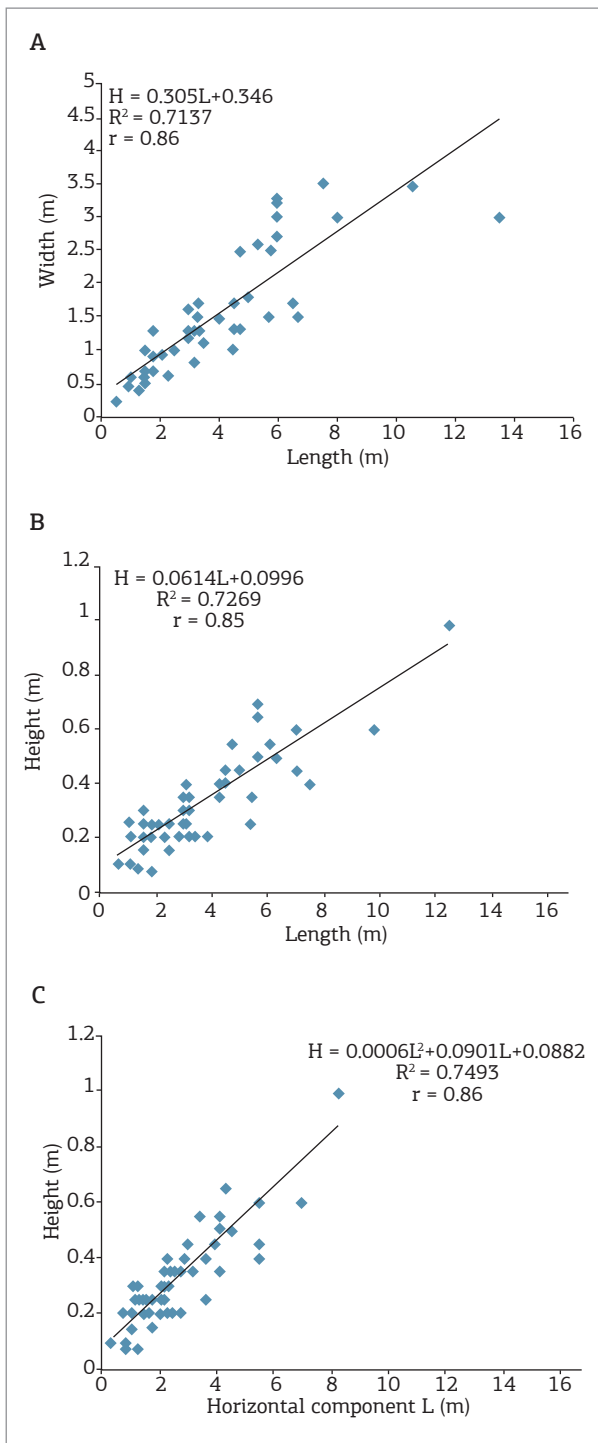
Figure 7. Morphometric parameters of the nebkhas.
