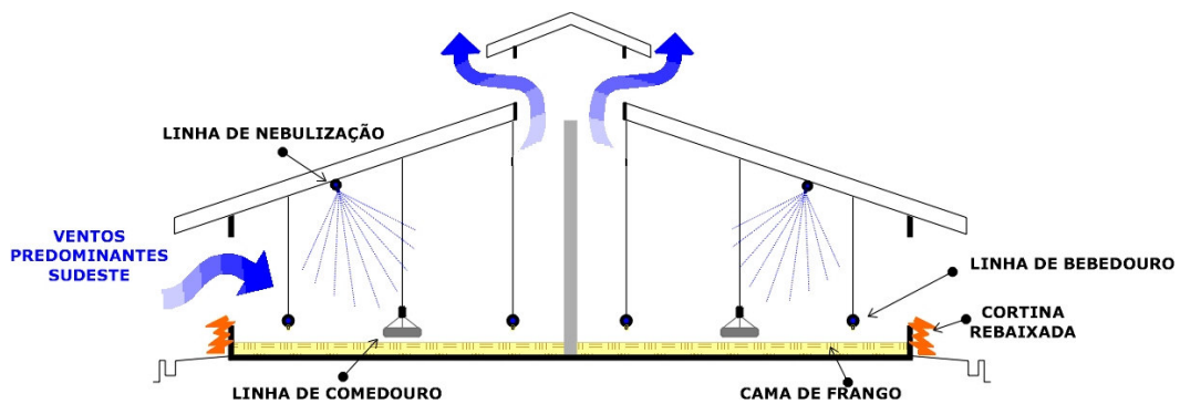
FIGURA 2. Corte transversal do galpão G_c em período de resfriamento.
