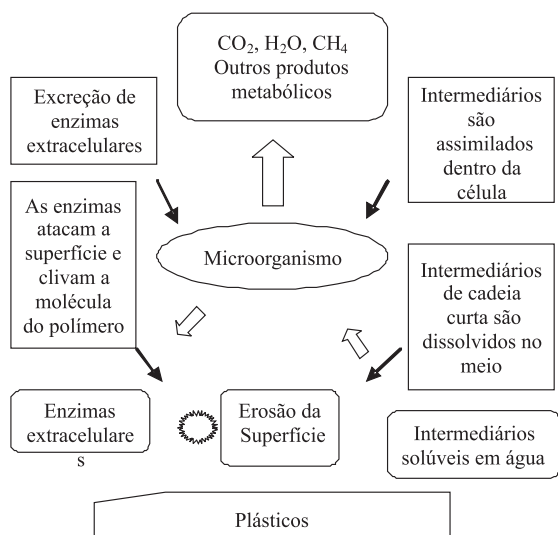
Figura 3. Mecanismo geral de degradação de plásticos catalisada por enzimas hidrolíticas
