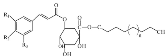
Figura 1. Estrutura química dos derivados do ácido cinâmico
