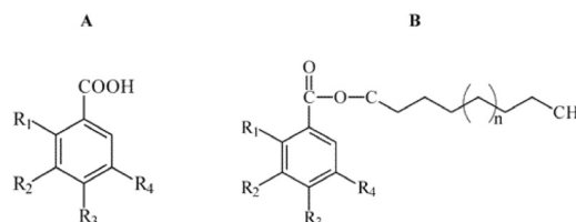
Figura 2. Estrutura química dos derivados do ácido benzóico (A) e dos ésteres alcoólicos derivados do ácido benzóico (B)
