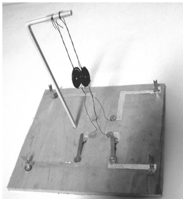
Figura 9 - Montagem final sem as pilhas.
