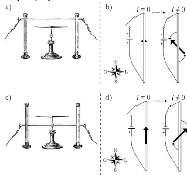
Figura 1 - Deflexão de uma bússola em relação ao meridiano magnético quando se passa uma corrente constante em um longo fio retilíneo colocado paralelamente à agulha imantada na experiência de Oersted. Se o fio está acima da agulha então o pólo da agulha que está mais próximo do terminal negativo da pilha gira para oeste, casos (a) e (b). Caso a agulha esteja sobre o fio, então o pólo da agulha que está mais próximo do terminal negativo da pilha gira para leste, casos (c) e (d).
