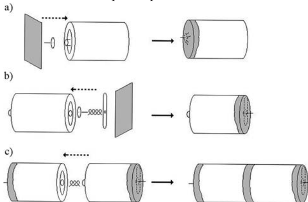
Figura 4 - Contatos para as pilhas.
