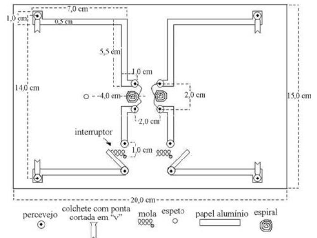
Figura 5 - Circuito elétrico e suas dimensões espaciais.
