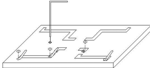
Figura 7 - Prendendo os contatos com percevejos.
