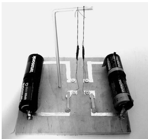
Figura 10 - Montagem final com as pilhas.
